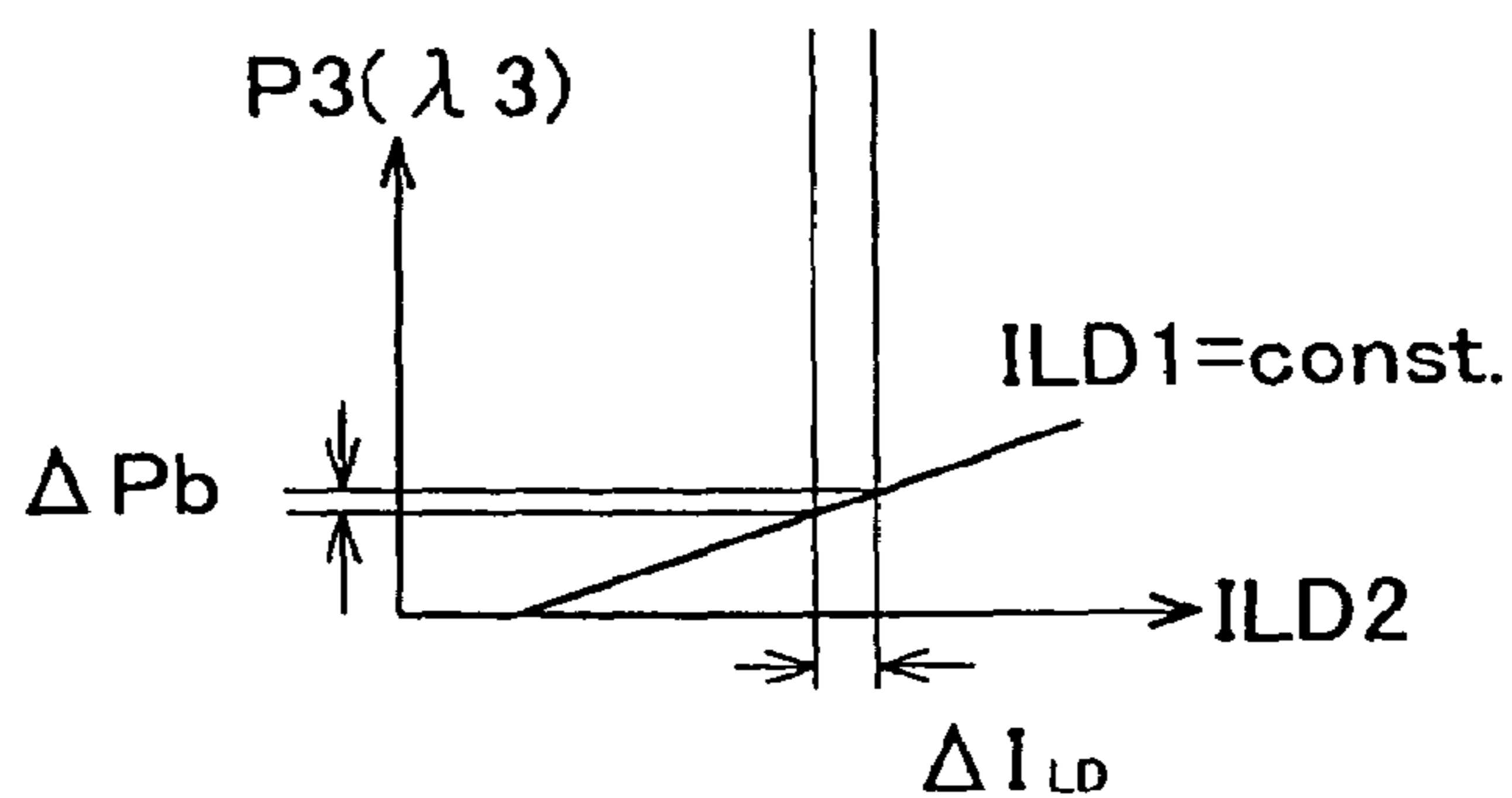
FIG.3B
