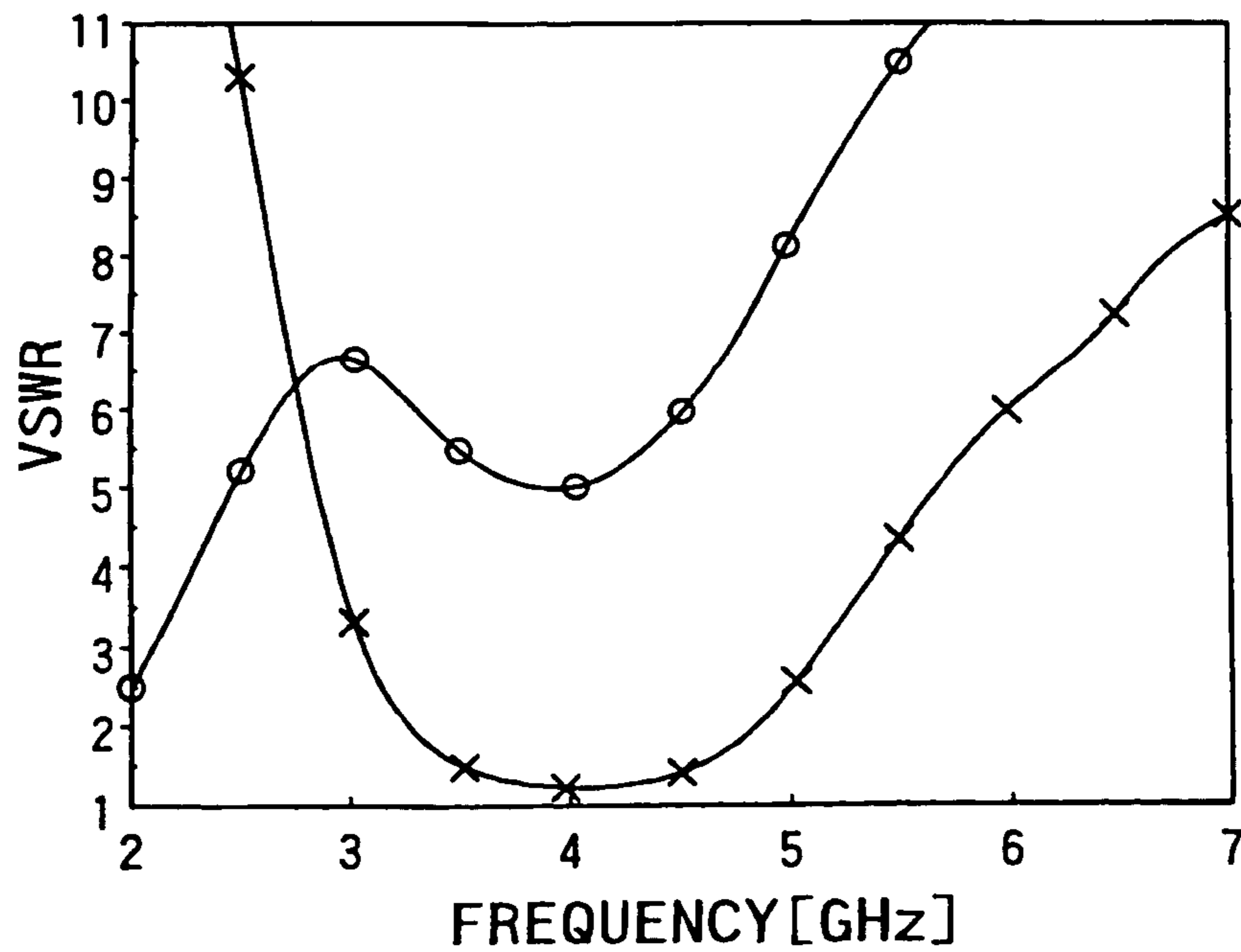
FIG. 12B
