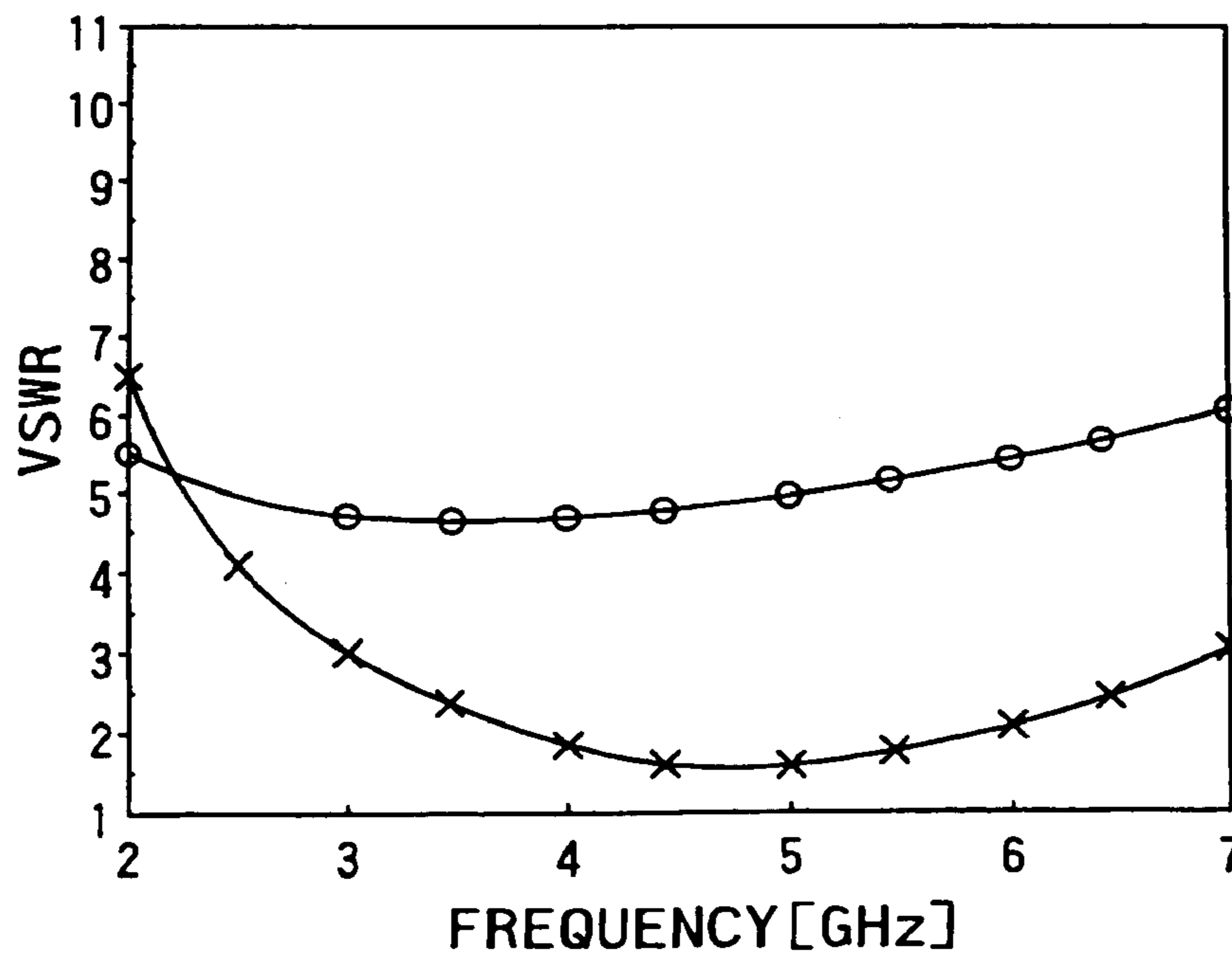
FIG. 14B
