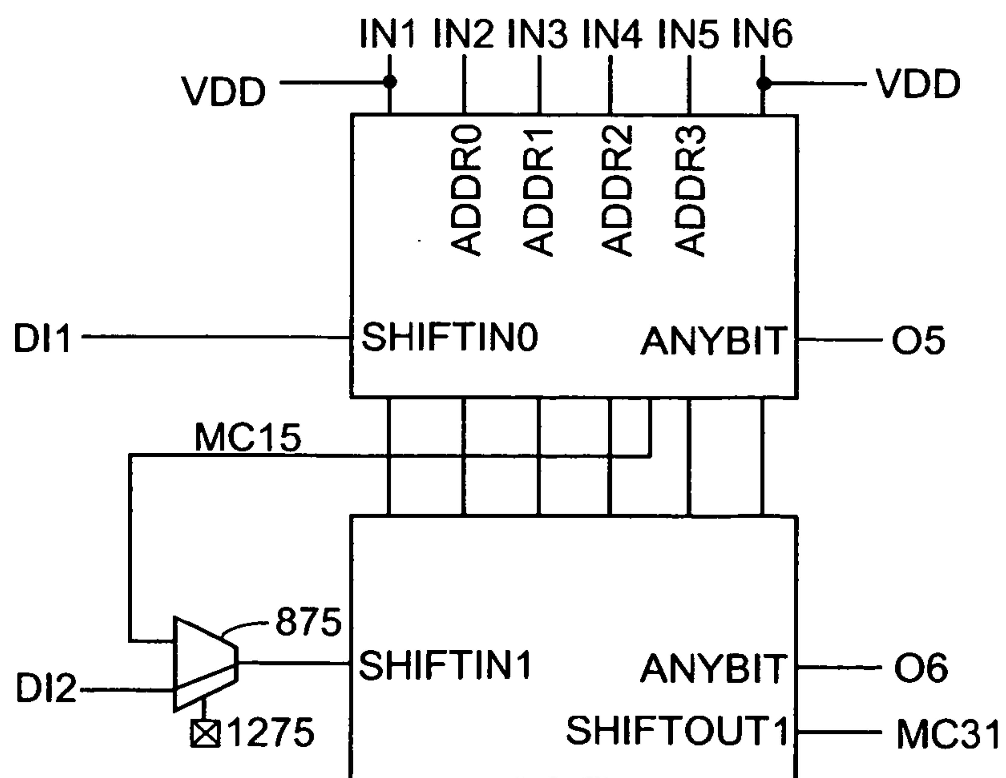
FIG. 13 (16x2 SRL)
