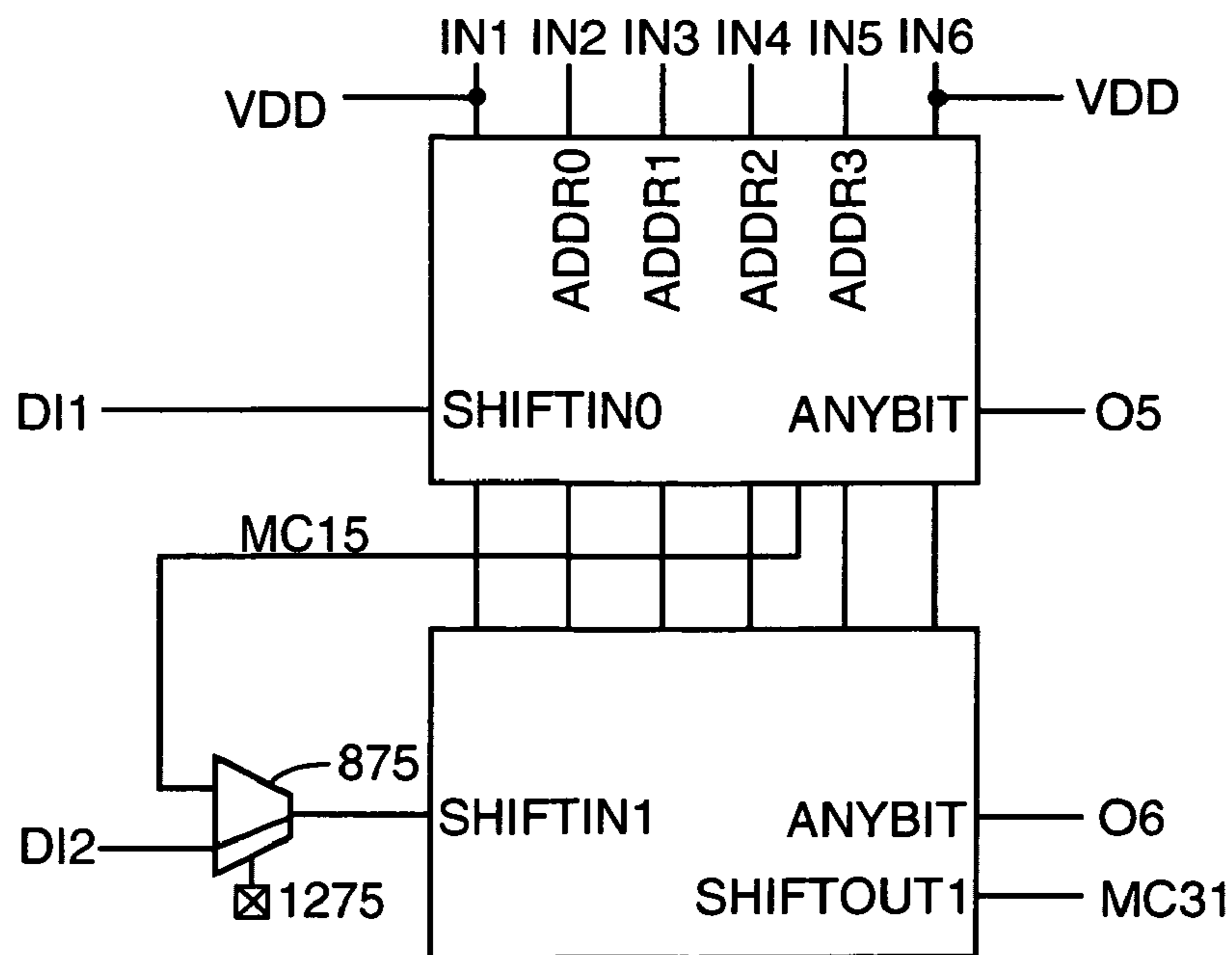
FIG. 13 (16x2 SRL)
