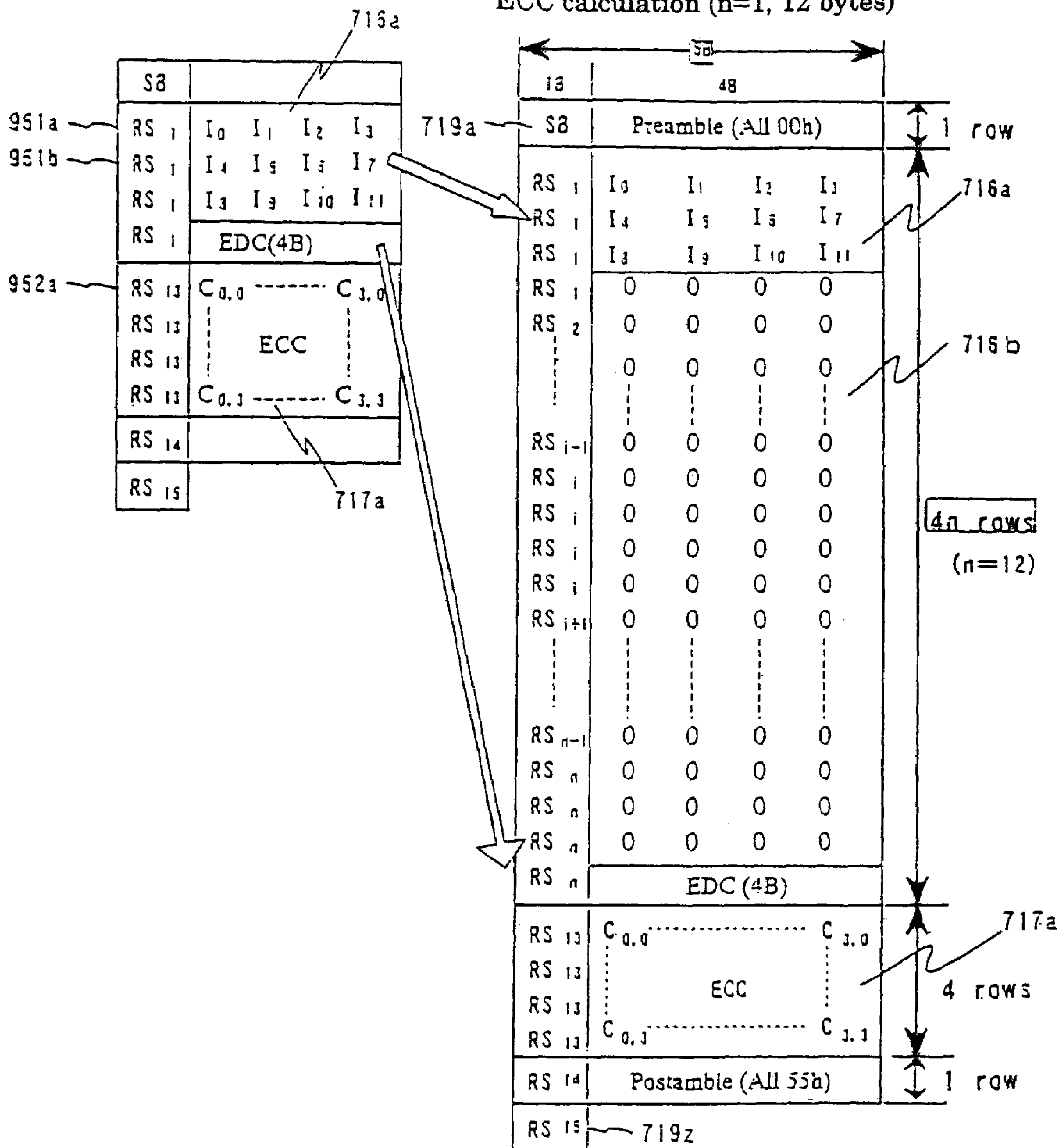
(a) data configuration (n=1, 12 bytes)
