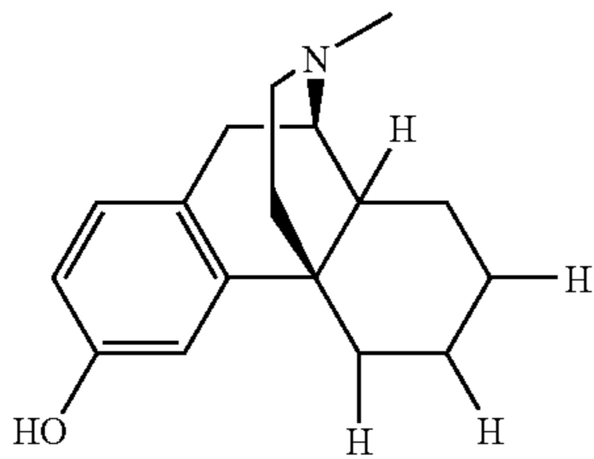
levorphanol,
