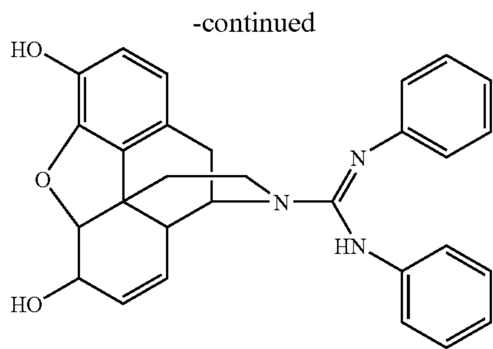
JFY-058
