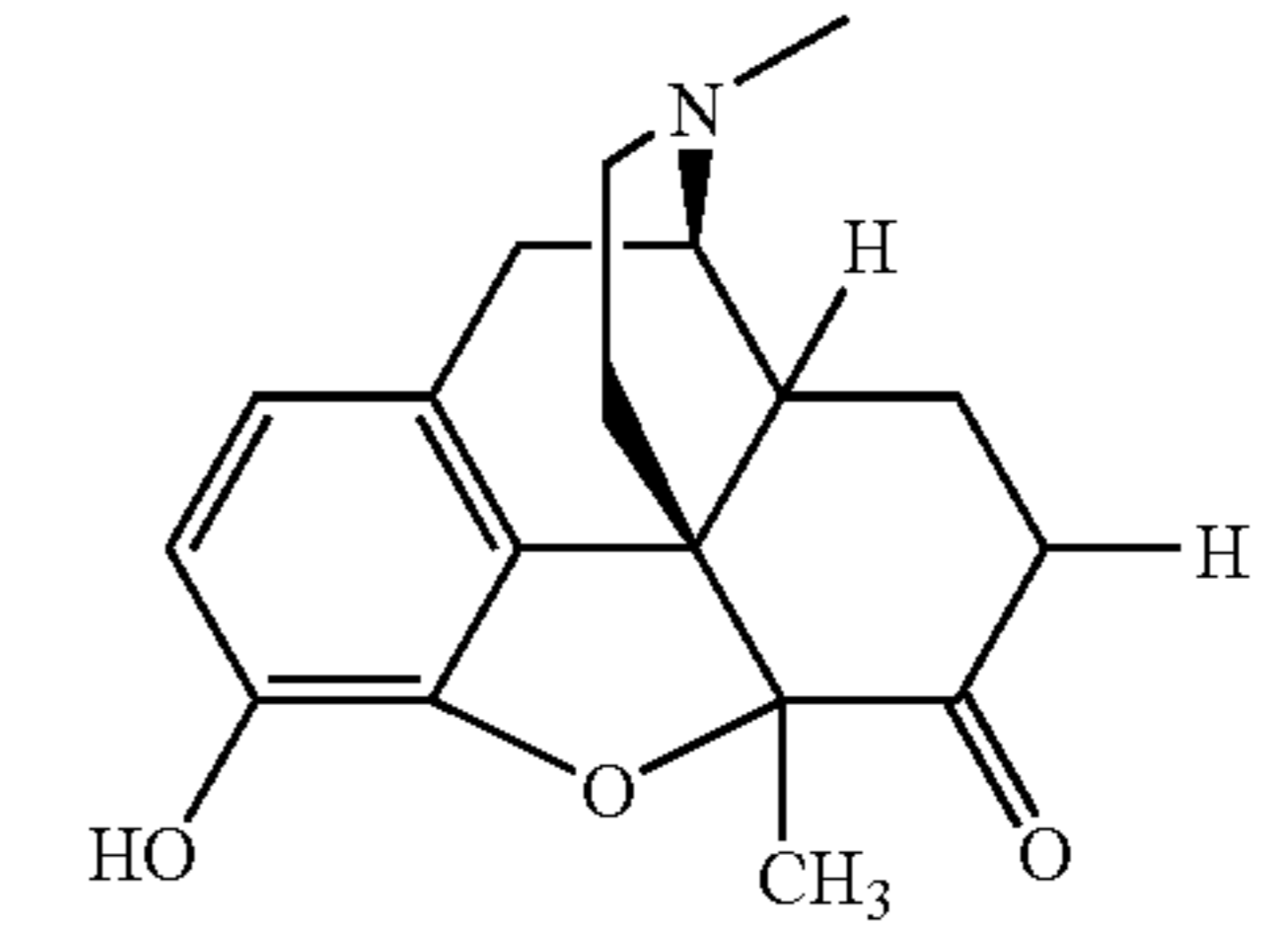
metopon,
