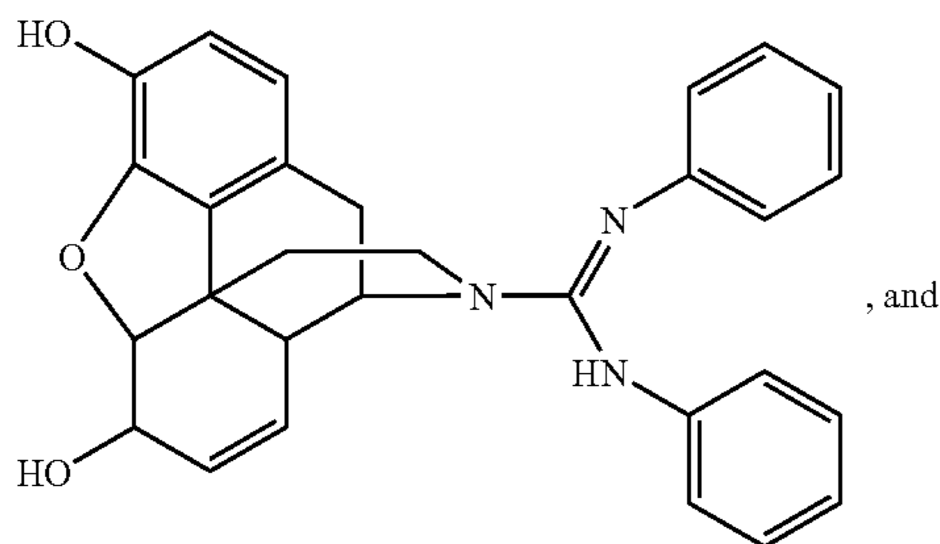
JFY-058
