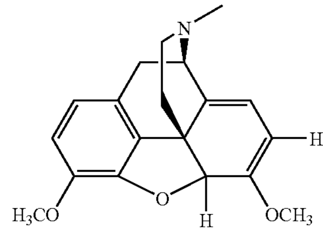
thebaine,
