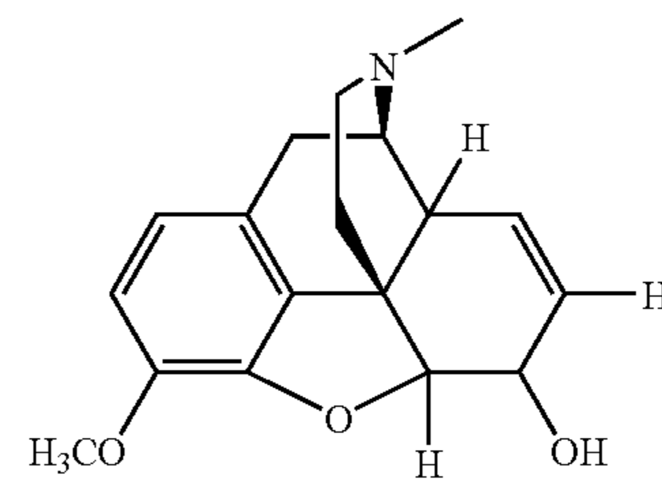
codeine,
