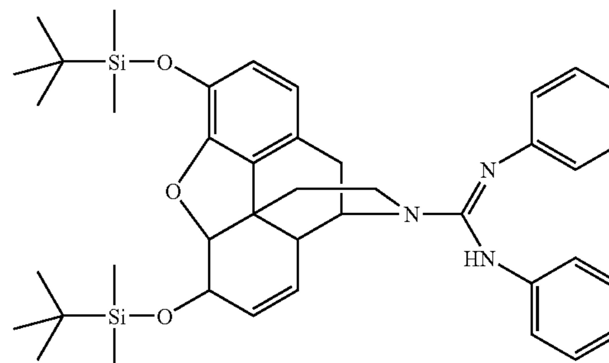
JFY-050
