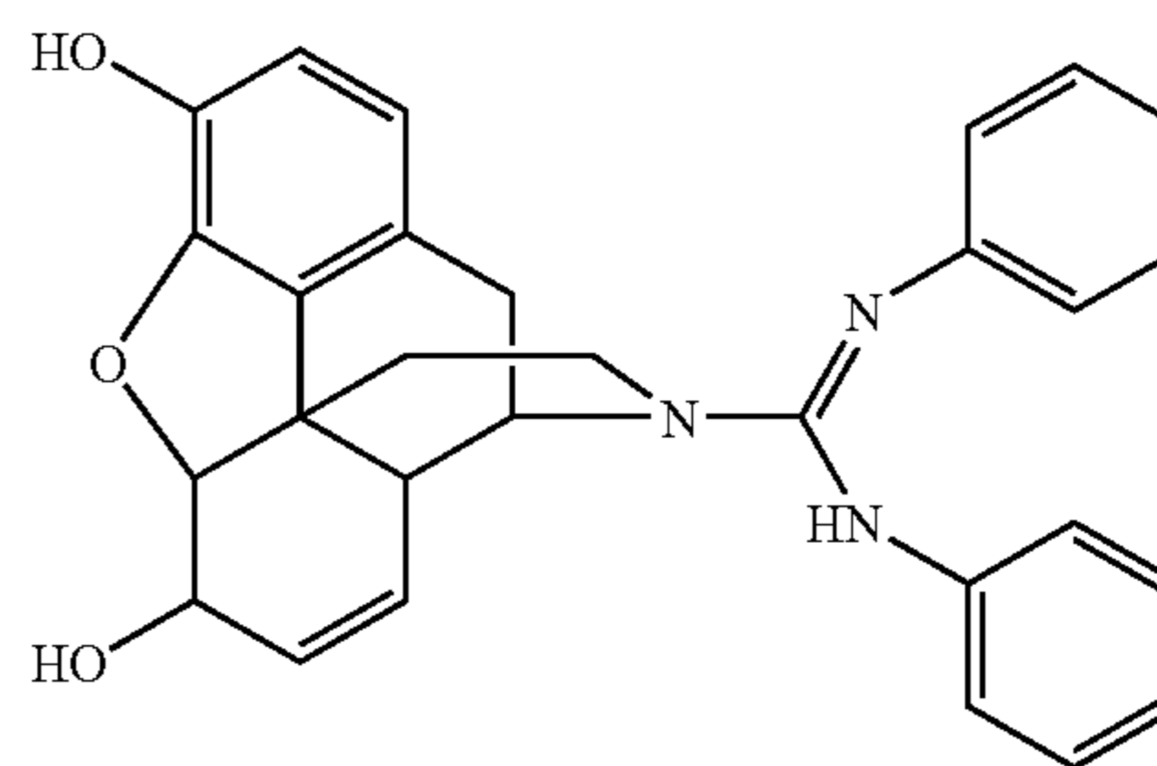
JFY-058
