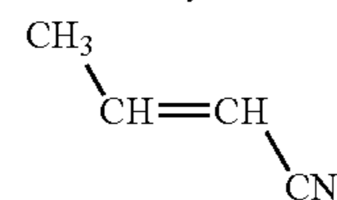
crotononitrile
