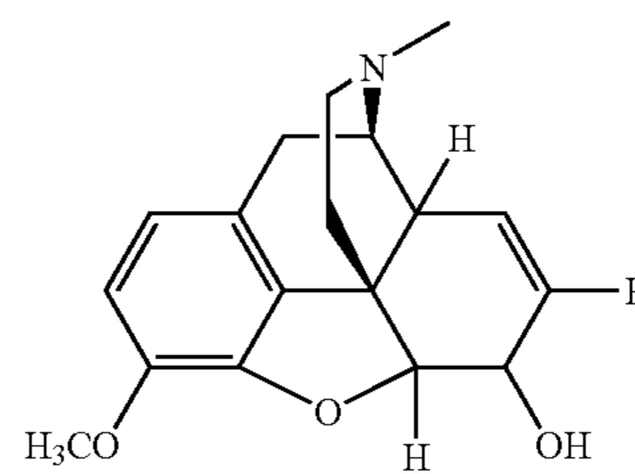
codeine,
