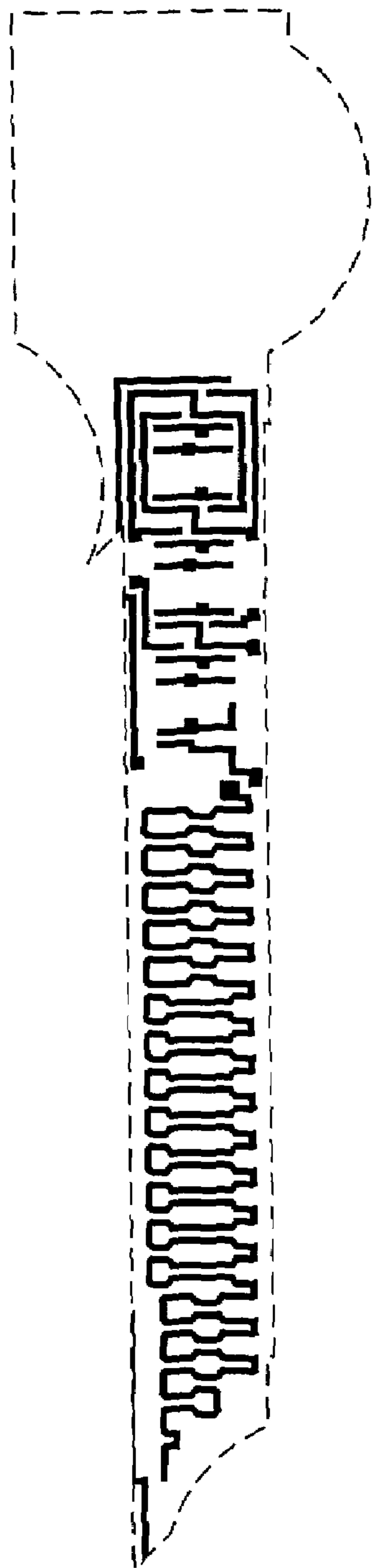
Poly mask
