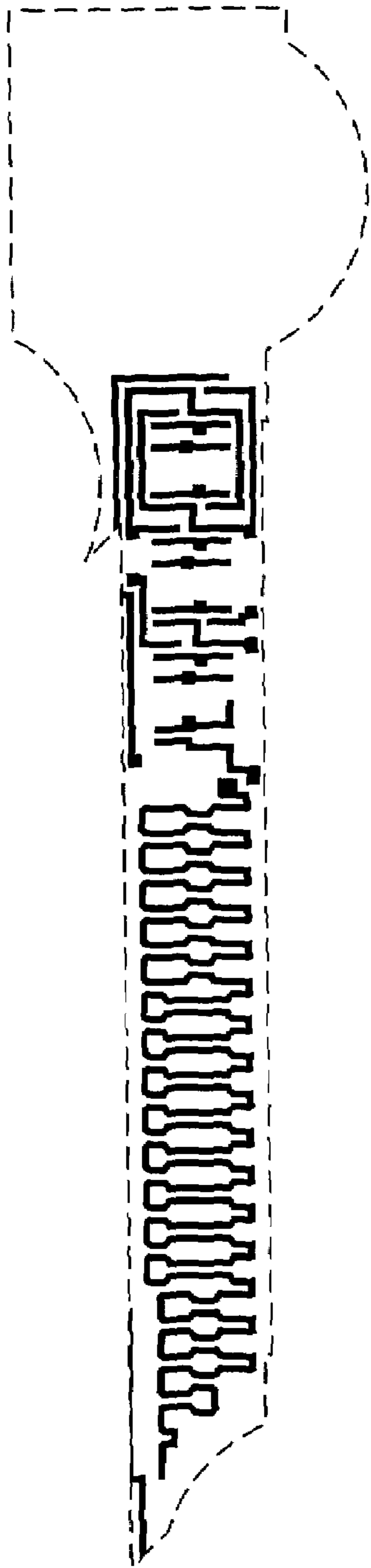
Poly mask
