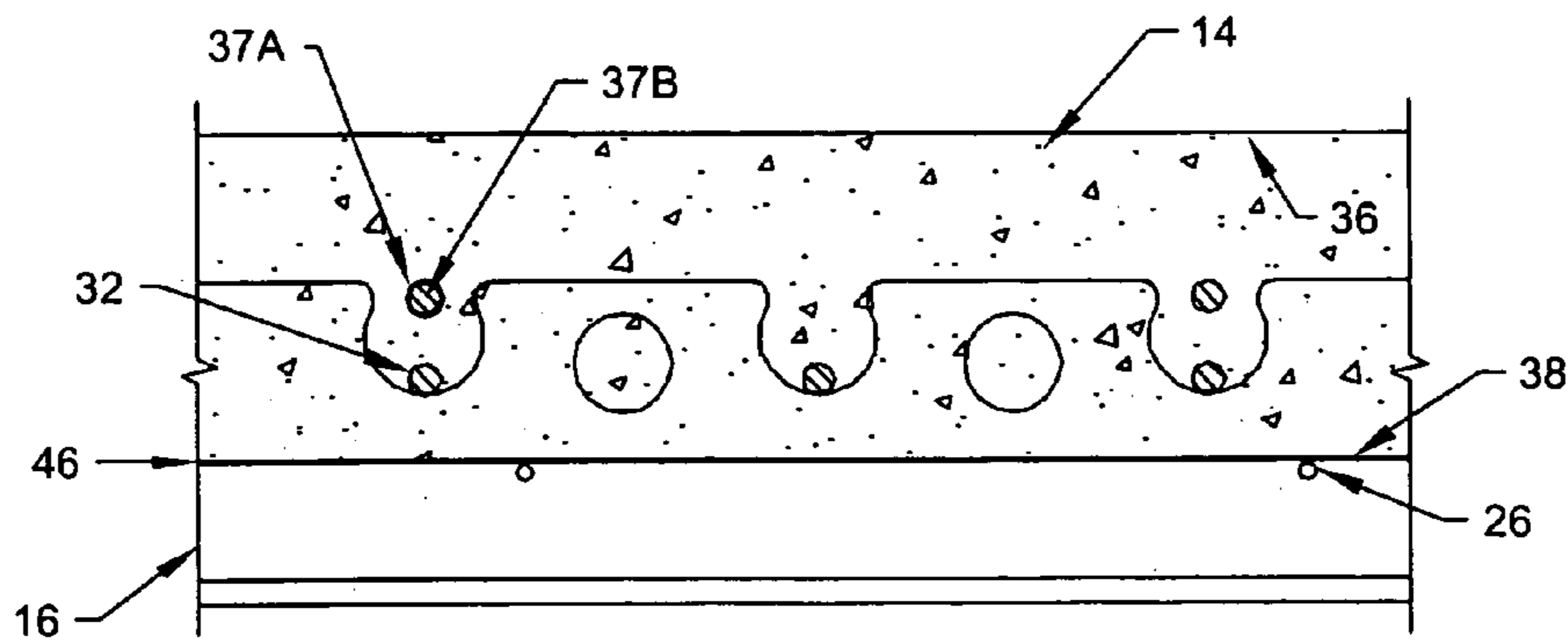
SECTION A-A
