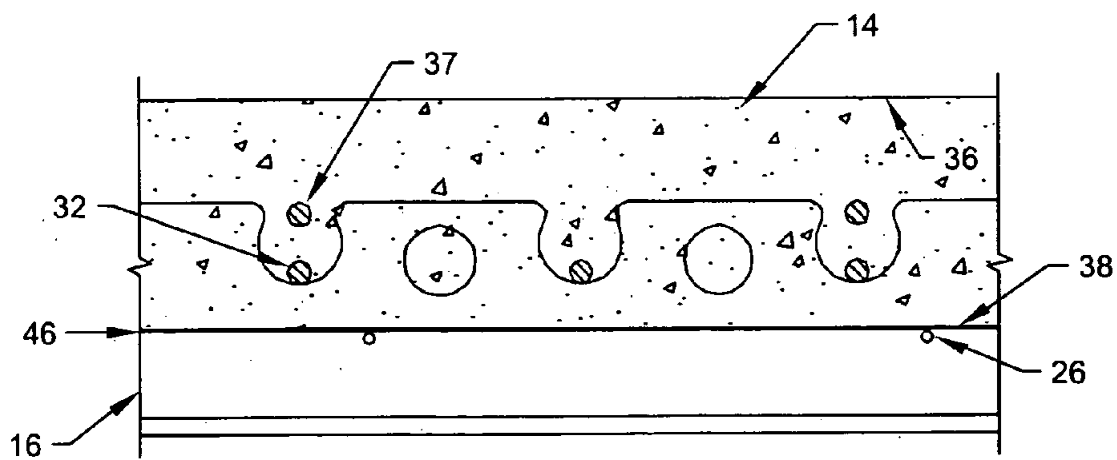
SECTION A-A
