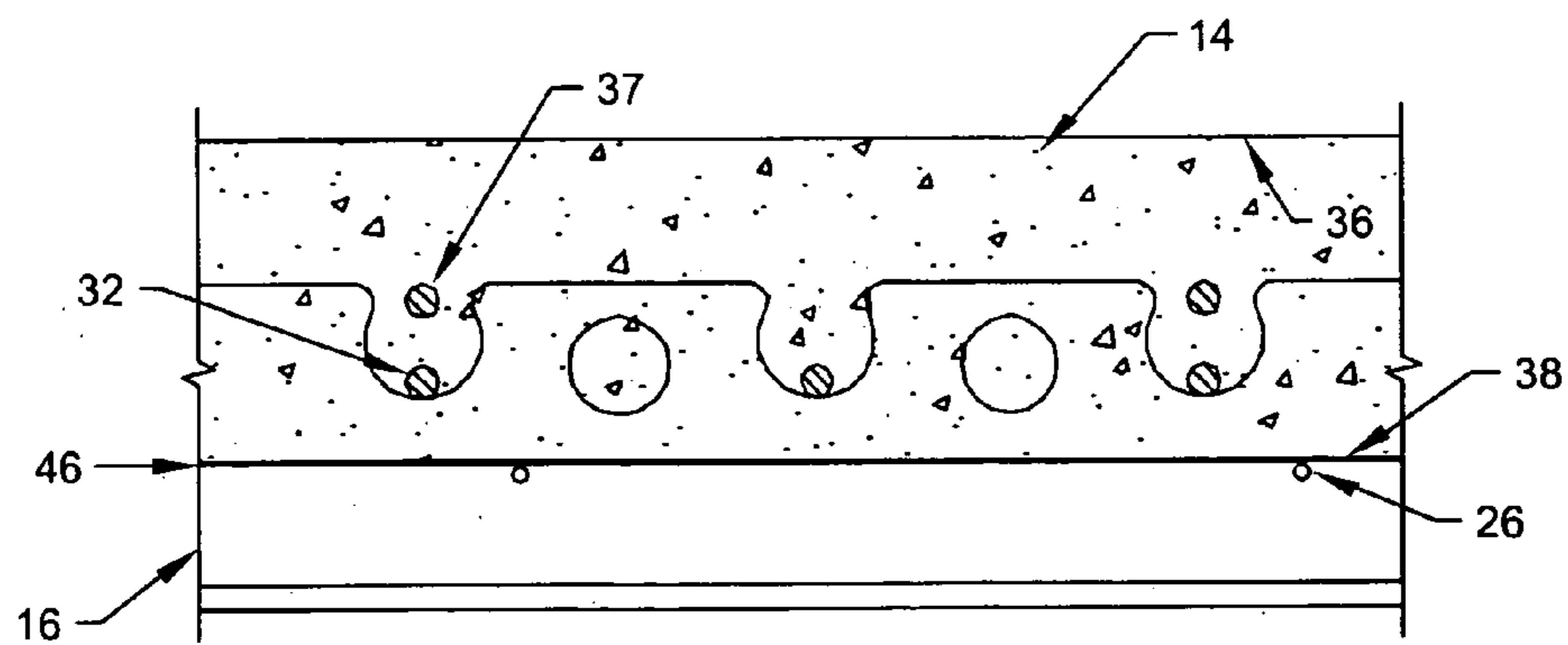
SECTION A-A
