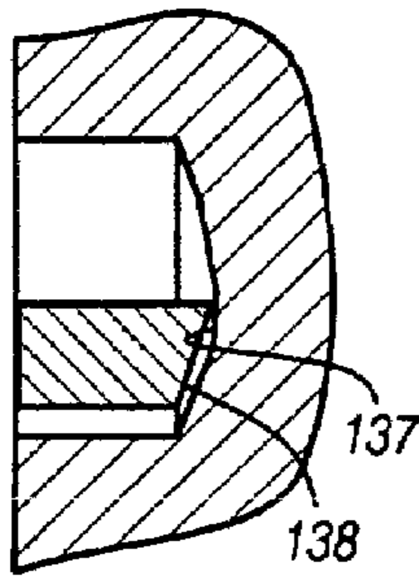
FIGURE 14 SECTION Q1-Q1 PRIOR ART
