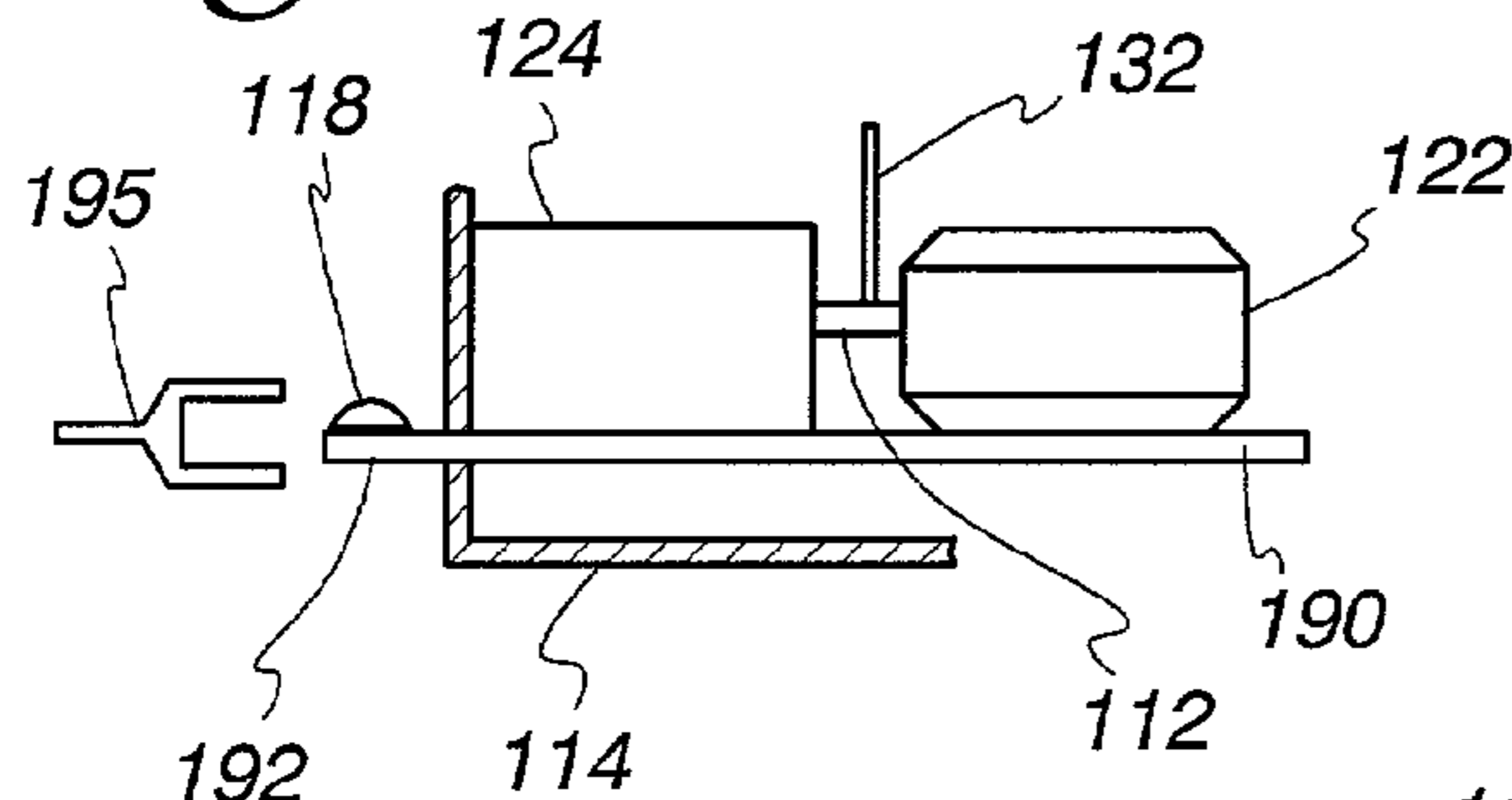
Fig. 14
