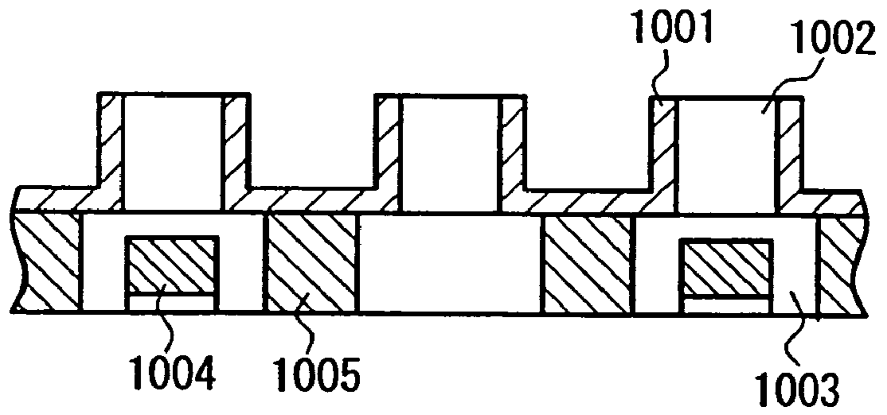
FIG. 10A
