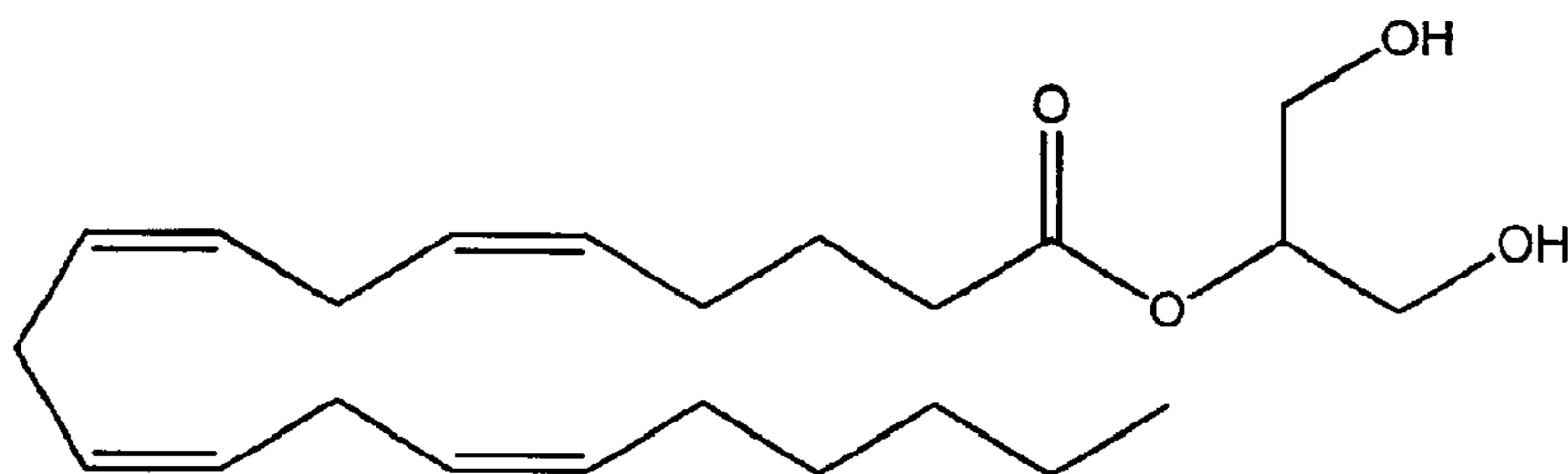
2-ARACHIDONYLGLYCEROL (2-AG)
