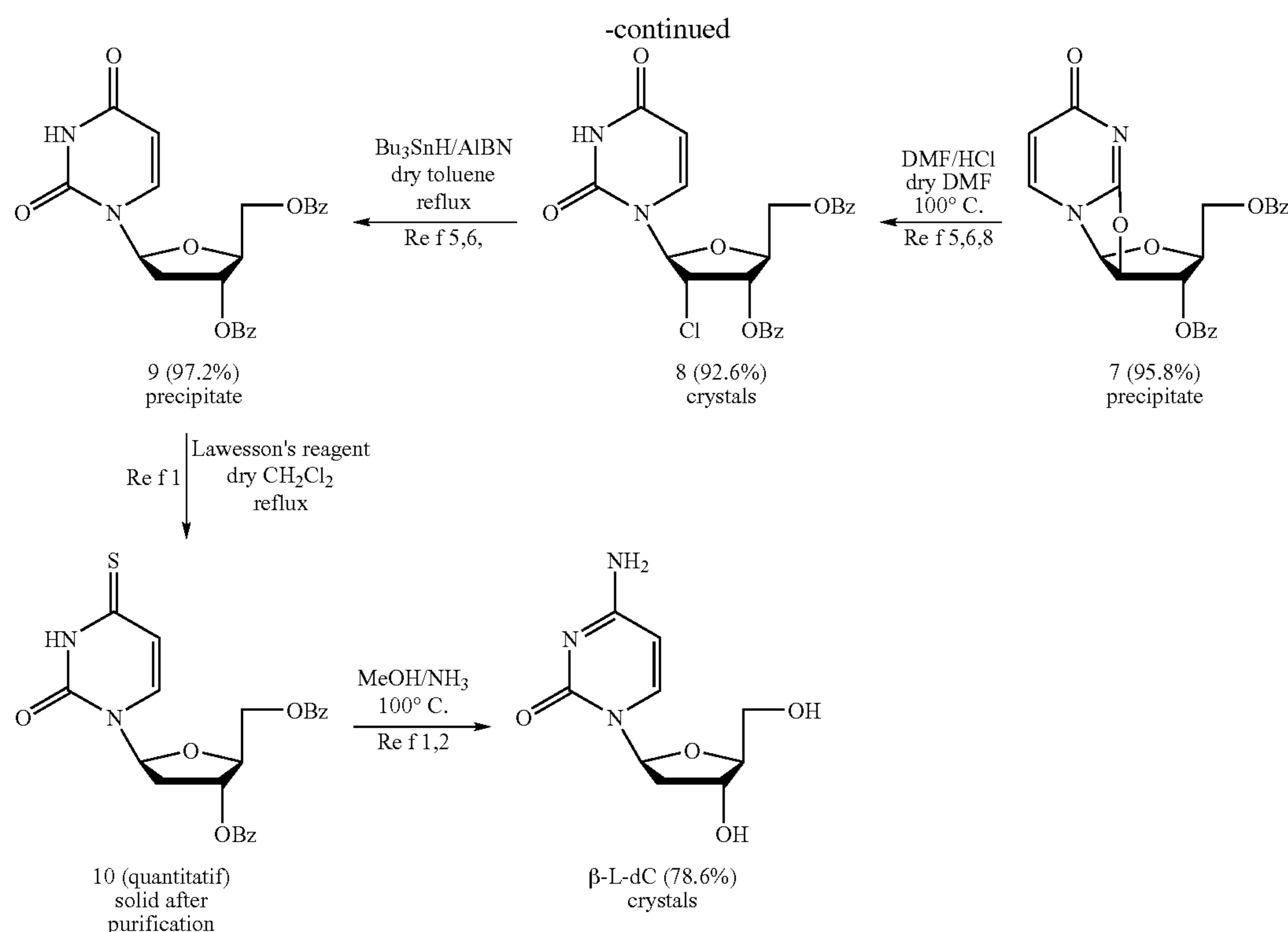
2-Amino- \beta -L-arabinofurano-[1',2':4,5]-oxazoline (5)
