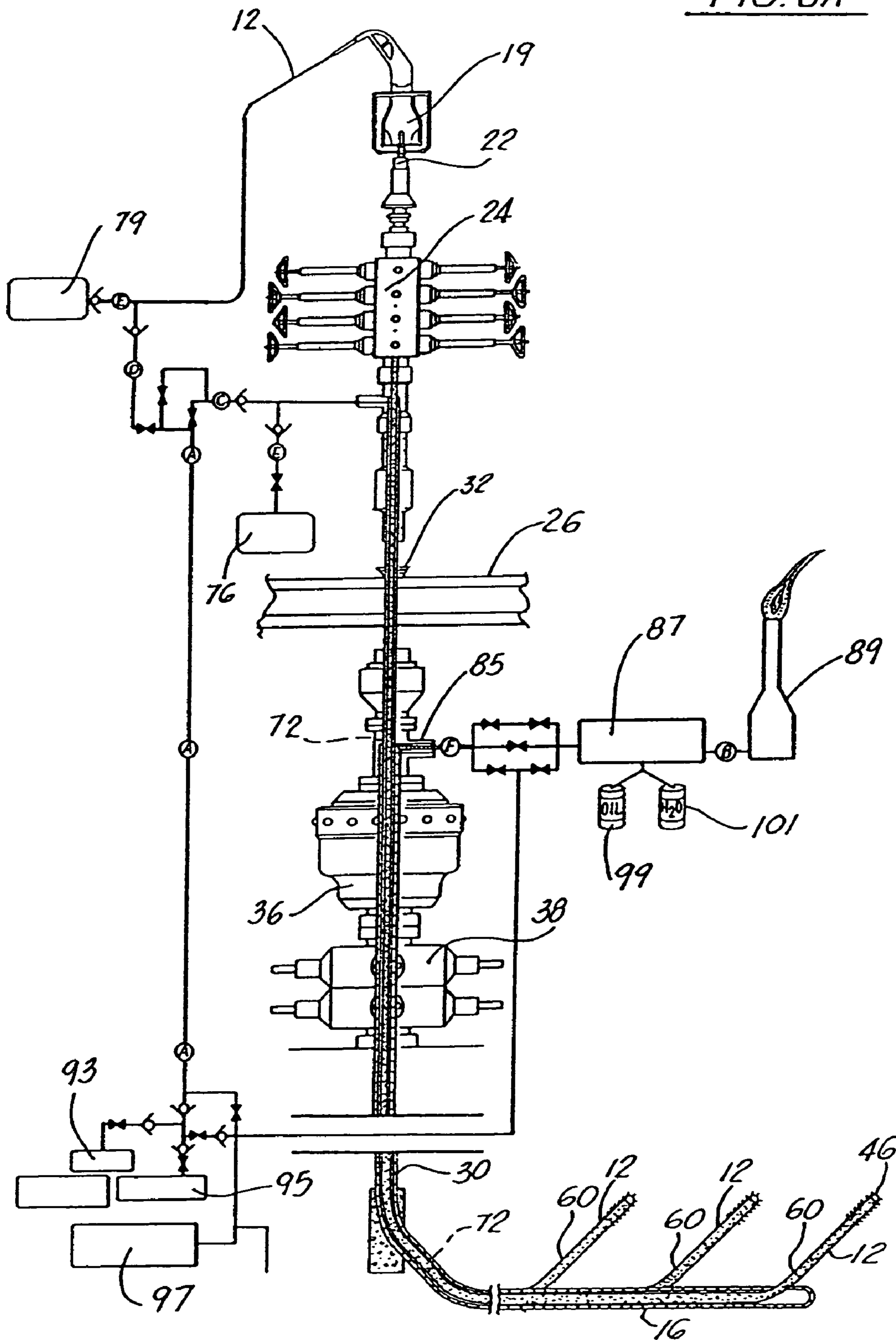
FIG. 8A
