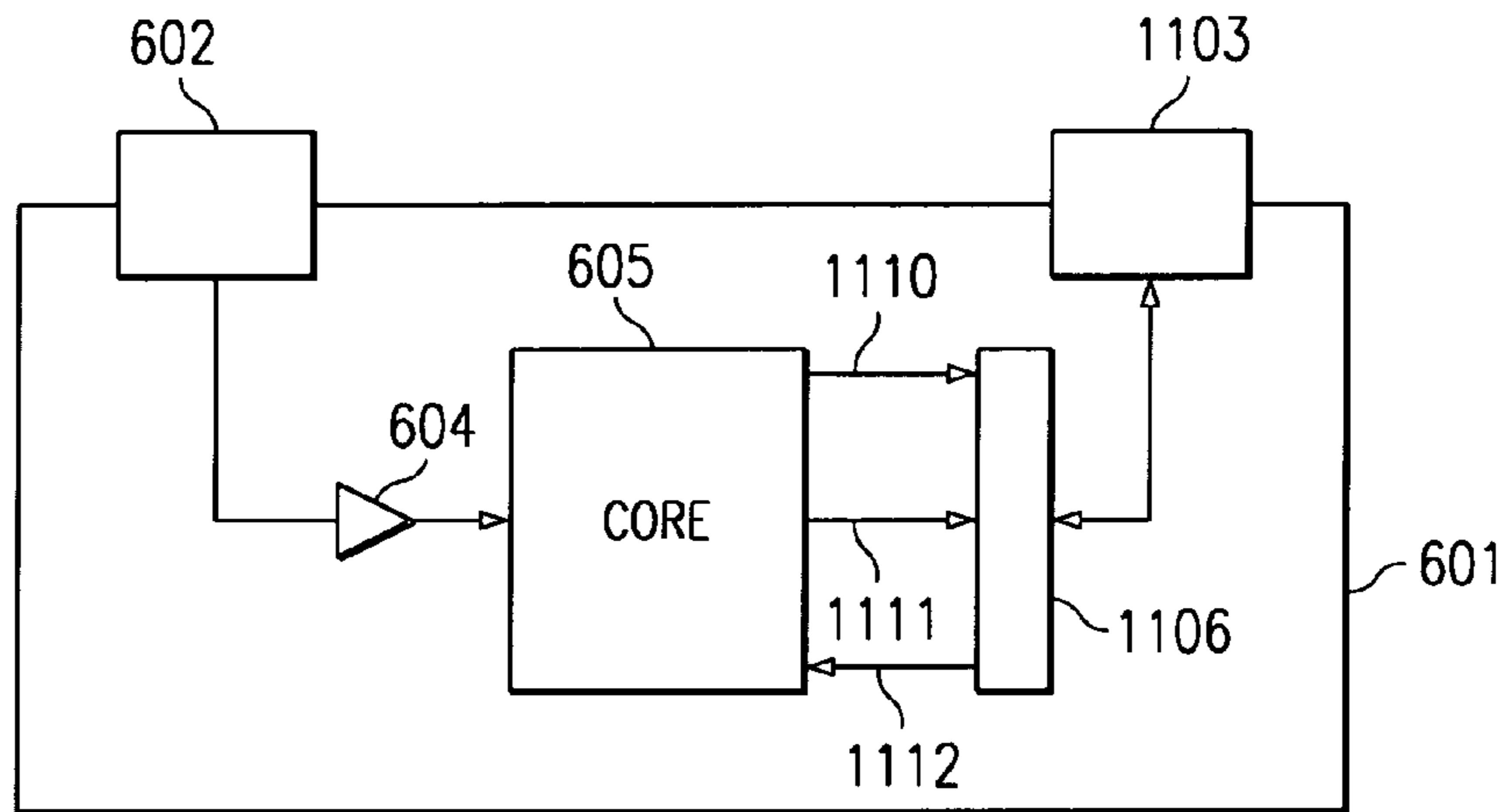
FIG. 11A
