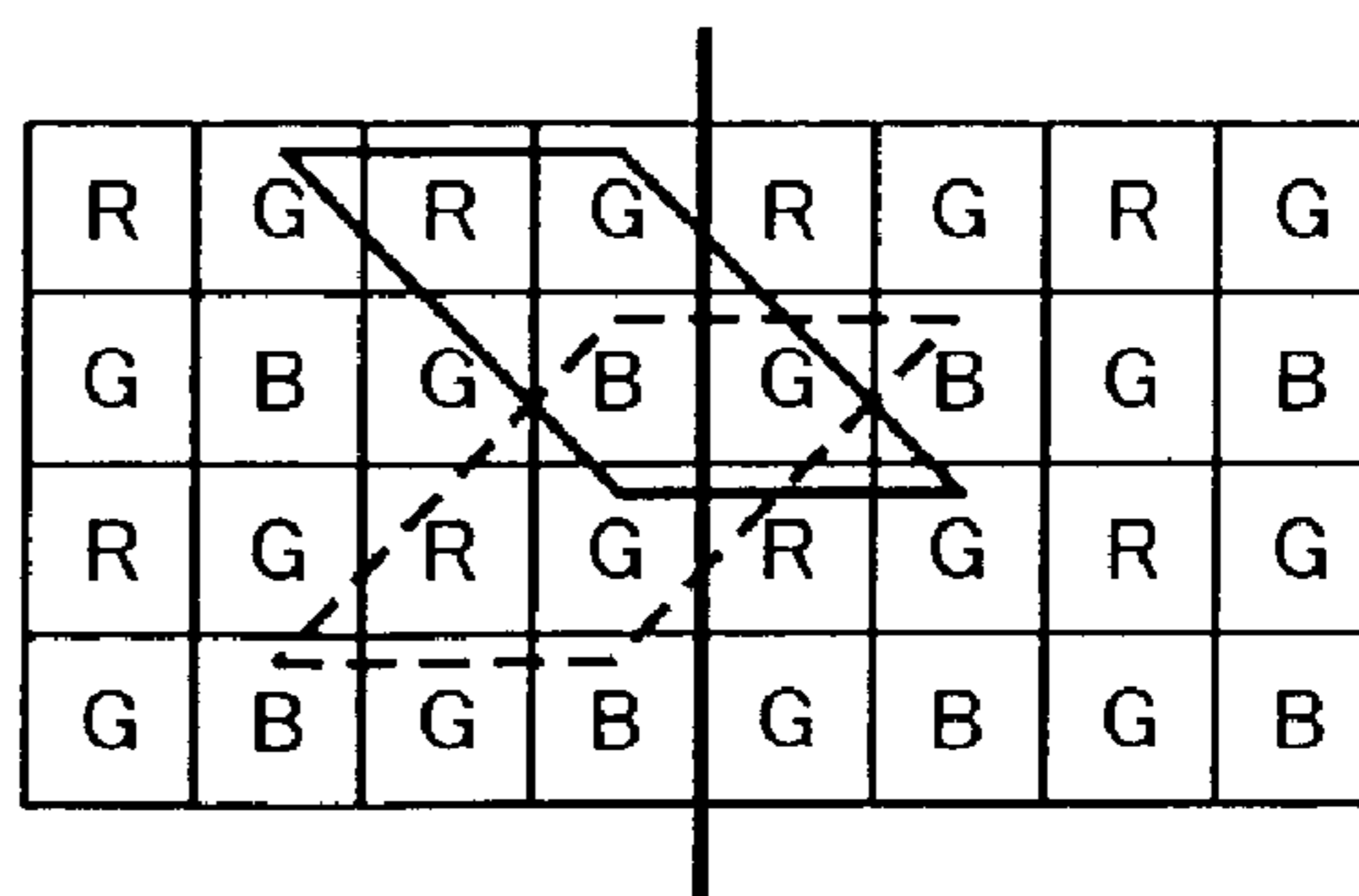
READOUT TYPE IV
