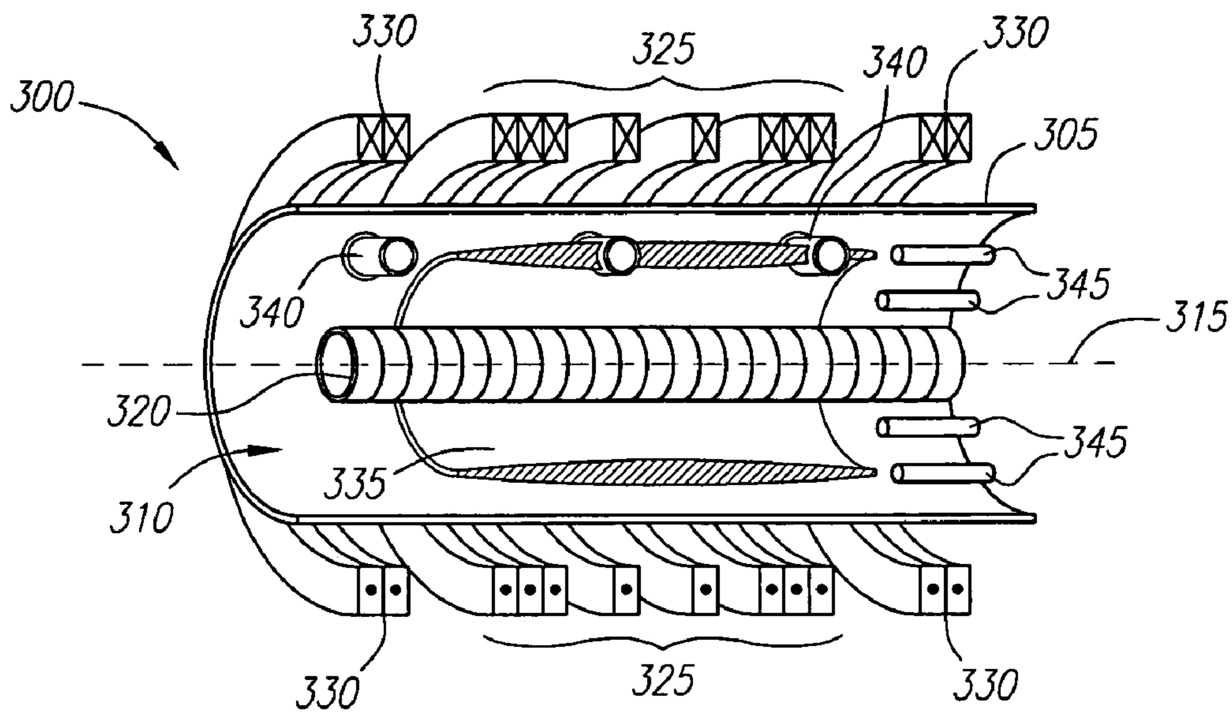
FIG. 25
