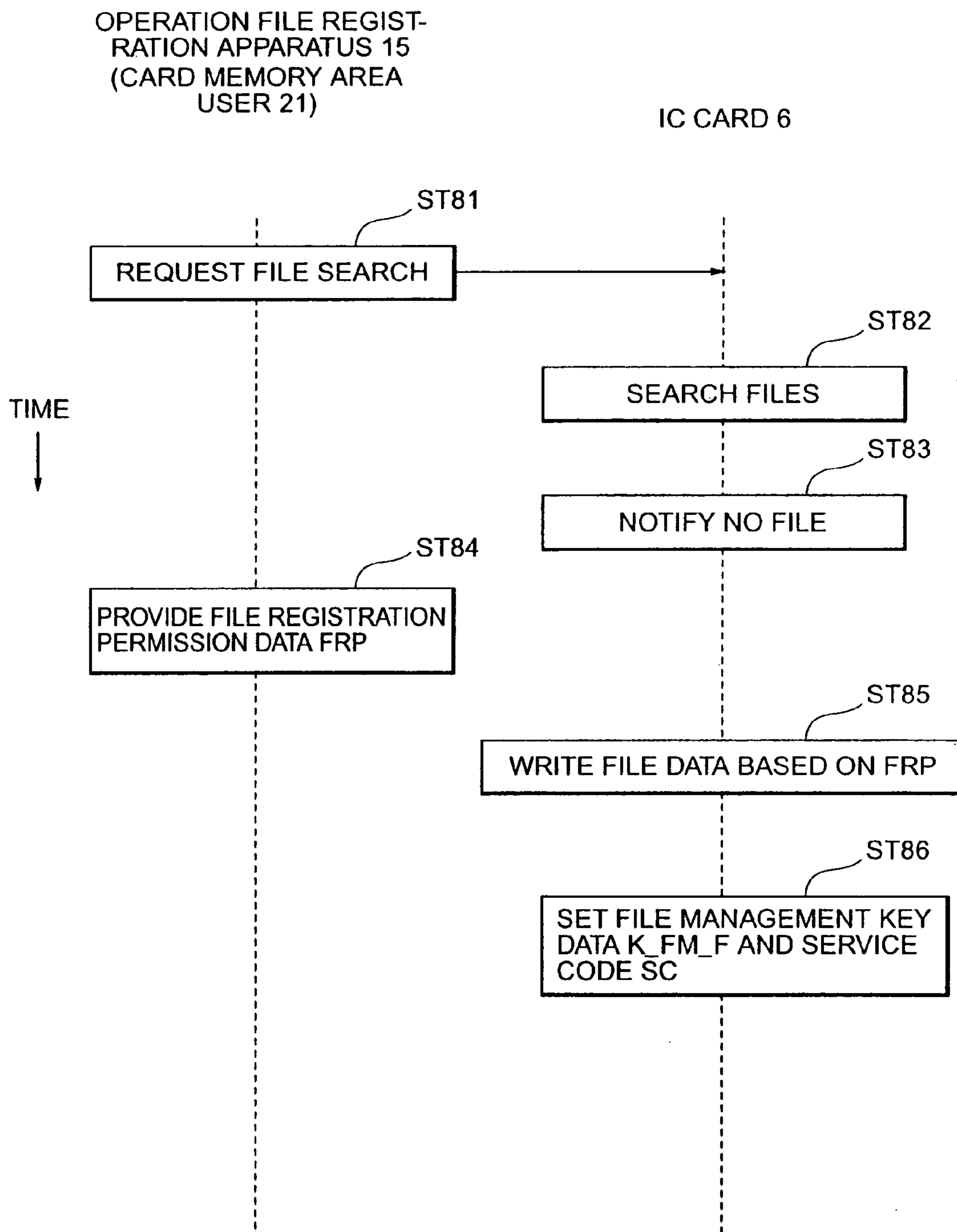
FIG. 24
