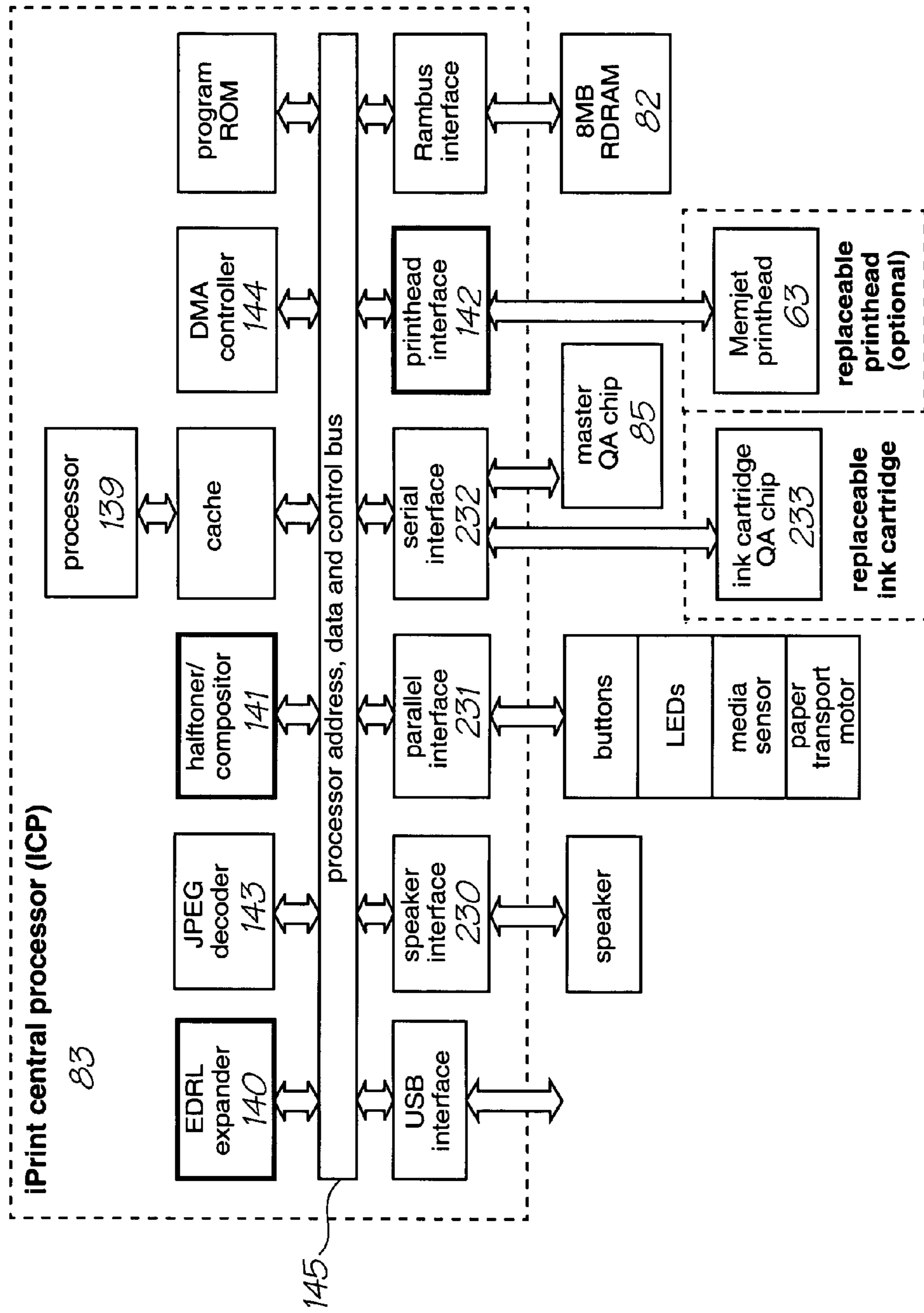
FIG. 17
