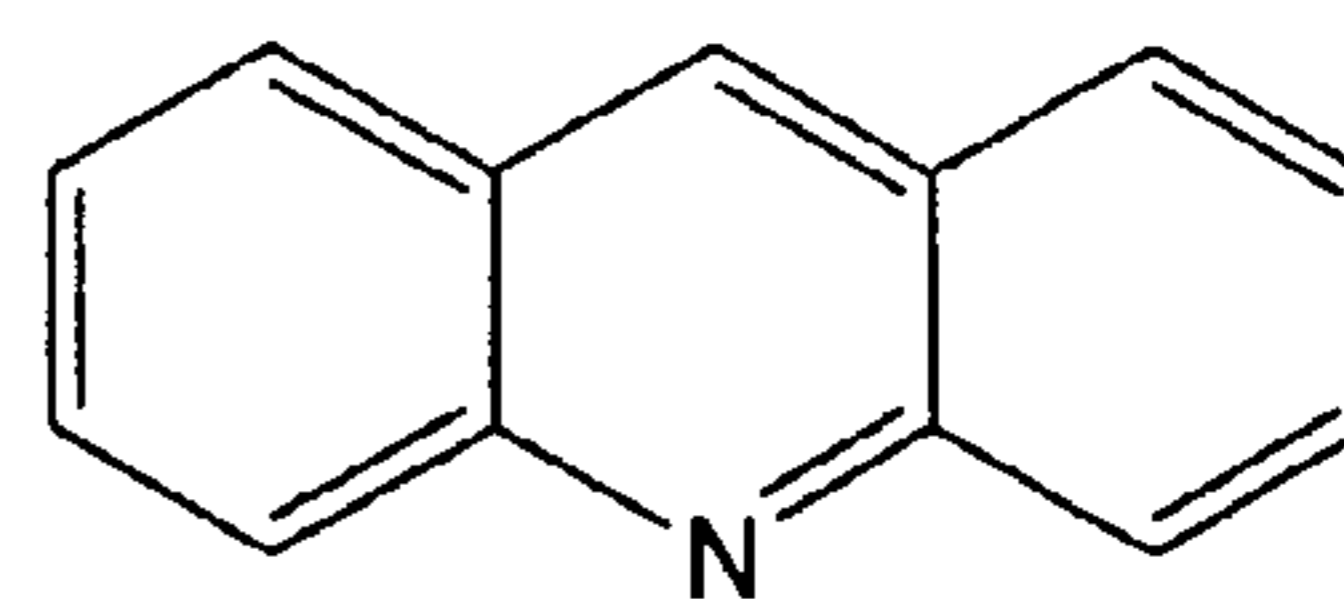
acridine
