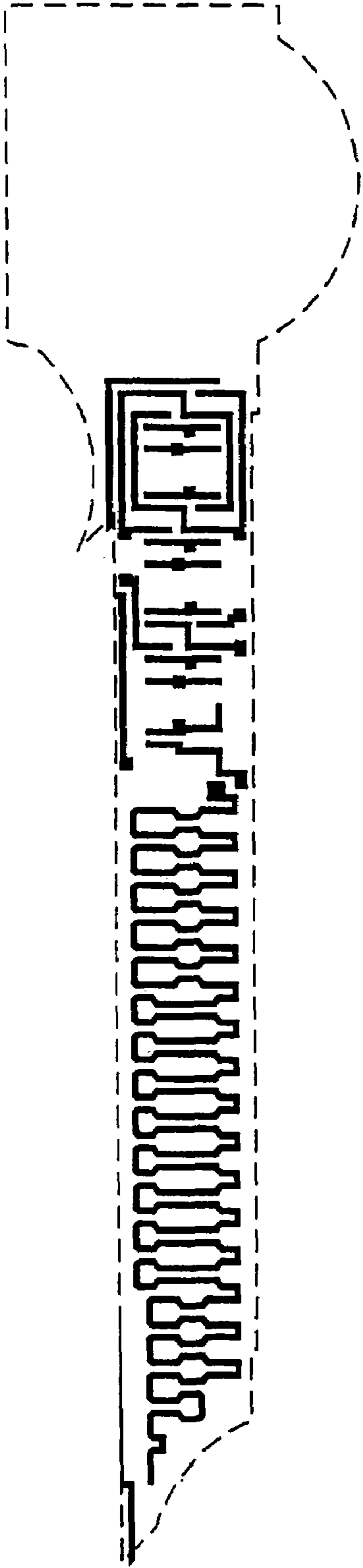
Poly mask
