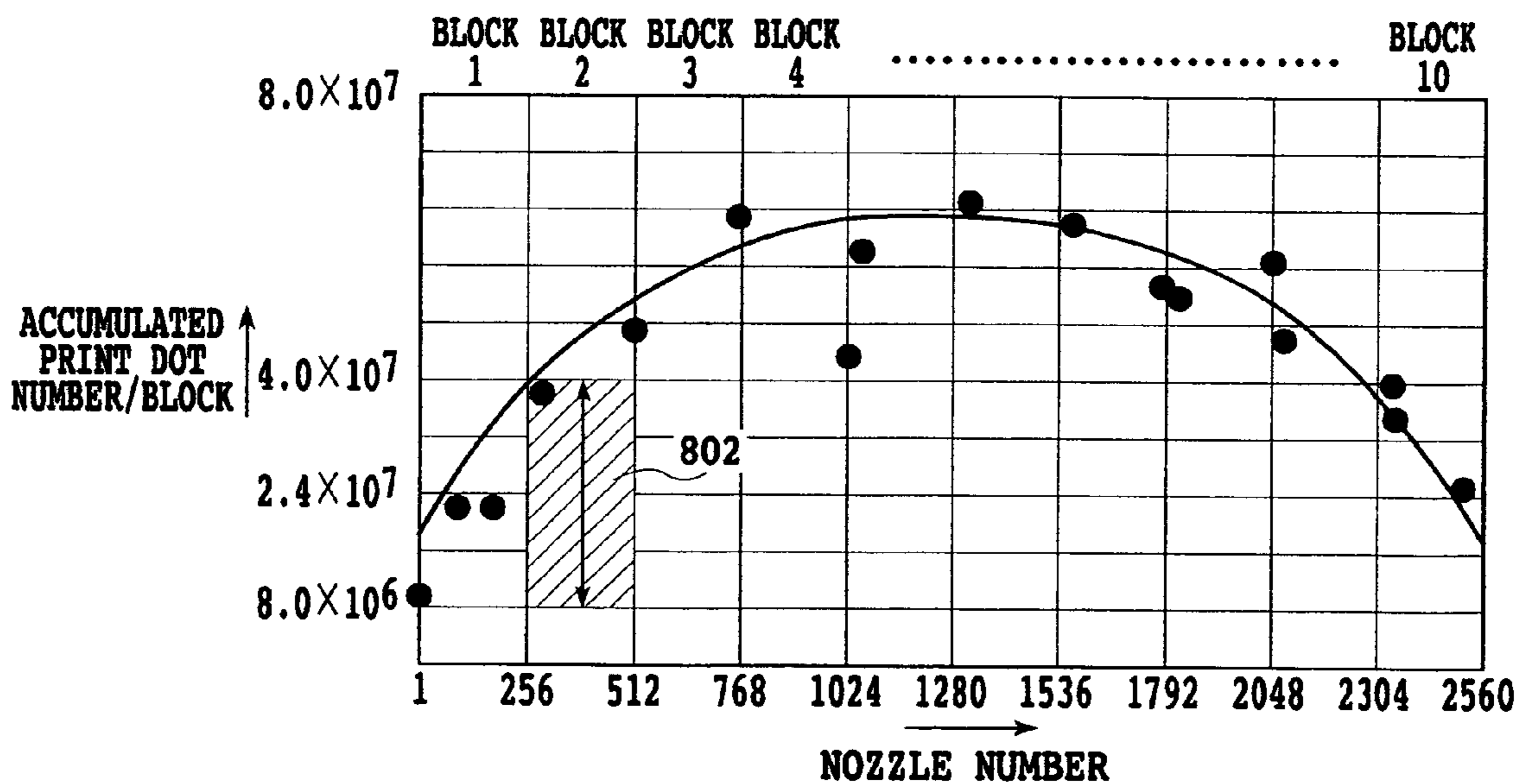
FIG. 8C
