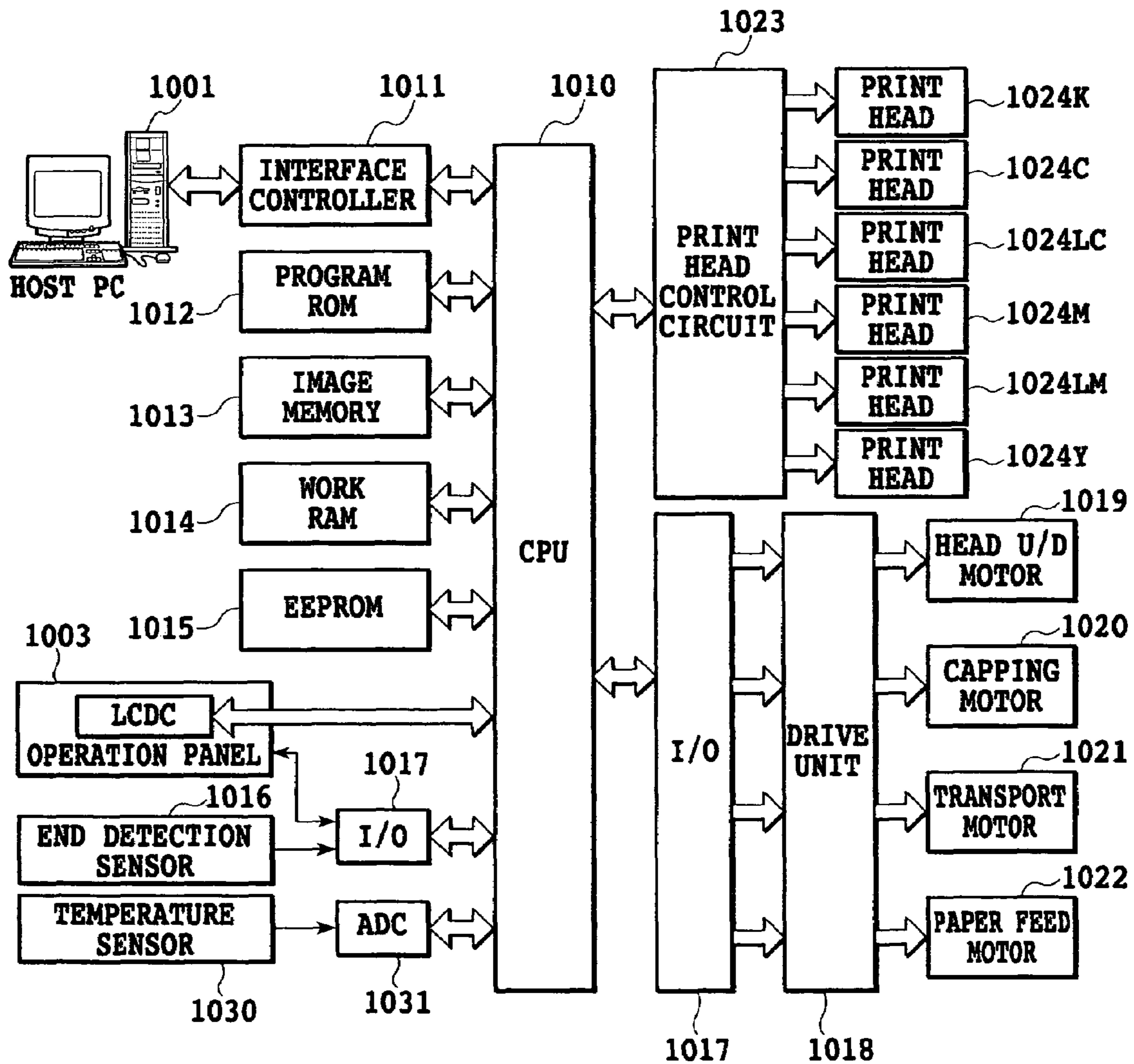
FIG. 10B
