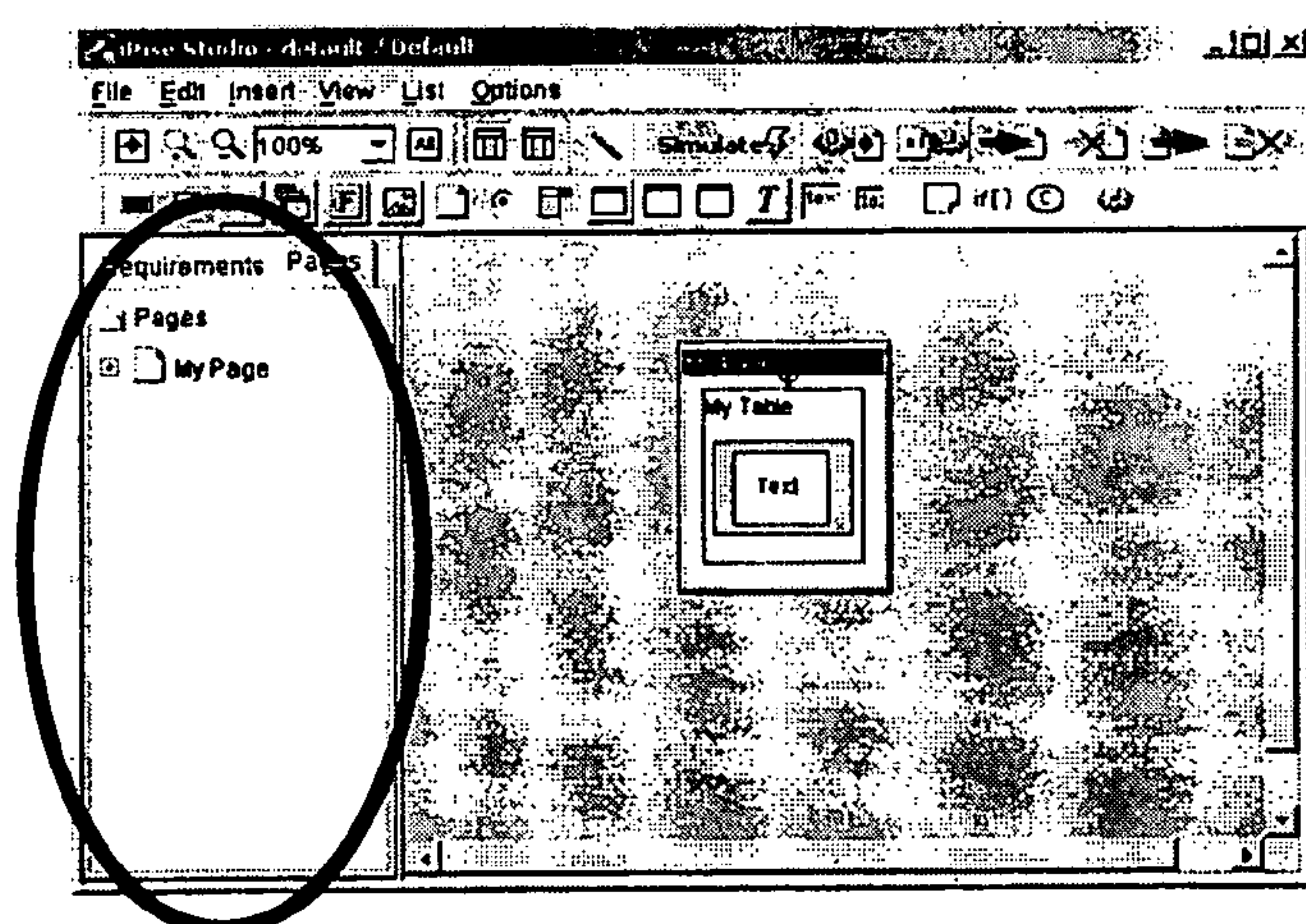
Project Browser
