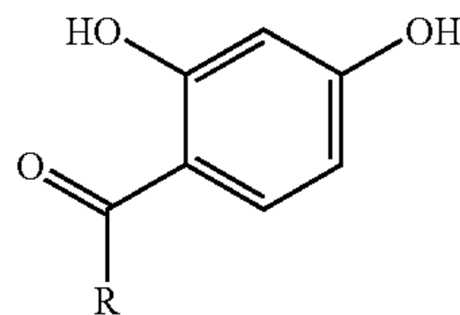
a 4-acylresorcinol
