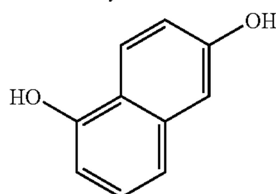
a 1,6-naphthalenediol
