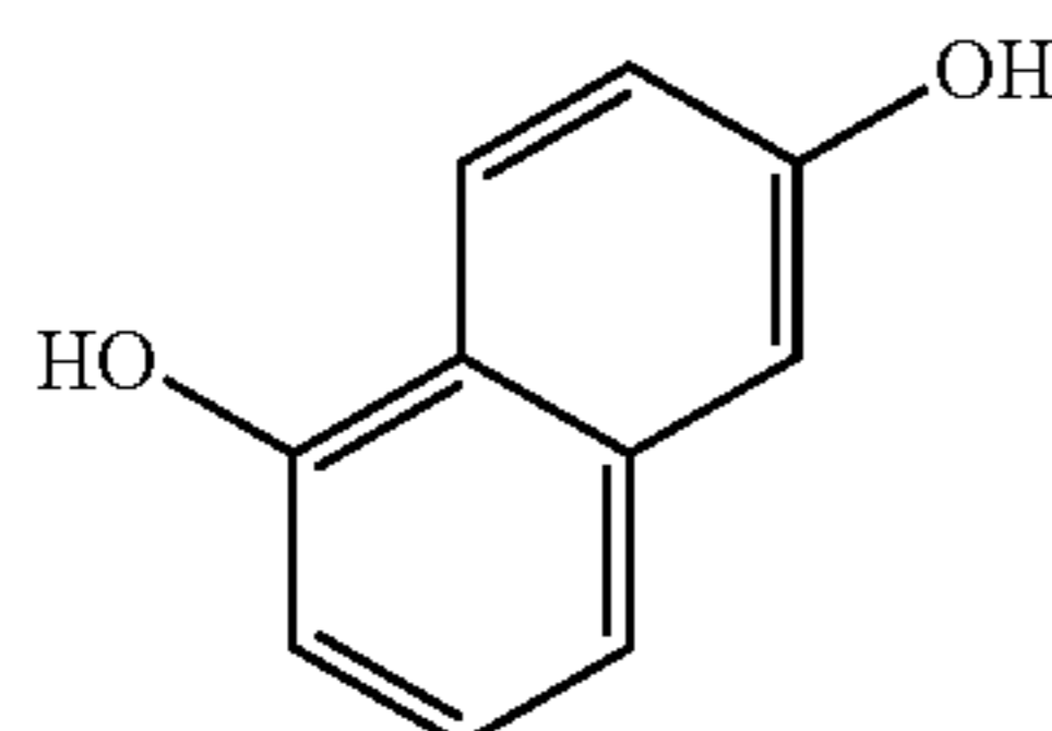
a 1,6-naphthalenediol
