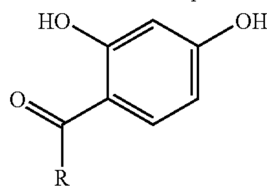
a 4-acylresorcinol
