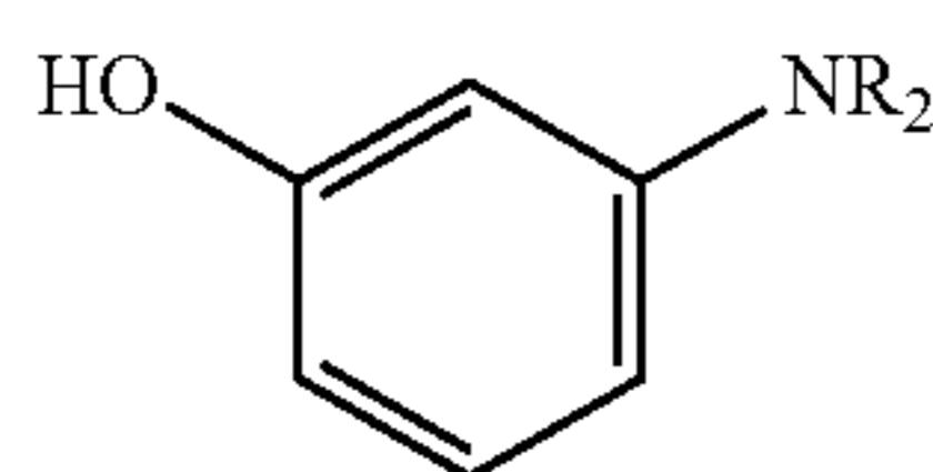
a 3-aminophenol
