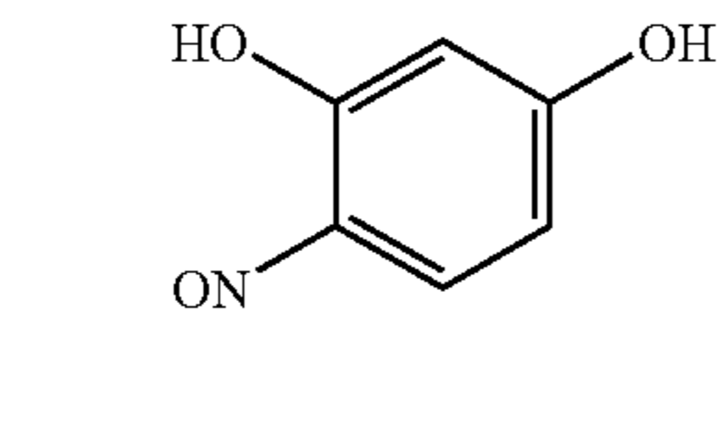
a 4-nitrosoresorcinol
