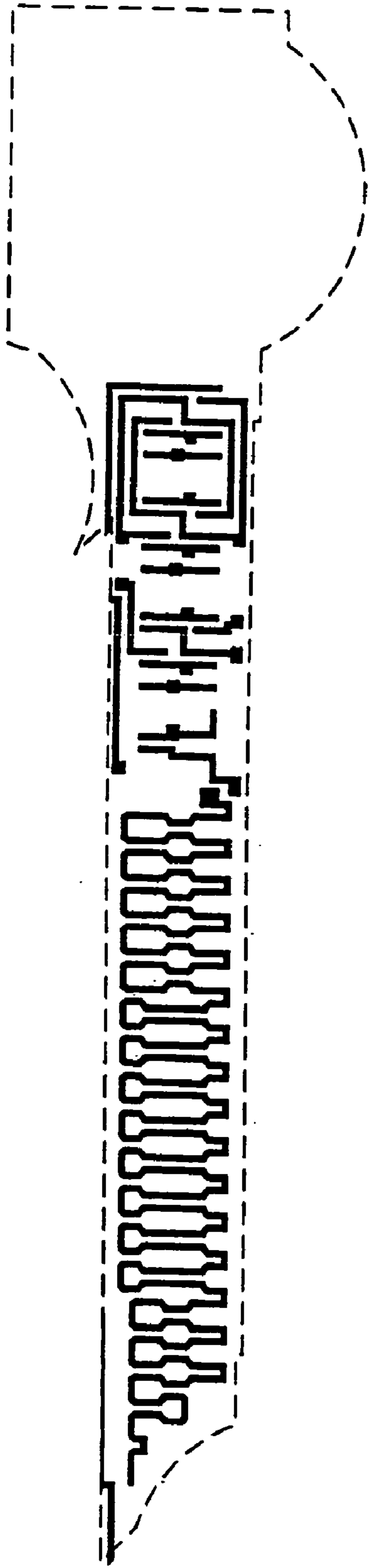
Poly mask
