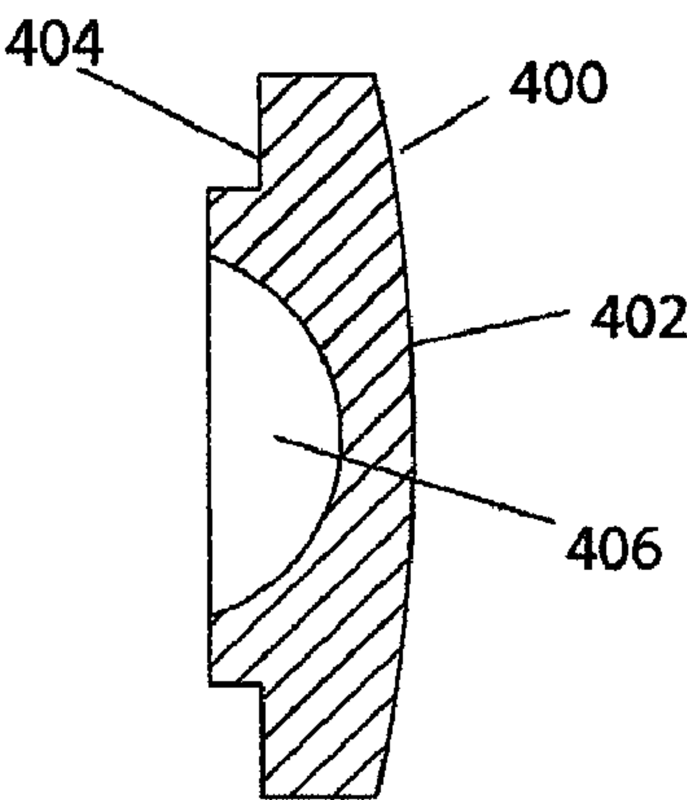
A-A FIG. 3r
