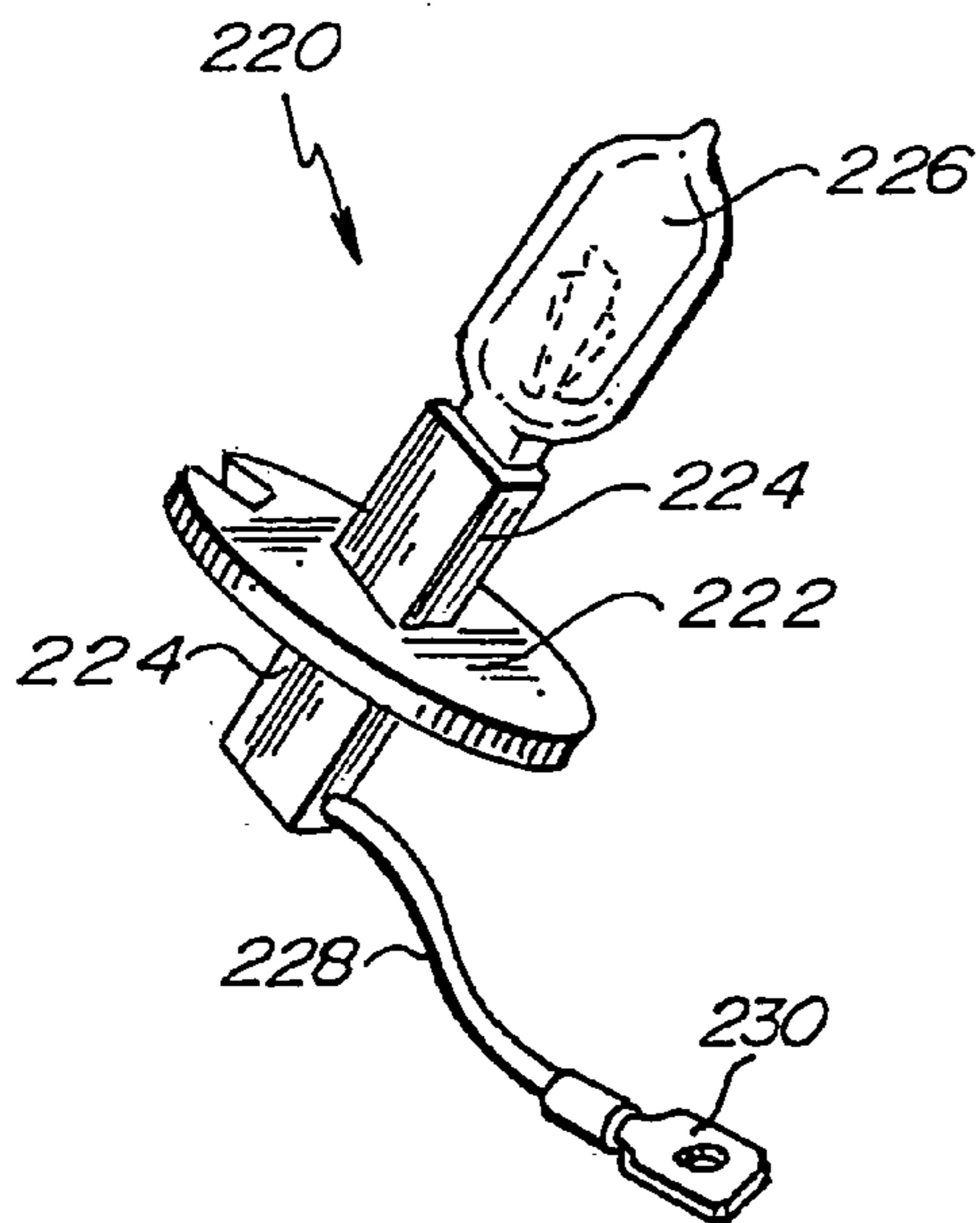
Fig. 18. PRIOR ART
