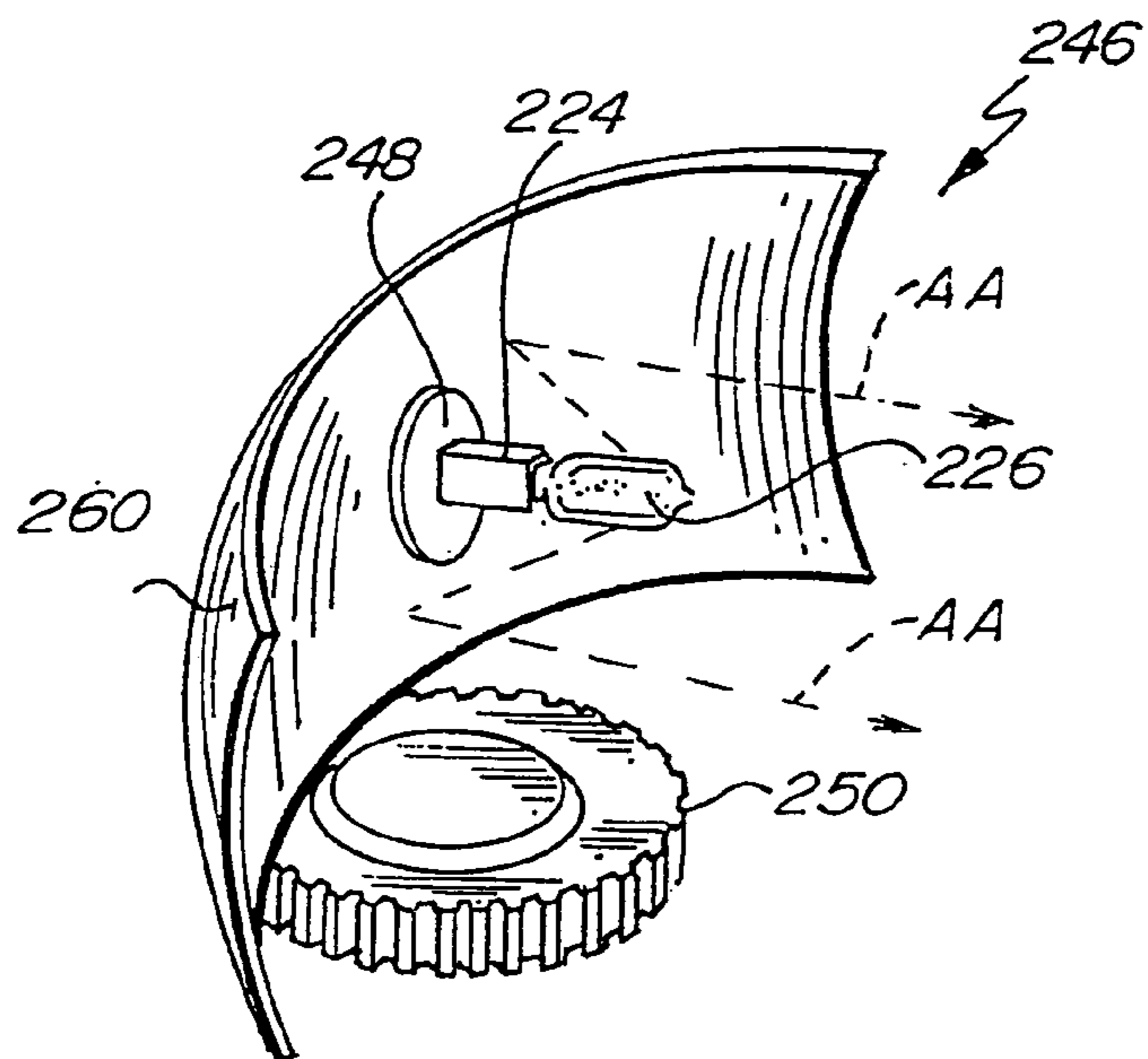
Fig. 20. PRIOR ART
