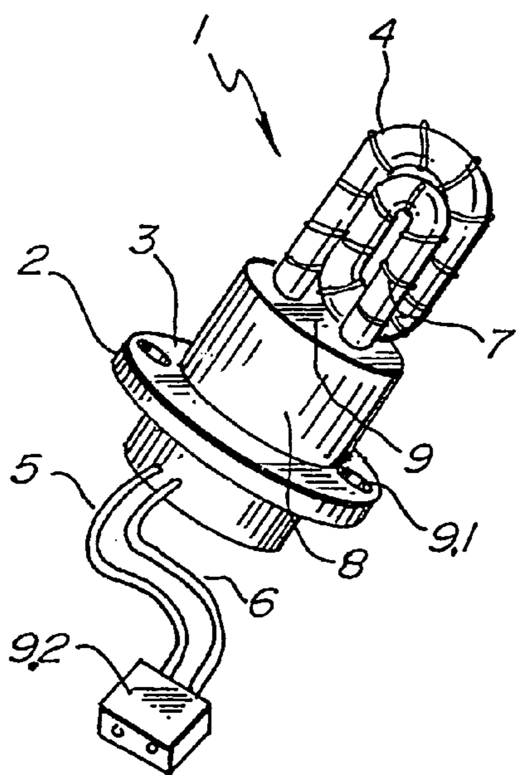
Fig. 16. PRIOR ART
