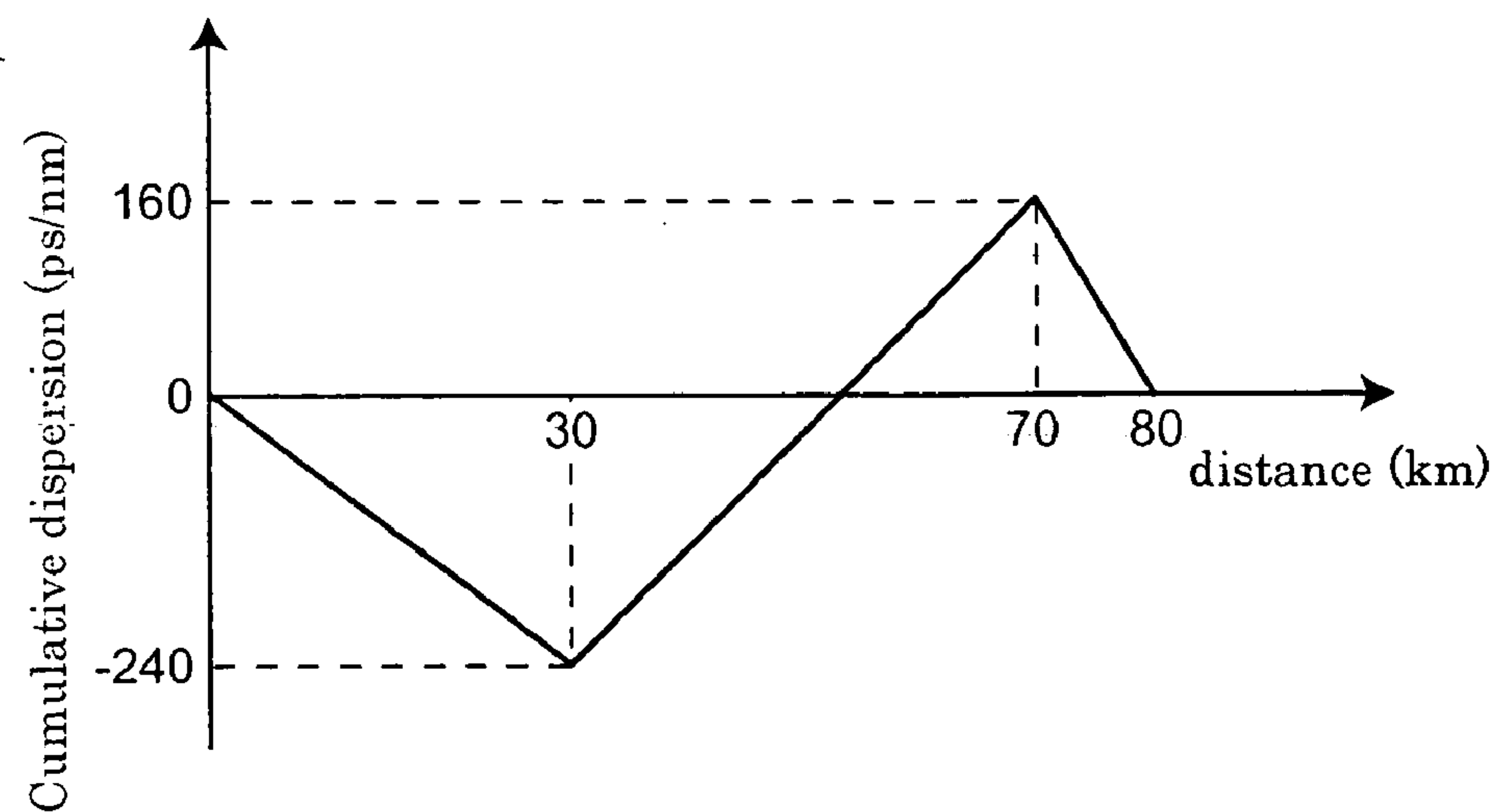
FIG. 2A
