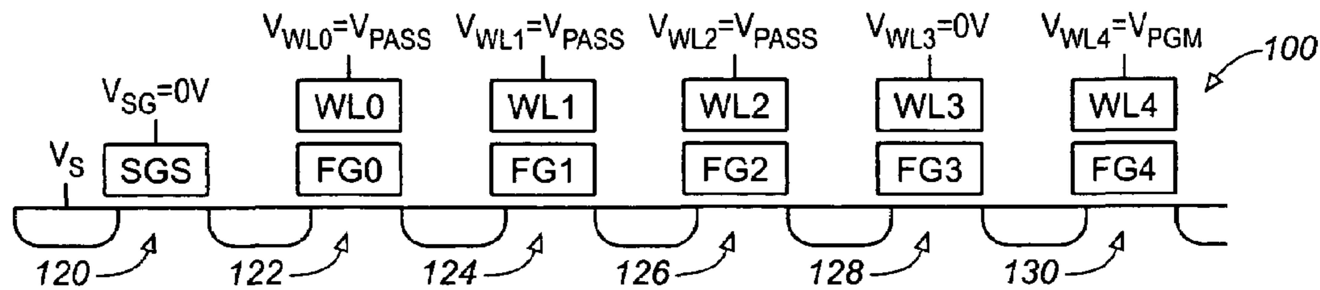
FIG. 6E (PRIOR ART)
