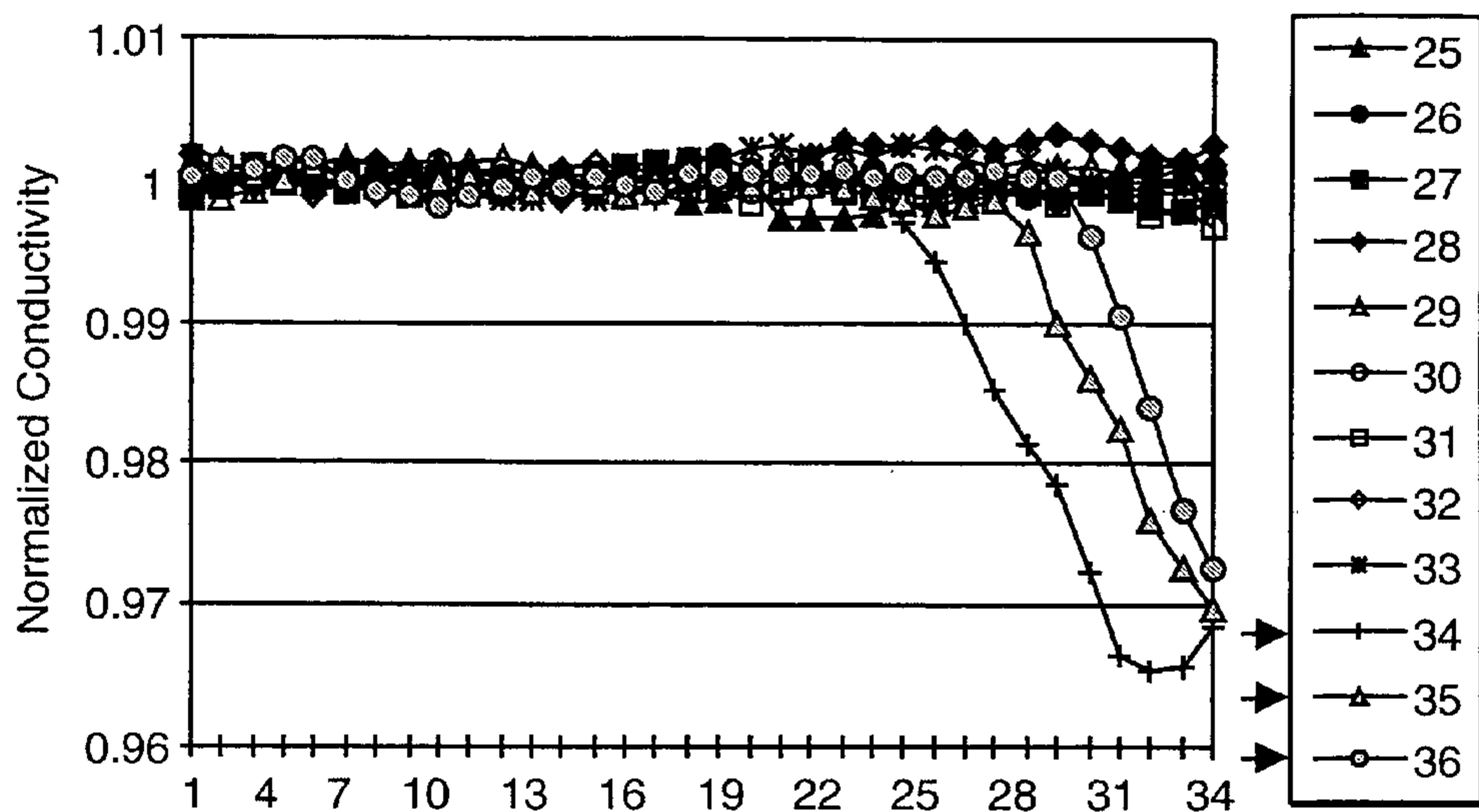
FIG. 44c Position (1/16" increments)
