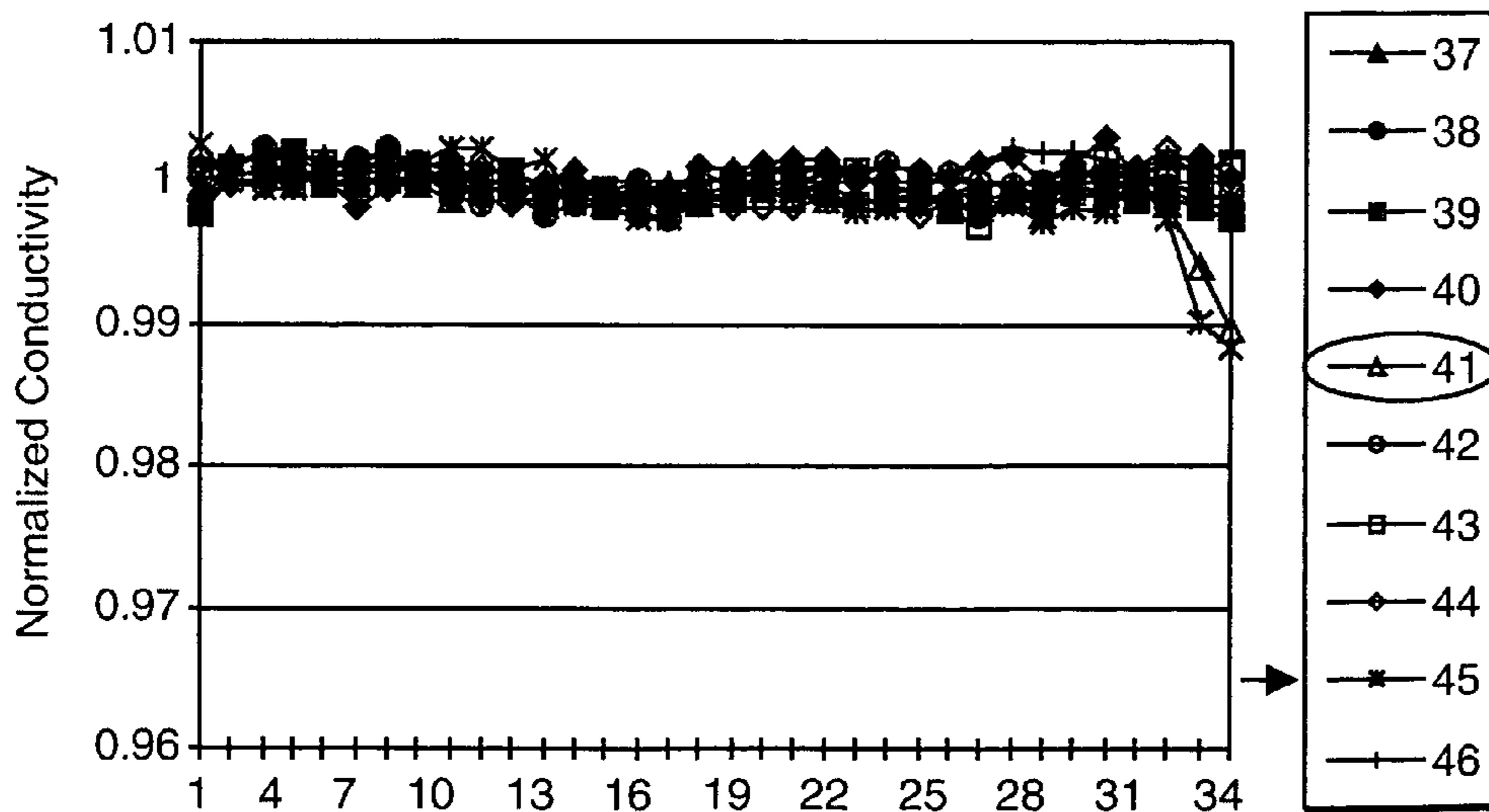
Position (1/16" increments)
