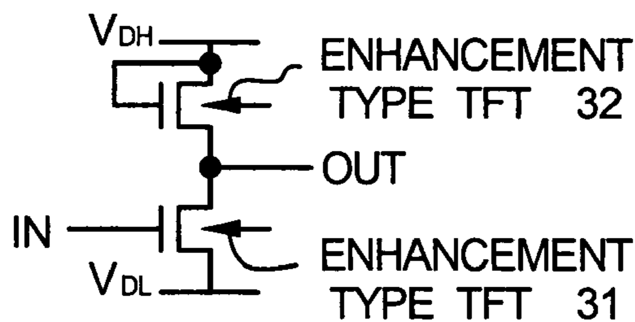
FIG. 8A EEMOS CIRCUIT
