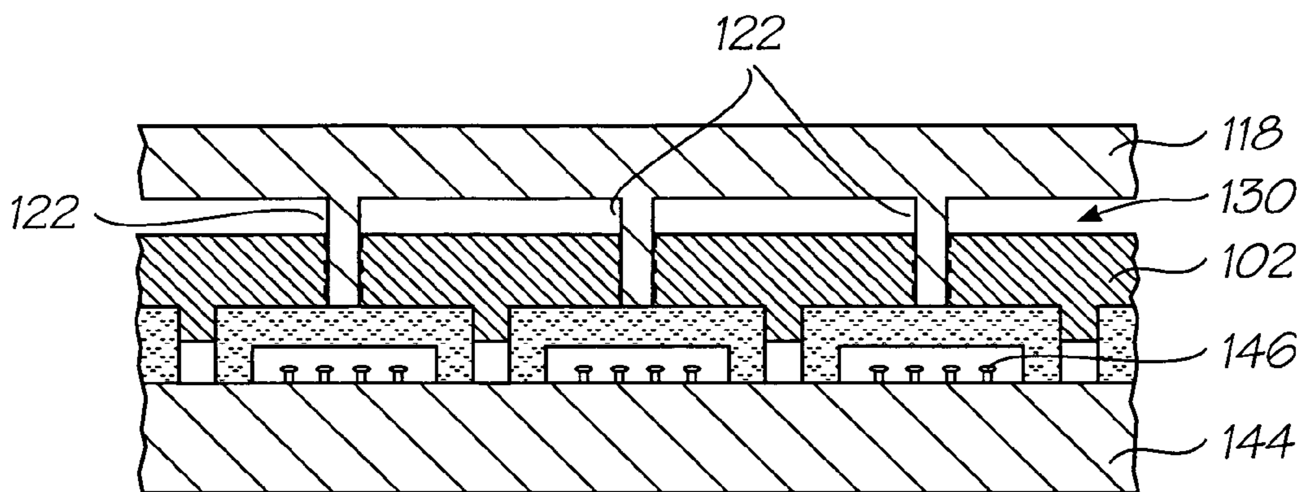
FIG. 19
