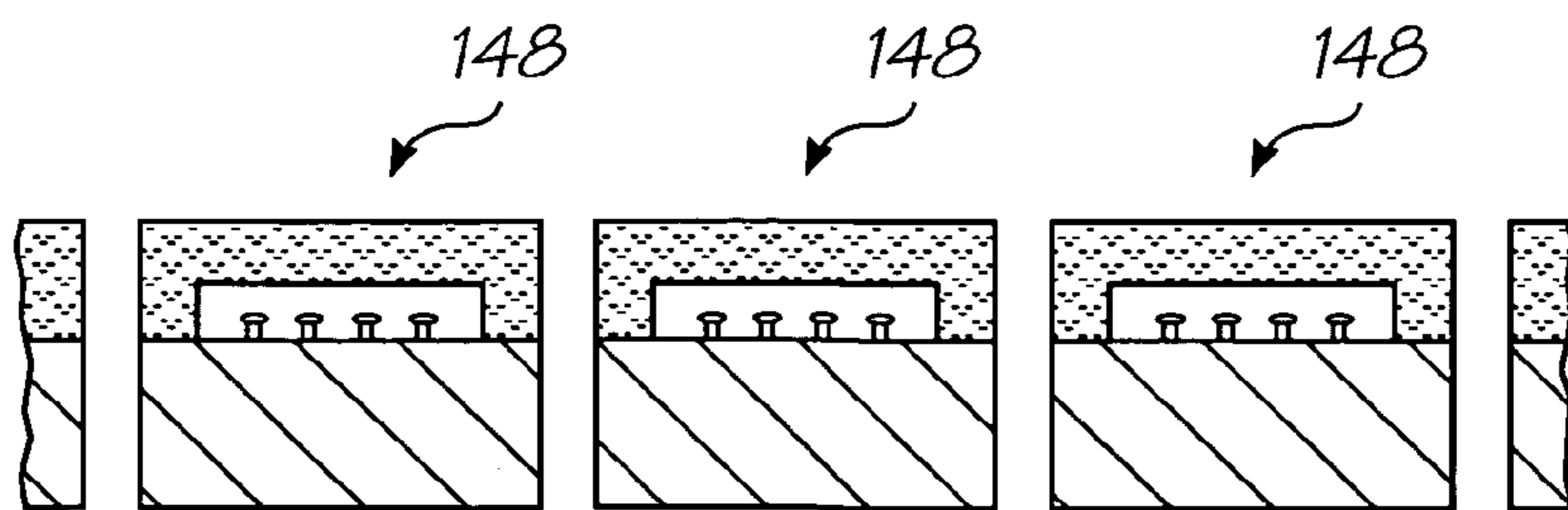
FIG. 21
