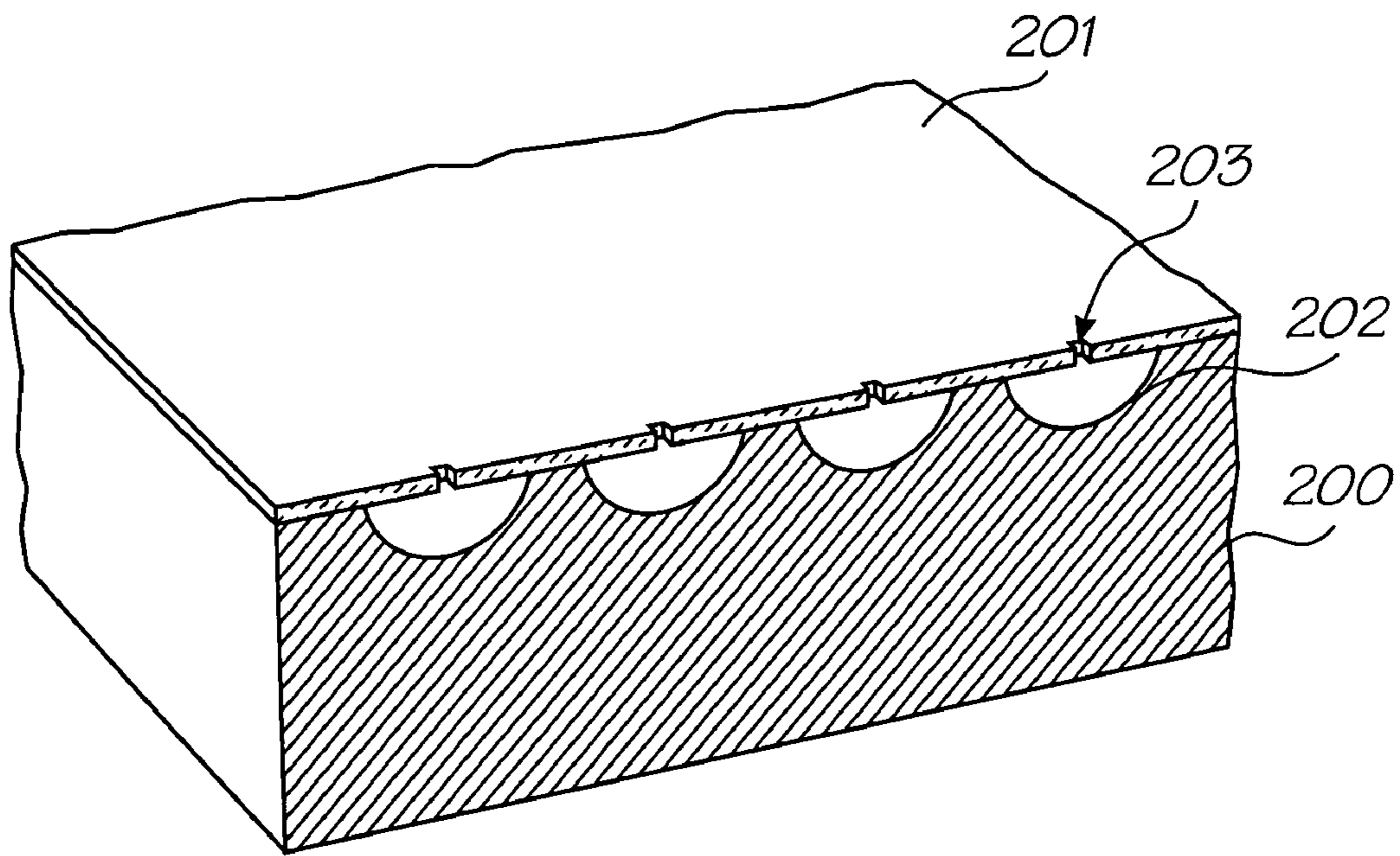
FIG. 23a
