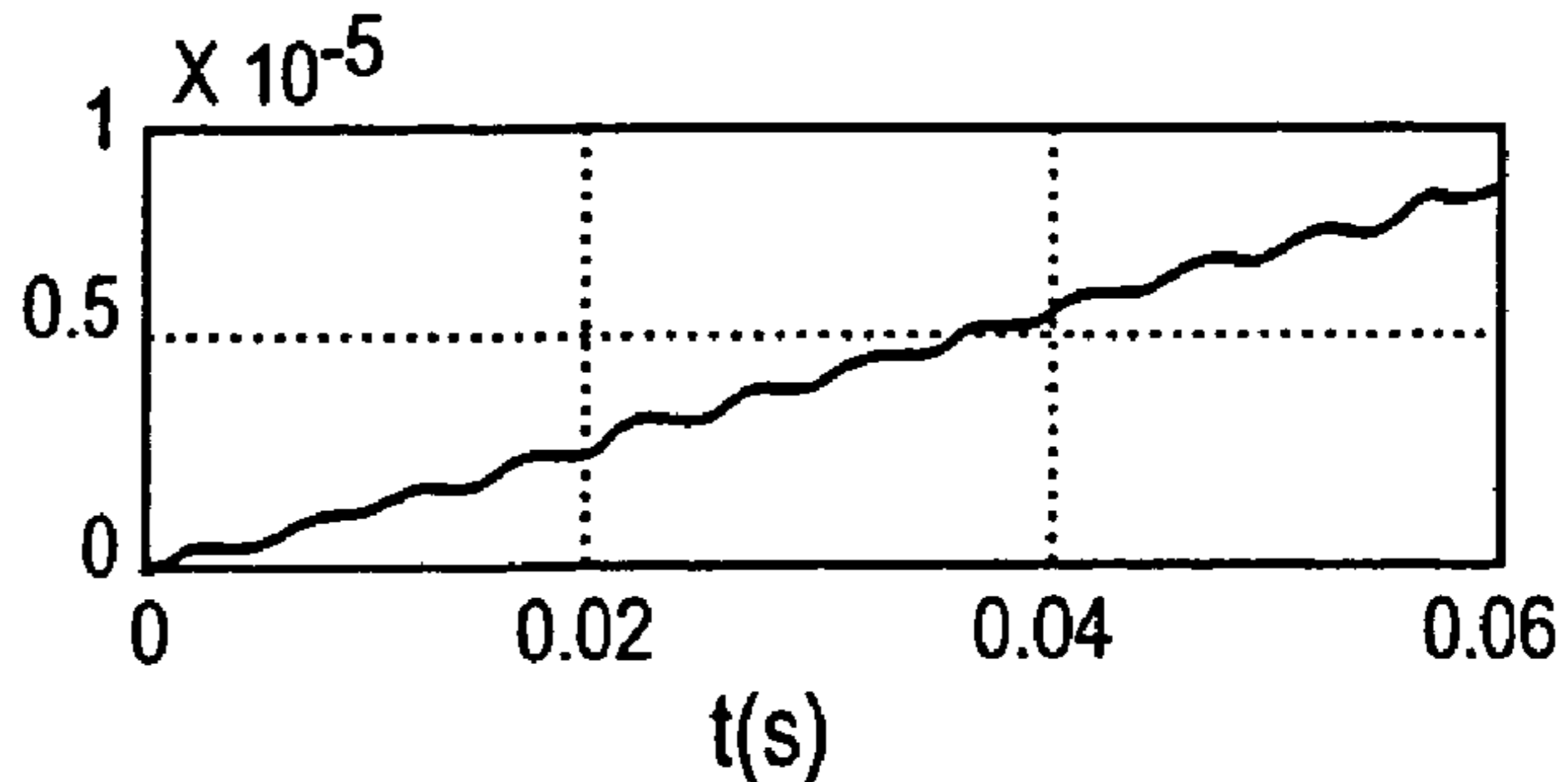
FIG. 18F E_{\text{EXTRACT}}(J)
