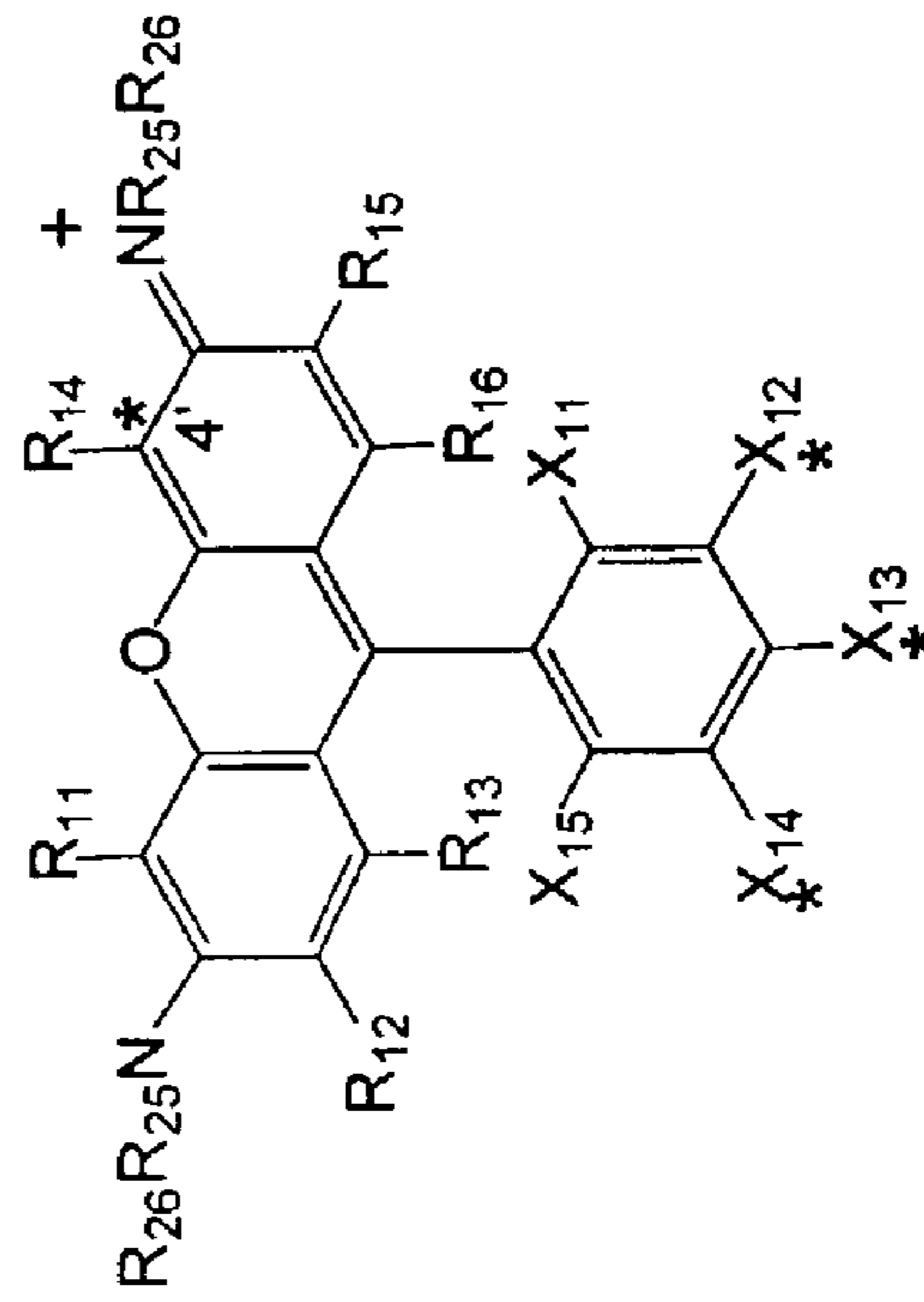
RHODAMINE
