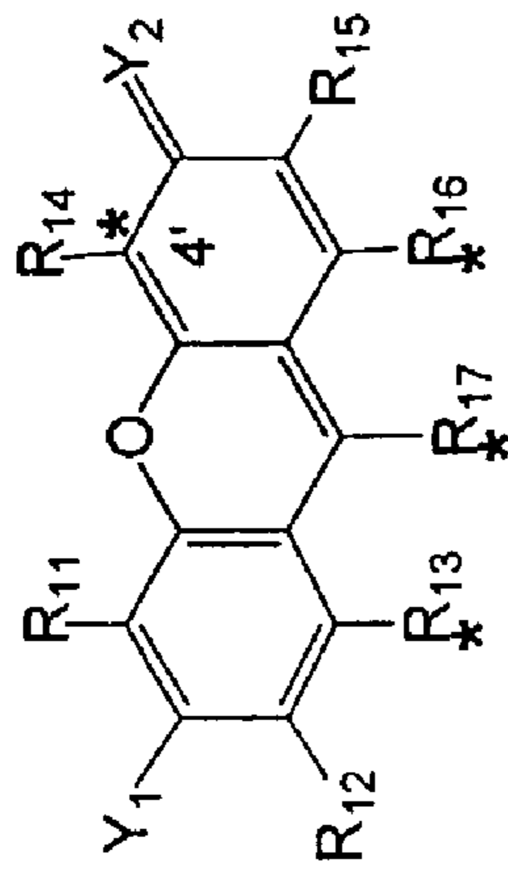
XANTHENE
