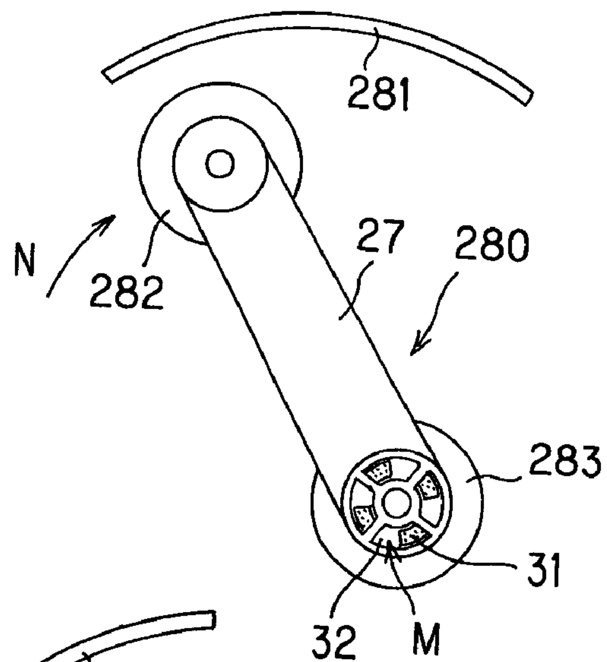
FIG. 8B
