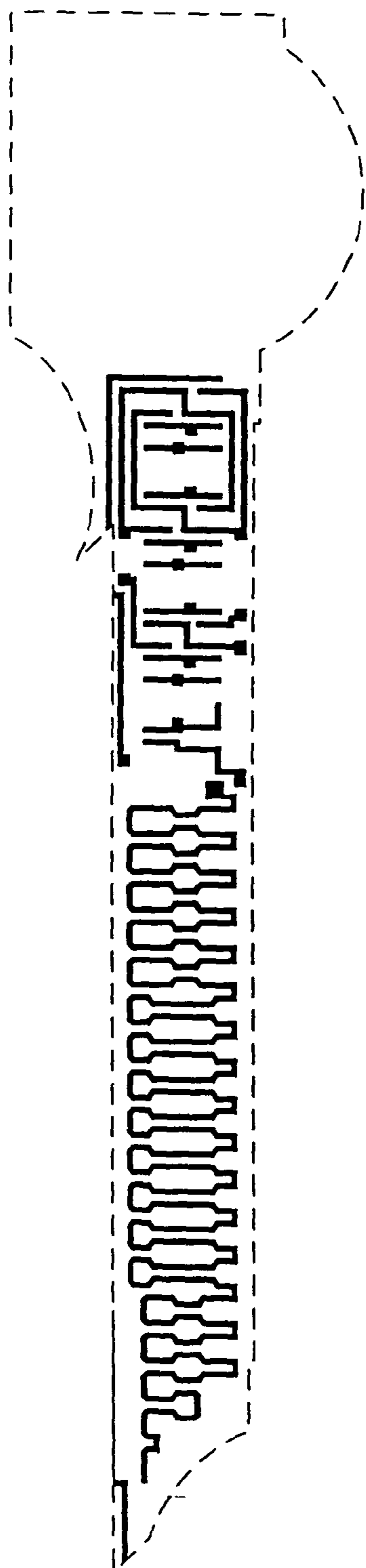
Poly mask
