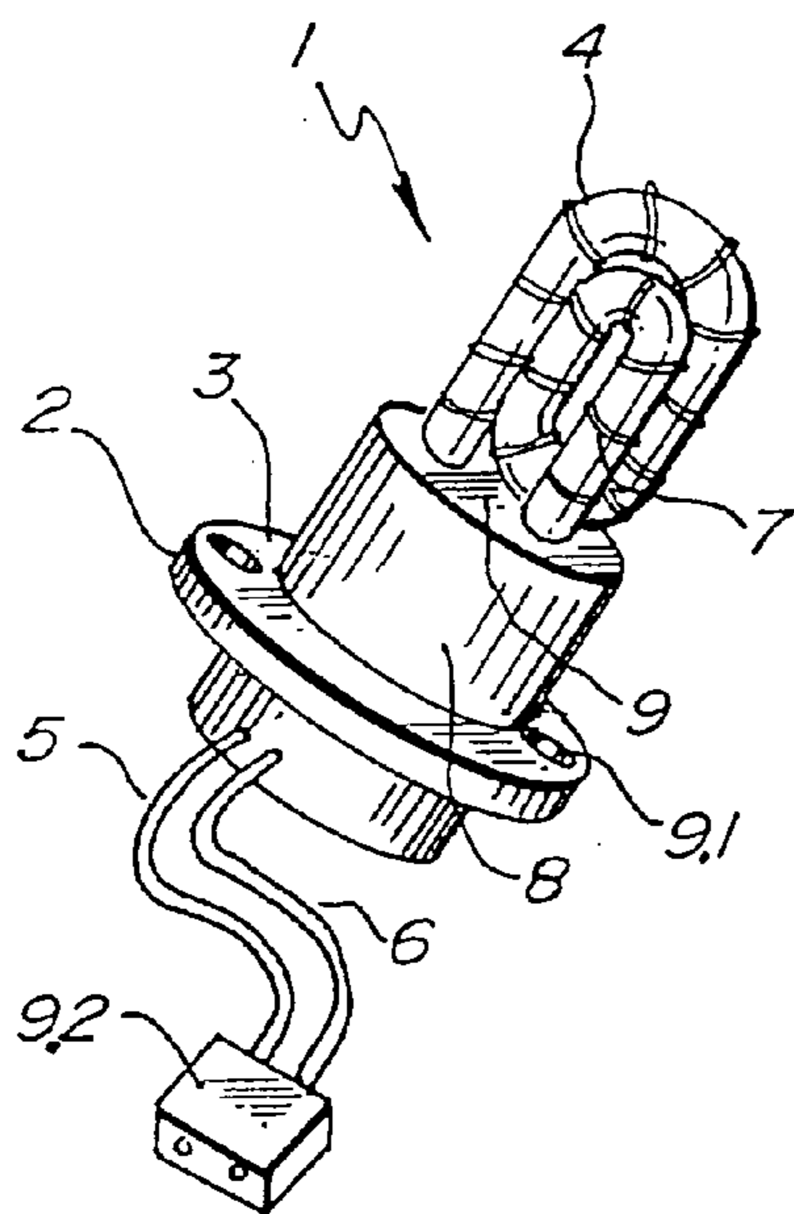
Fig. 16. PRIOR ART
