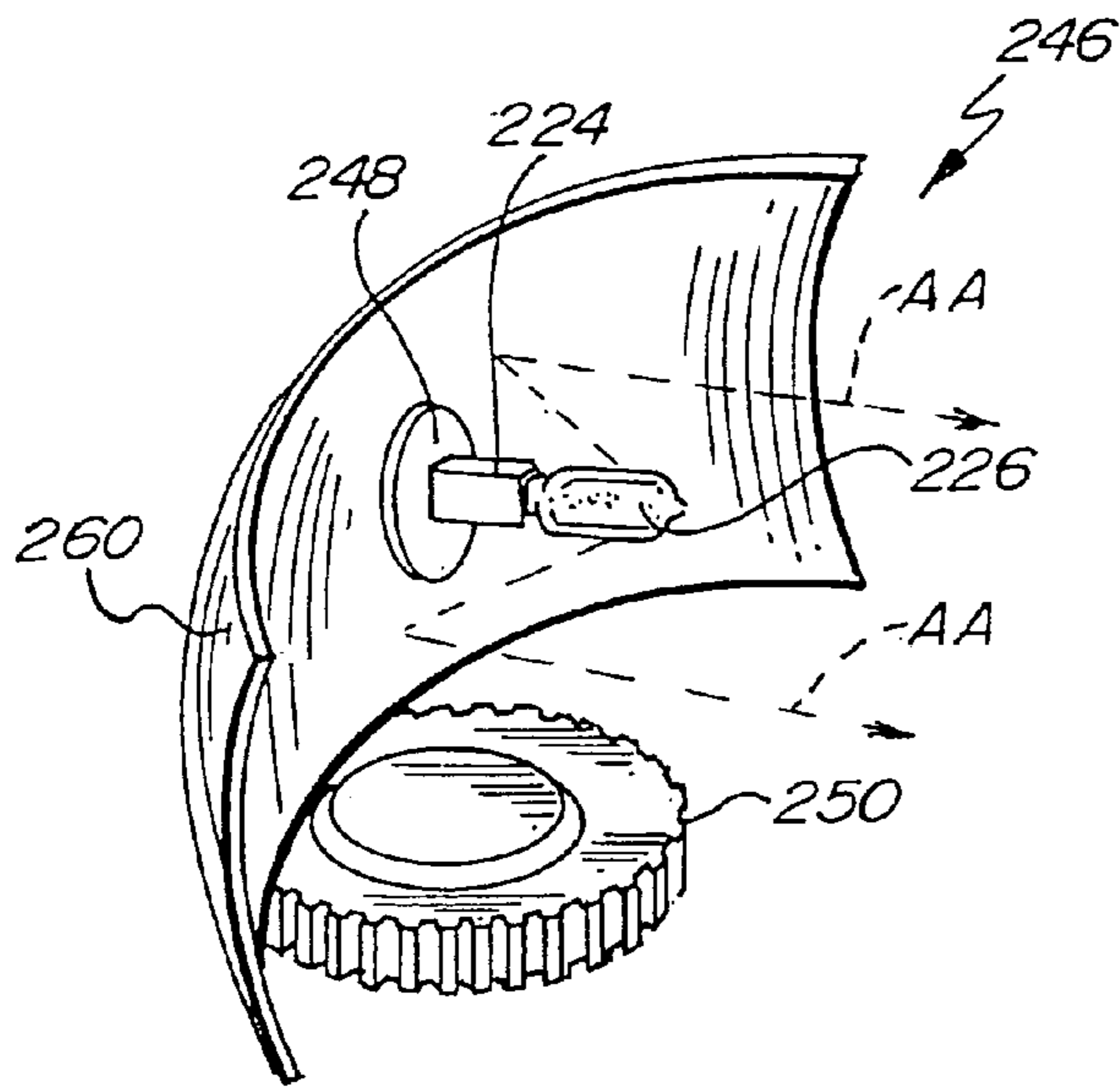
Fig. 20. PRIOR ART
