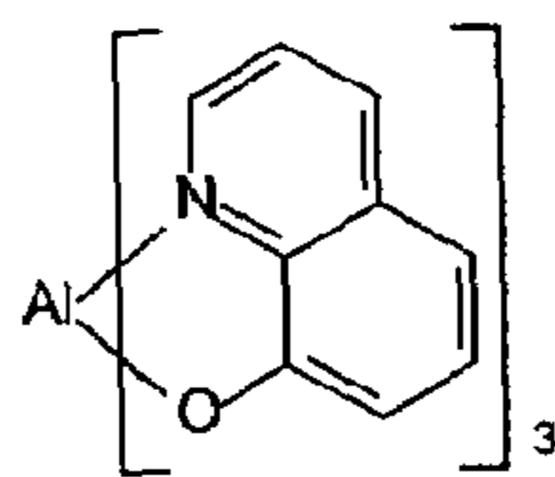
Alq 3
