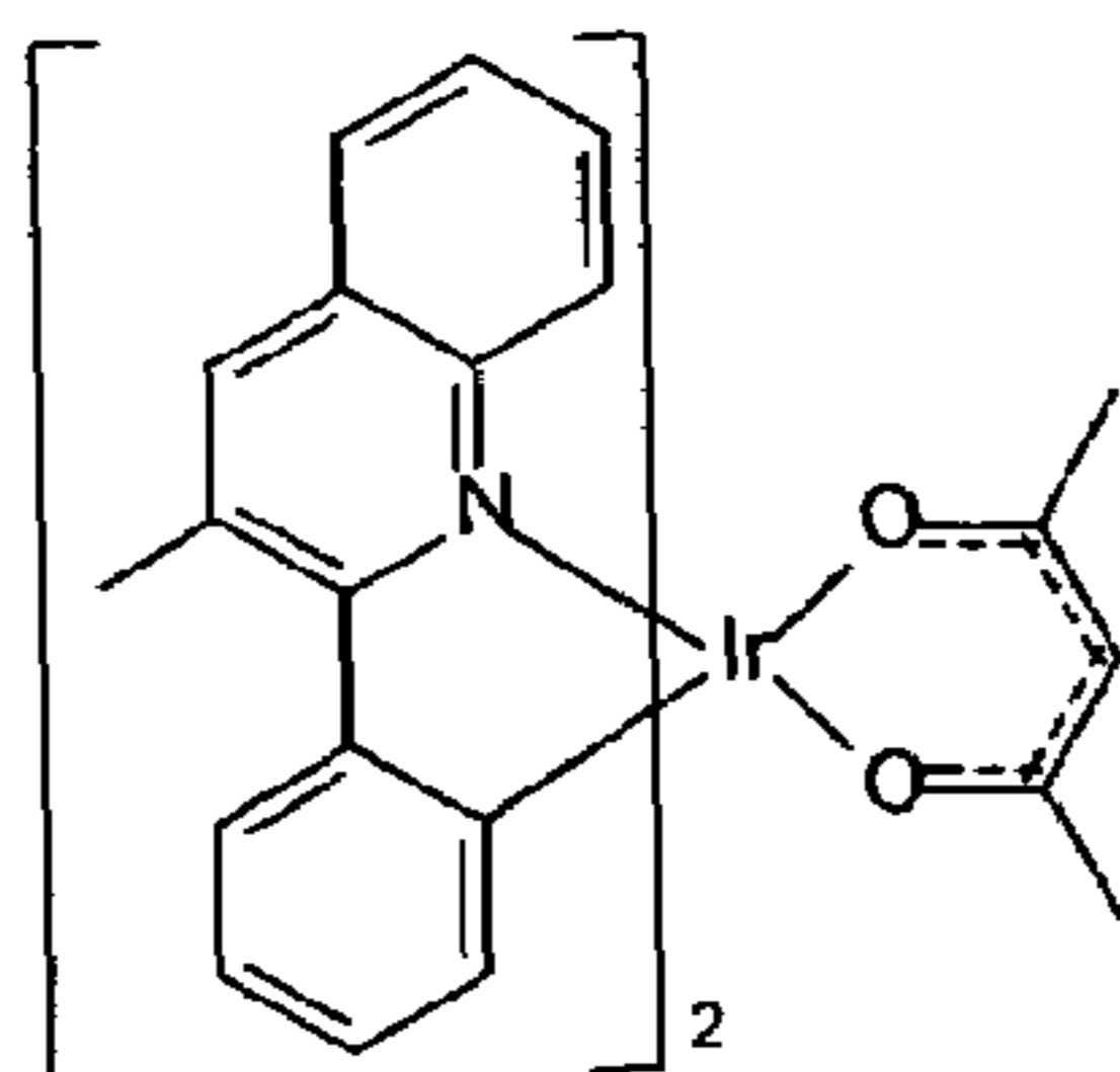
Ir(3-Mepq) 2 (acac)
