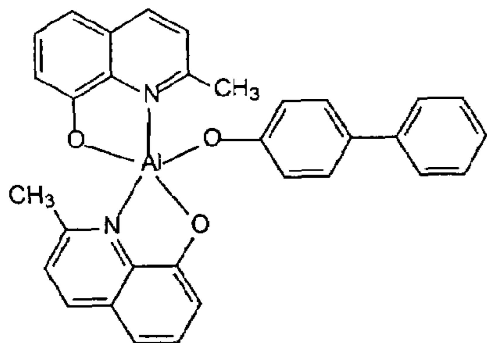
BAlq
