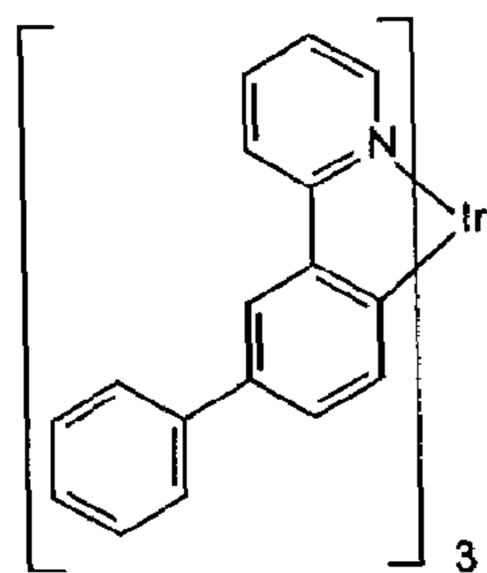
Ir(Ph-ppy)
