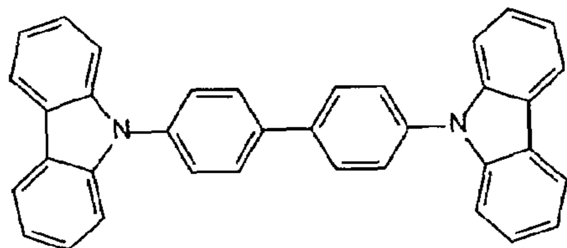
CBP
