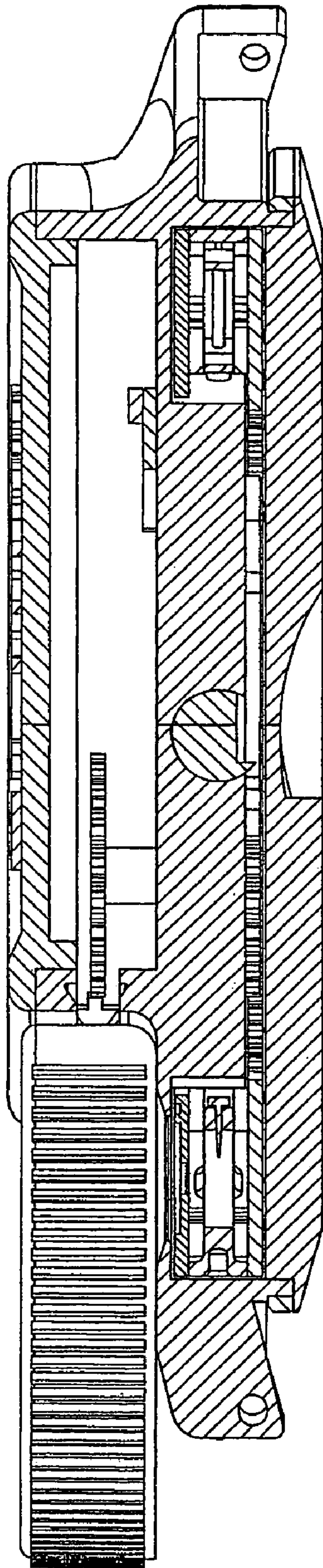
SECTION A-A
