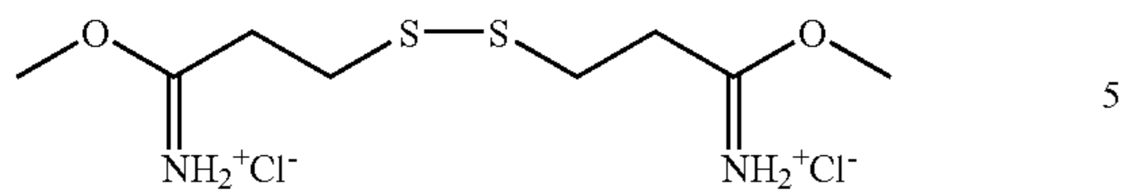
DTBP
