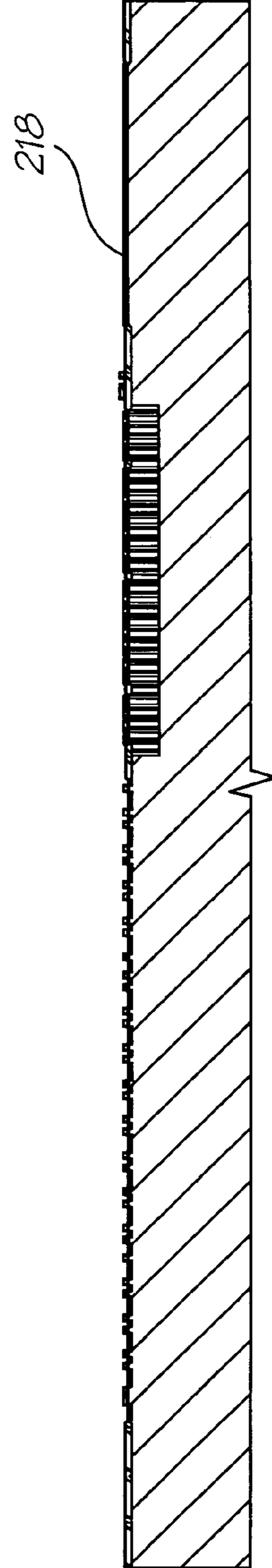
p+ implant
