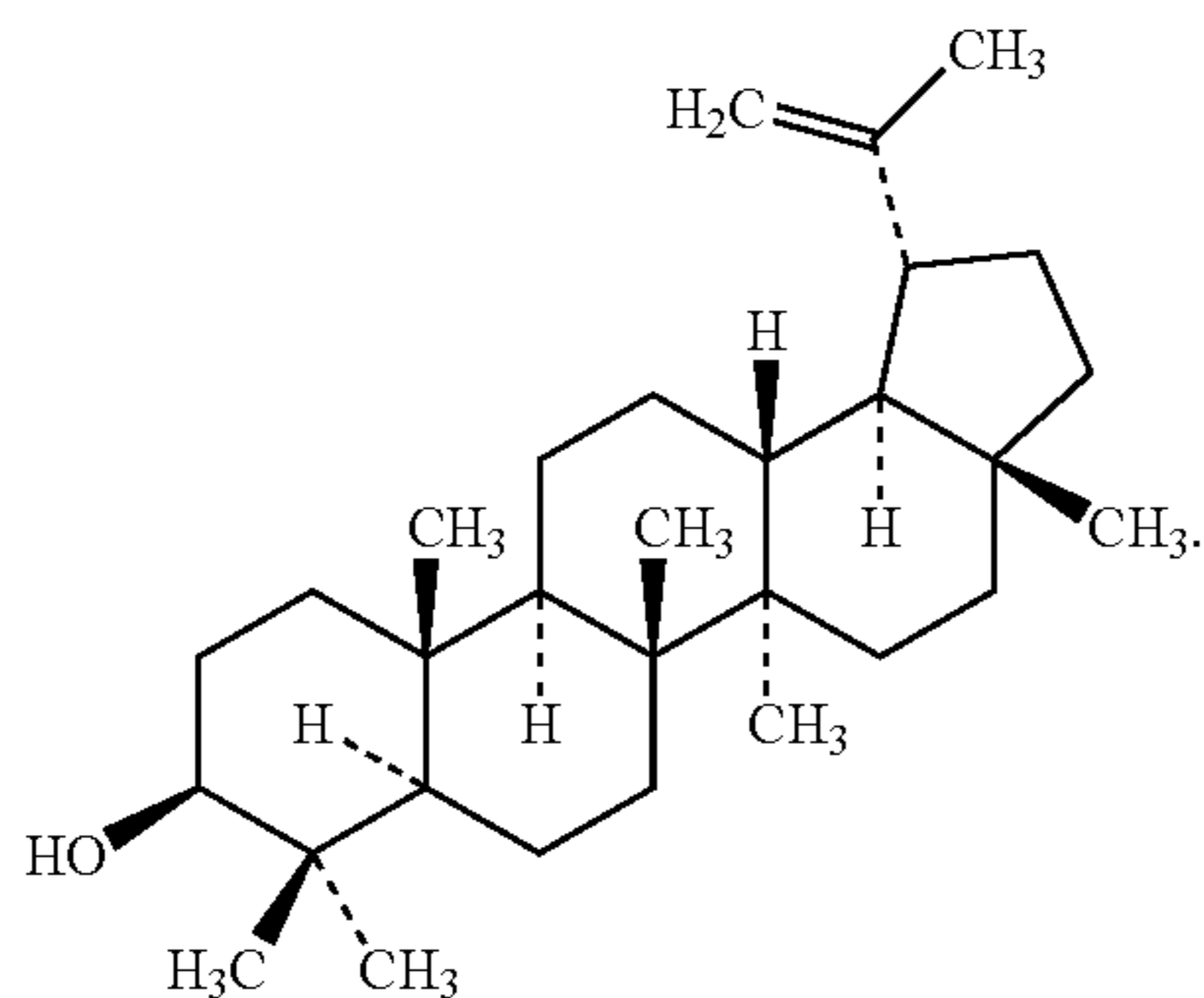
Lupeol
