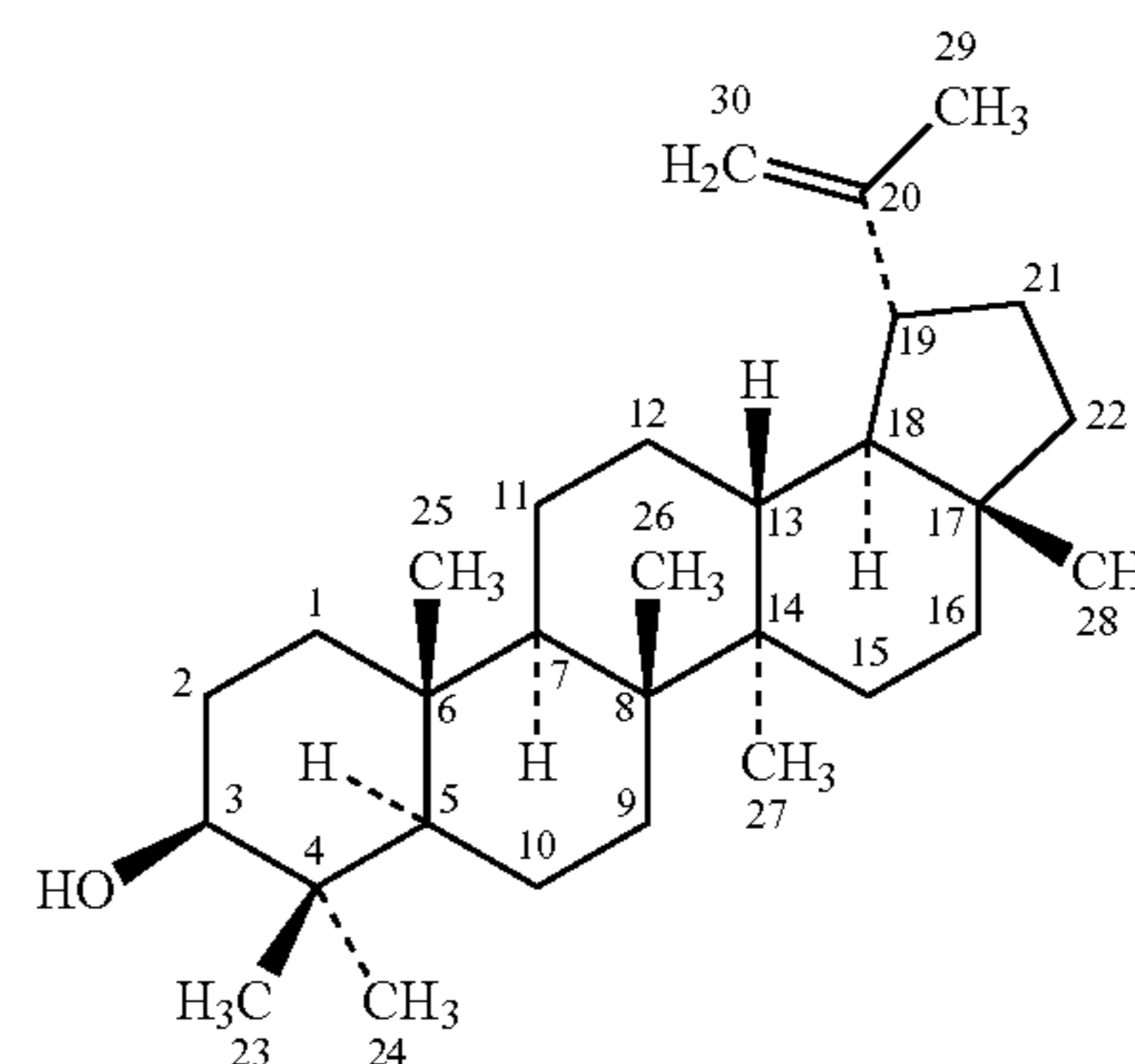
Lupeol
