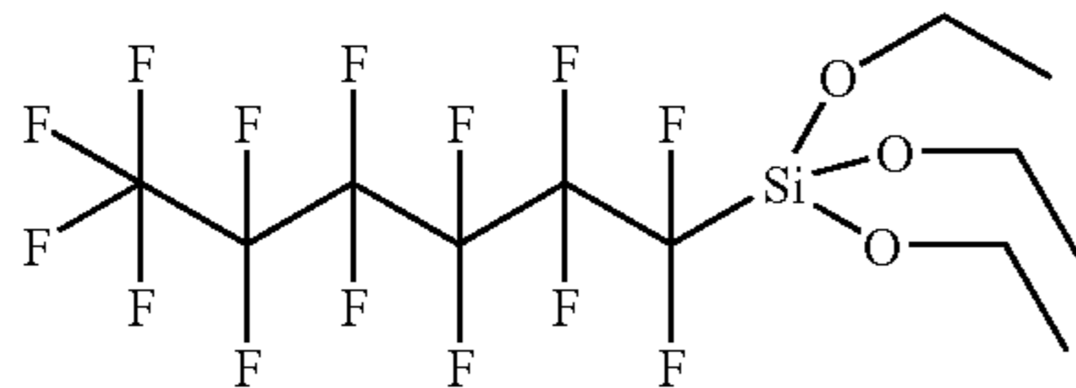
Perfluorohexanetriethoxysilane
