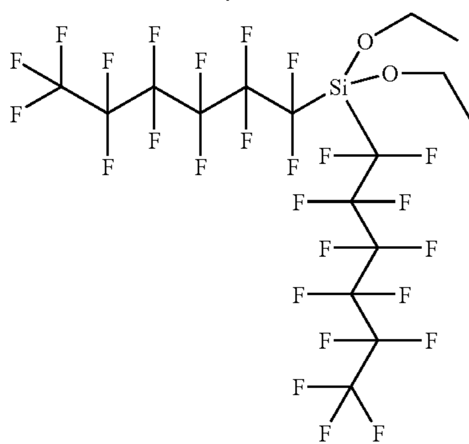
Bis(perfluorohexane)diethoxysilane
