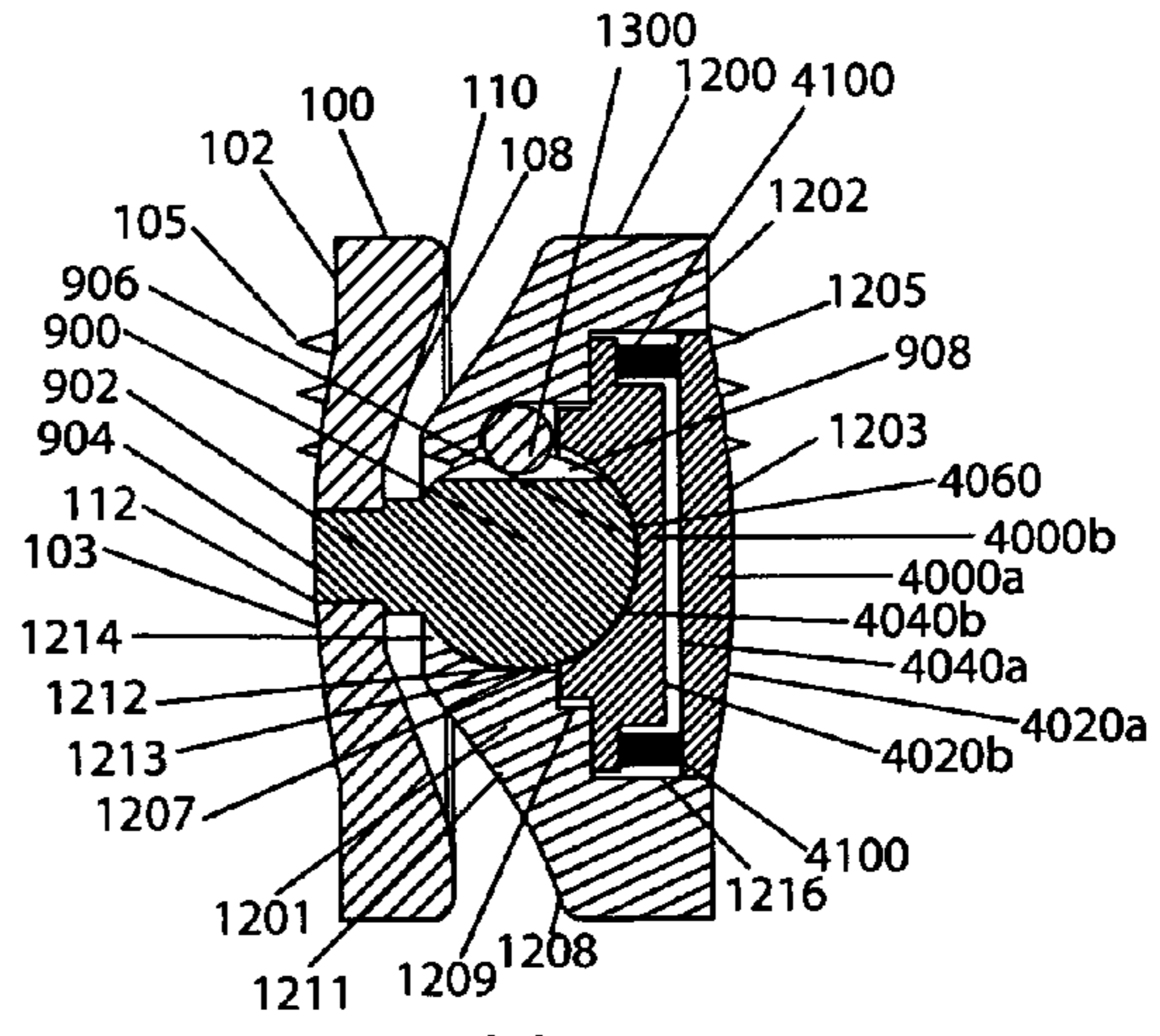
A-A FIG. 7k
