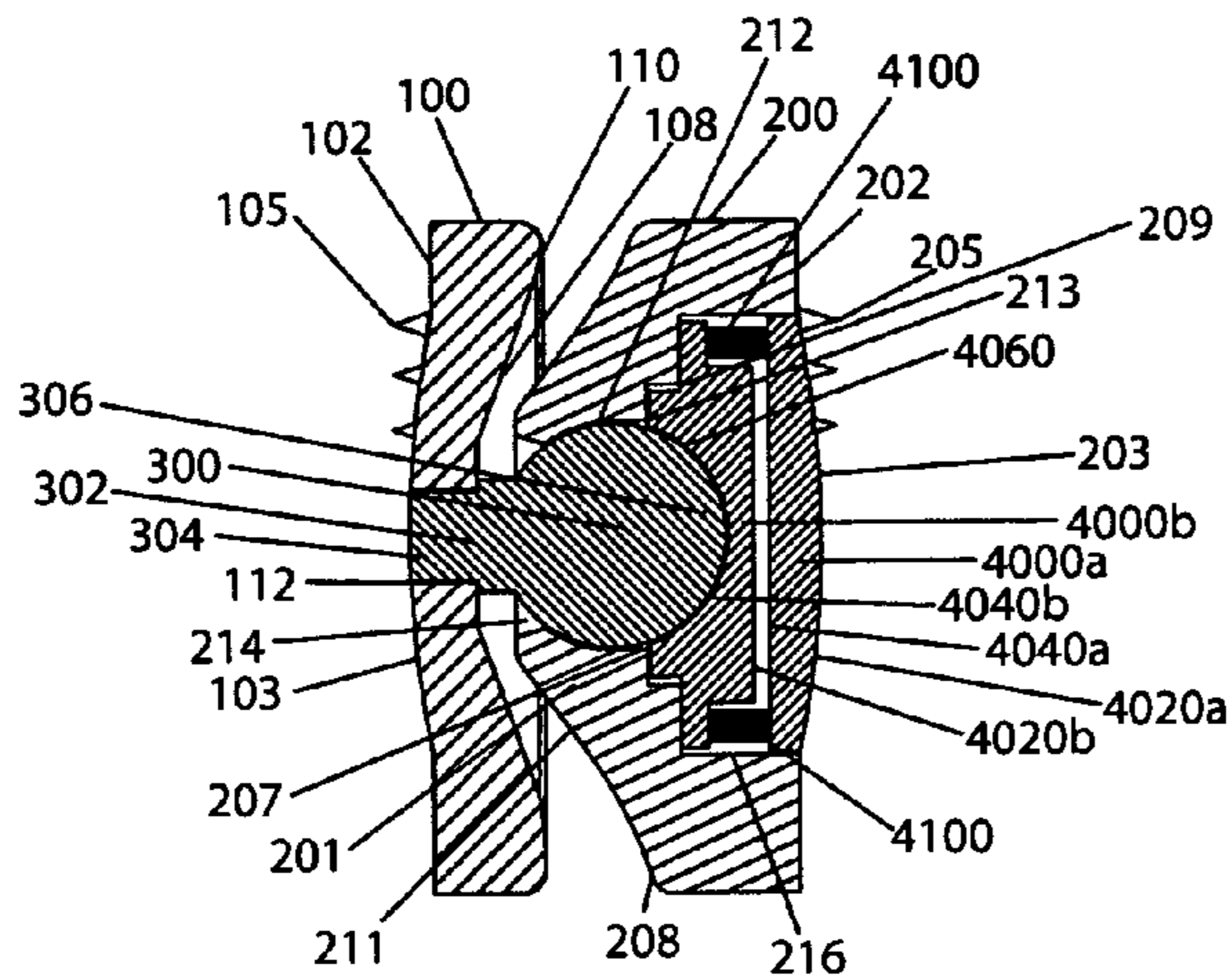
A-A FIG. 3z
