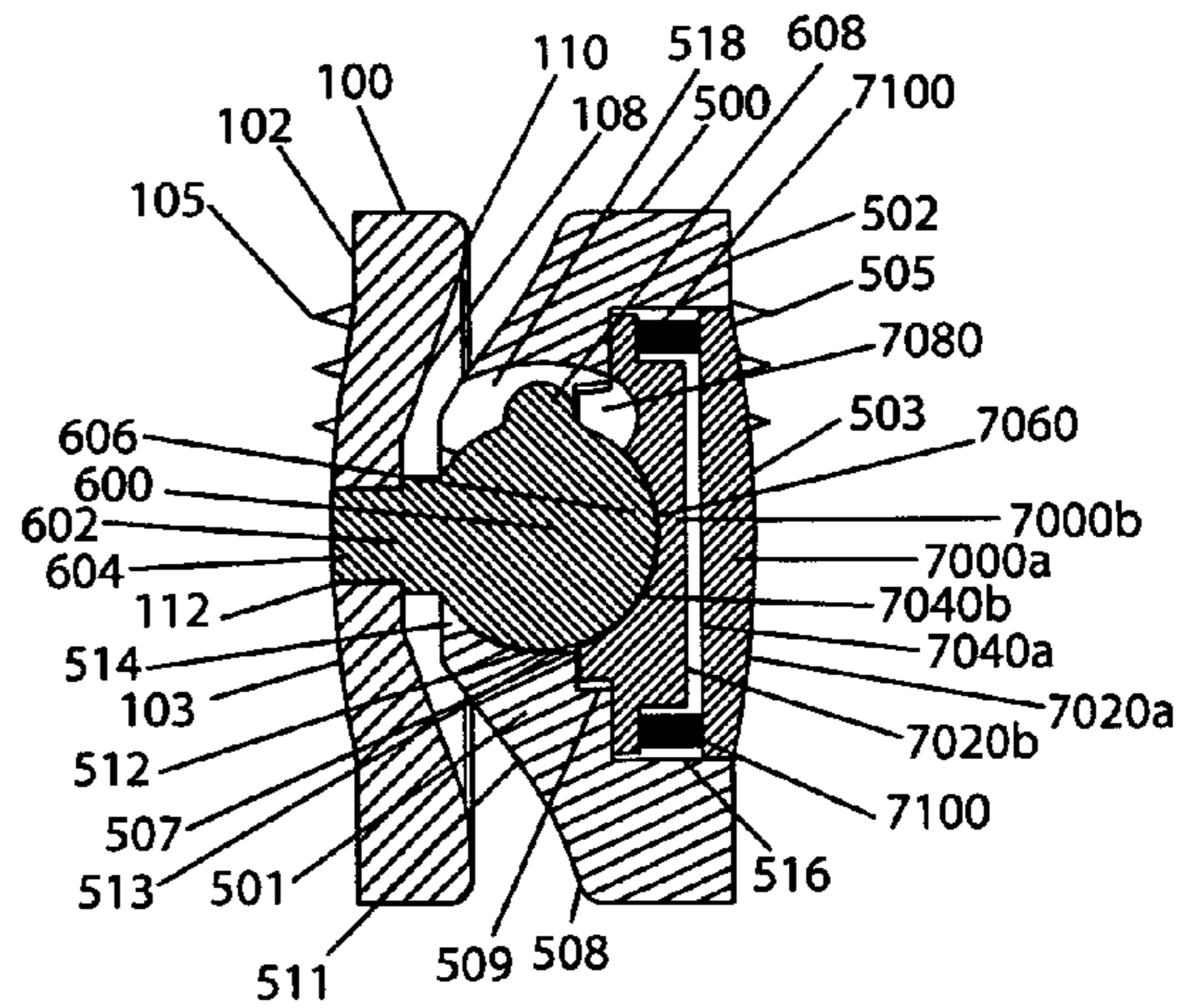
A-A FIG. 4u
