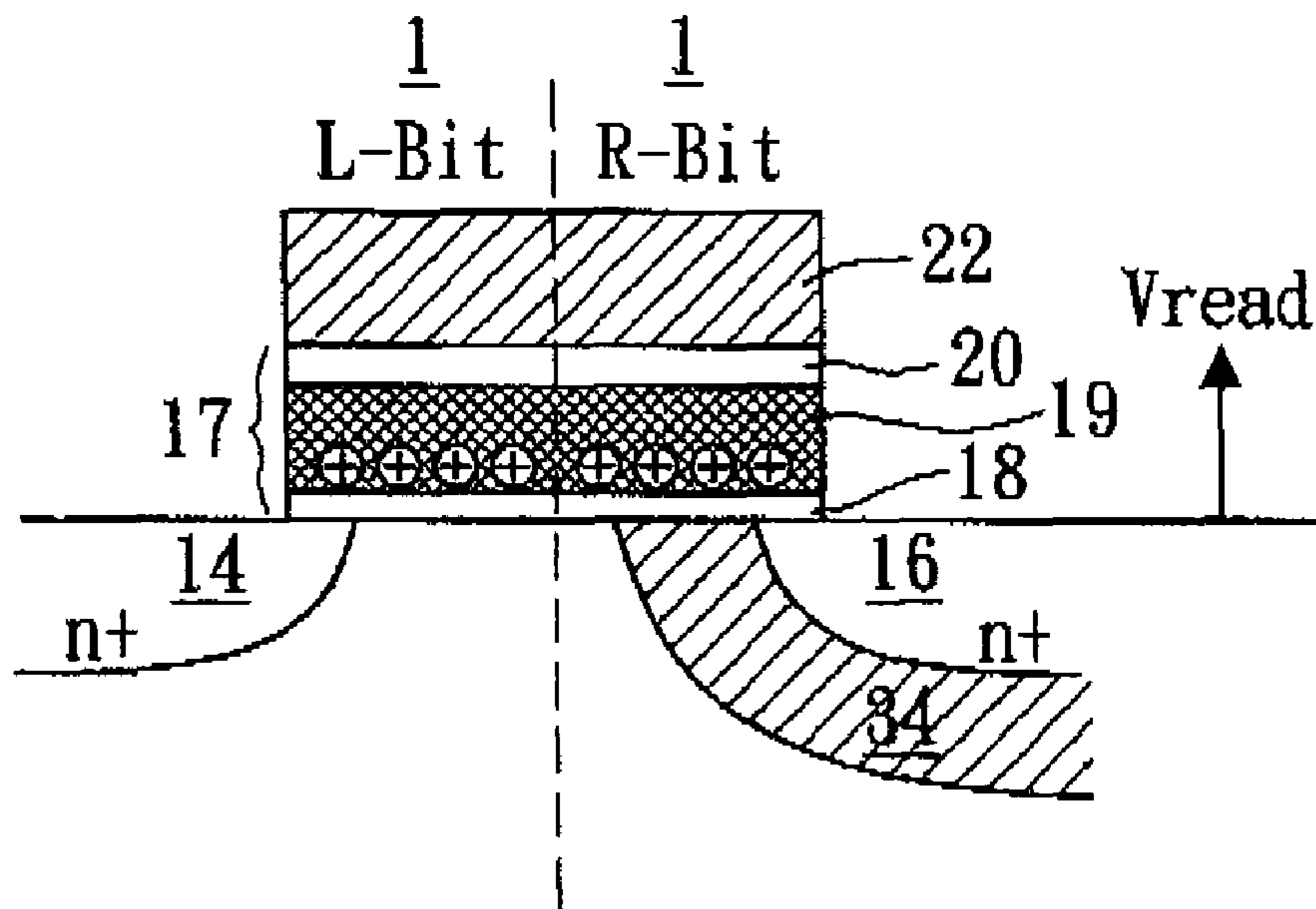
FIG. 3H(PRIOR ART)
