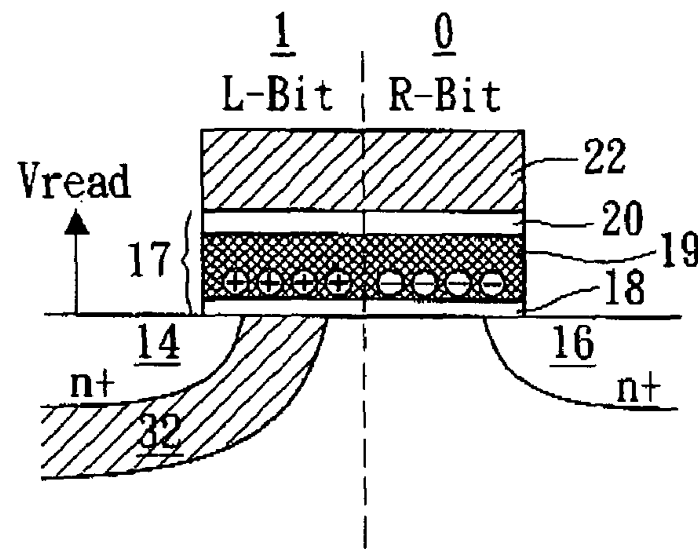
FIG. 3B(PRIOR ART)
