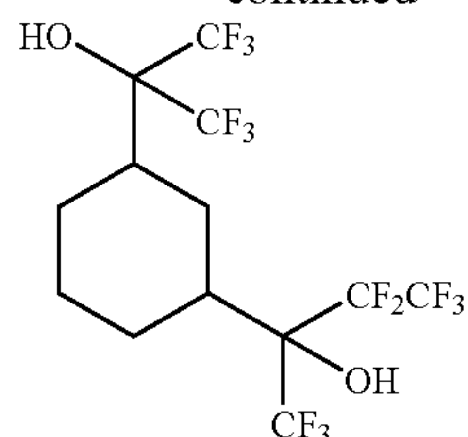
1,1,1,3,3,4,4,4-octafluoro-2-(3-[2,2,2-trifluoro-1-hydroxy-1-(trifluoromethyl)ethyl]cyclohexyl)butan-2-ol
