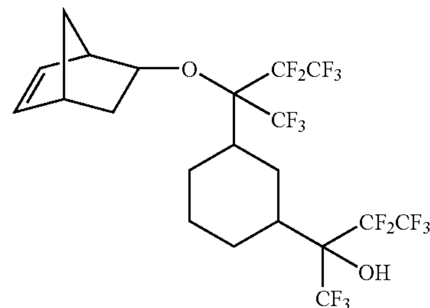
2-{3-[1-bicyclo[2.2.1]hept-5-en-2-yloxy-2,2,3,3,3-pentafluoro-1-(trifluoromethyl)propyl]cyclohexyl}-1,1,1,3,3,4,4,4-octafluorobutan-2-ol
