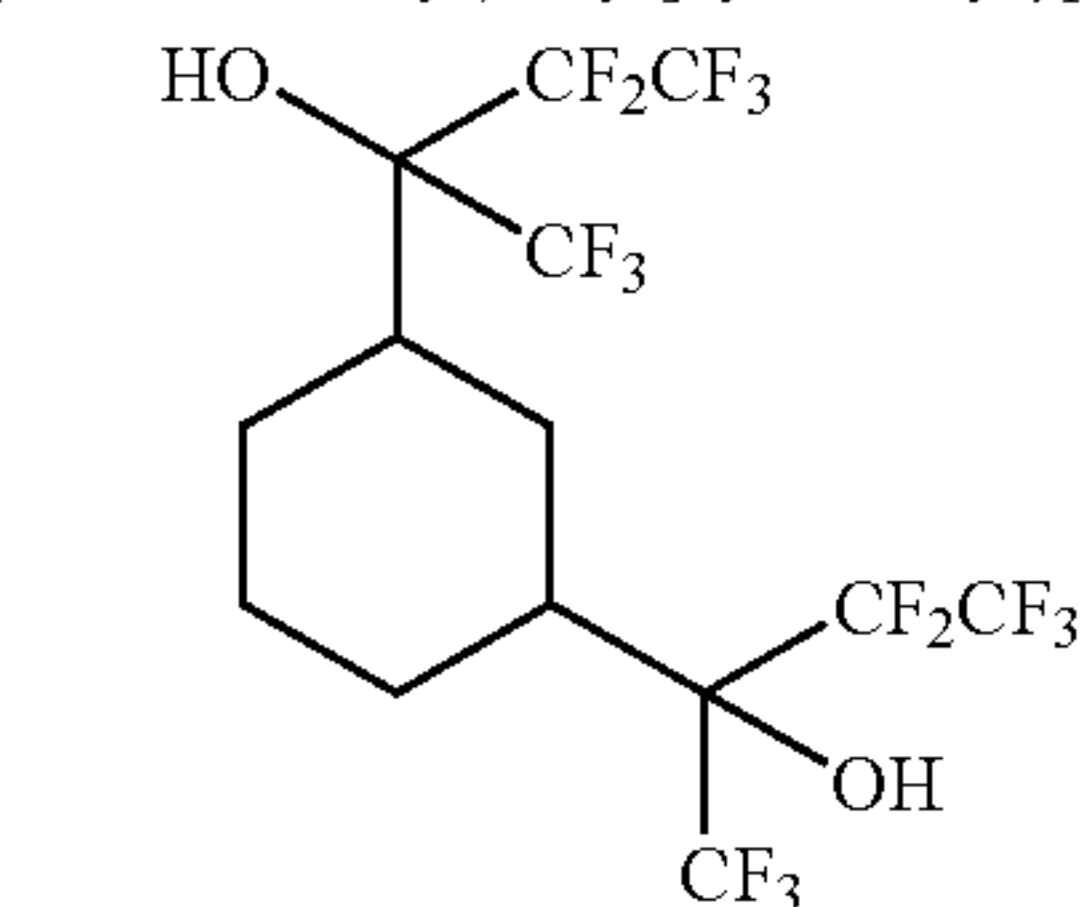
1,1,1,3,3,3,4,4,4-octafluoro-2-(3-[2,2,3,3,3-pentafluoro-1-hydroxy-1-(trifluoromethyl)propyl]cyclohexyl)butan-2-ol
