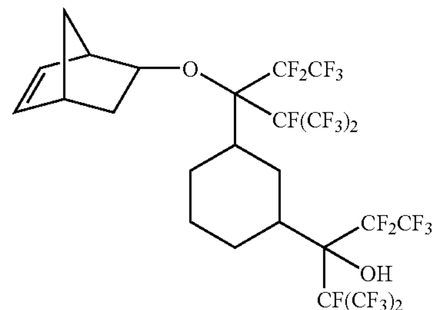
2-{3-[1-bicyclo[2.2.1]hept-5-en-2-yloxy-2,2,2-trifluoro-1-(trifluoromethyl)ethyl]cyclohexyl}-1,1,1,3,3,4,4,4-octafluorobutan-2-ol
