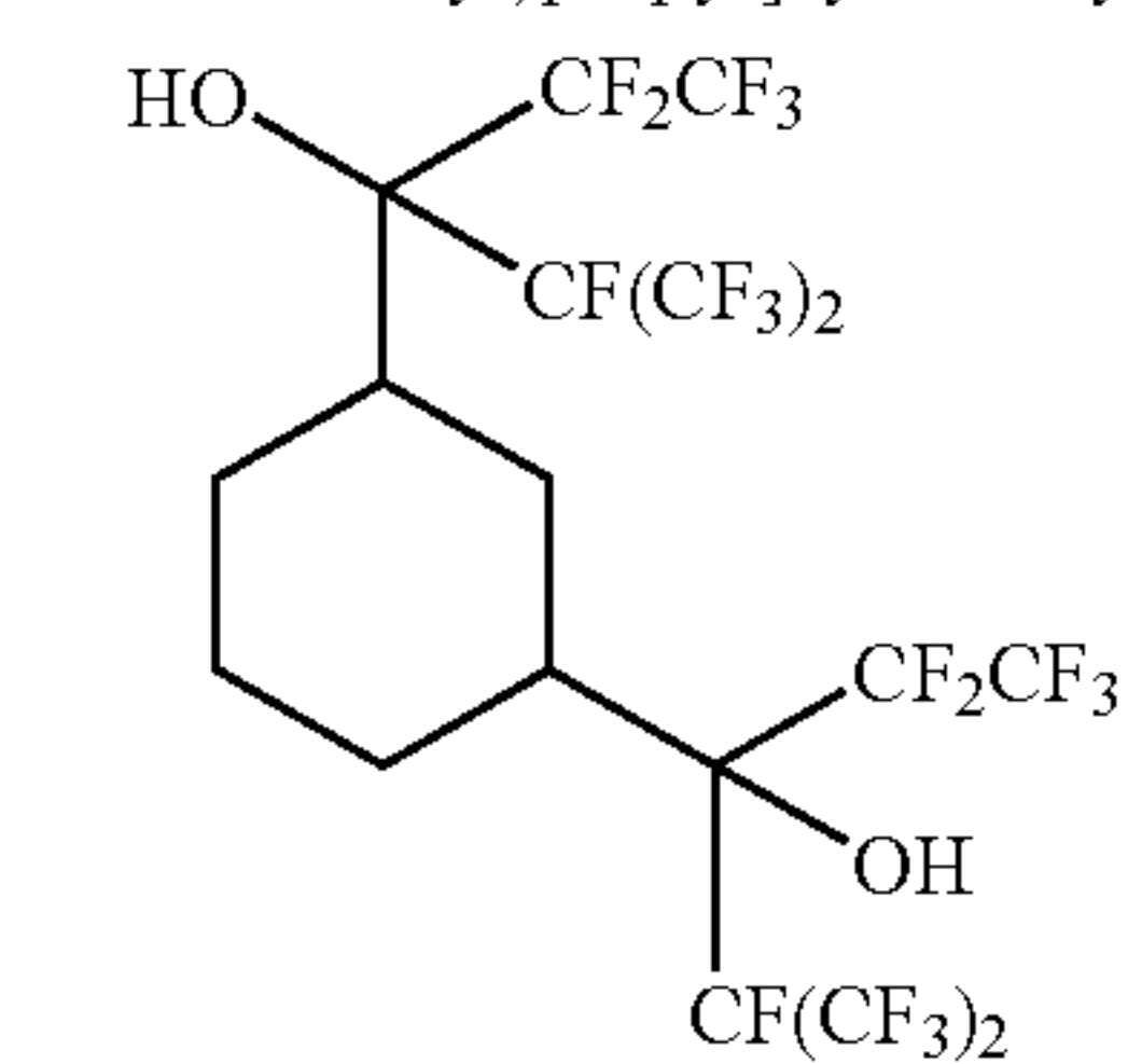
1,1,1,2,4,4,5,5,5-nonafluoro-3-(3-{2,2,3,3,3-pentafluoro-1-hydroxy-1-[1,2,2,2-tetrafluoro-(trifluoromethyl)ethyl]propyl}cyclohexyl)-2-(trifluoromethyl)pentan-3-ol
