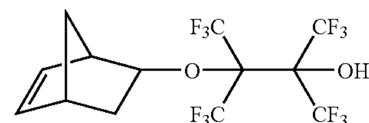
3-bicyclo[2.2.1]hept-5-en-2-yloxy-2,3-bis(trifluoromethyl)-1,1,4,4,4-hexafluorobutan-2-ol
