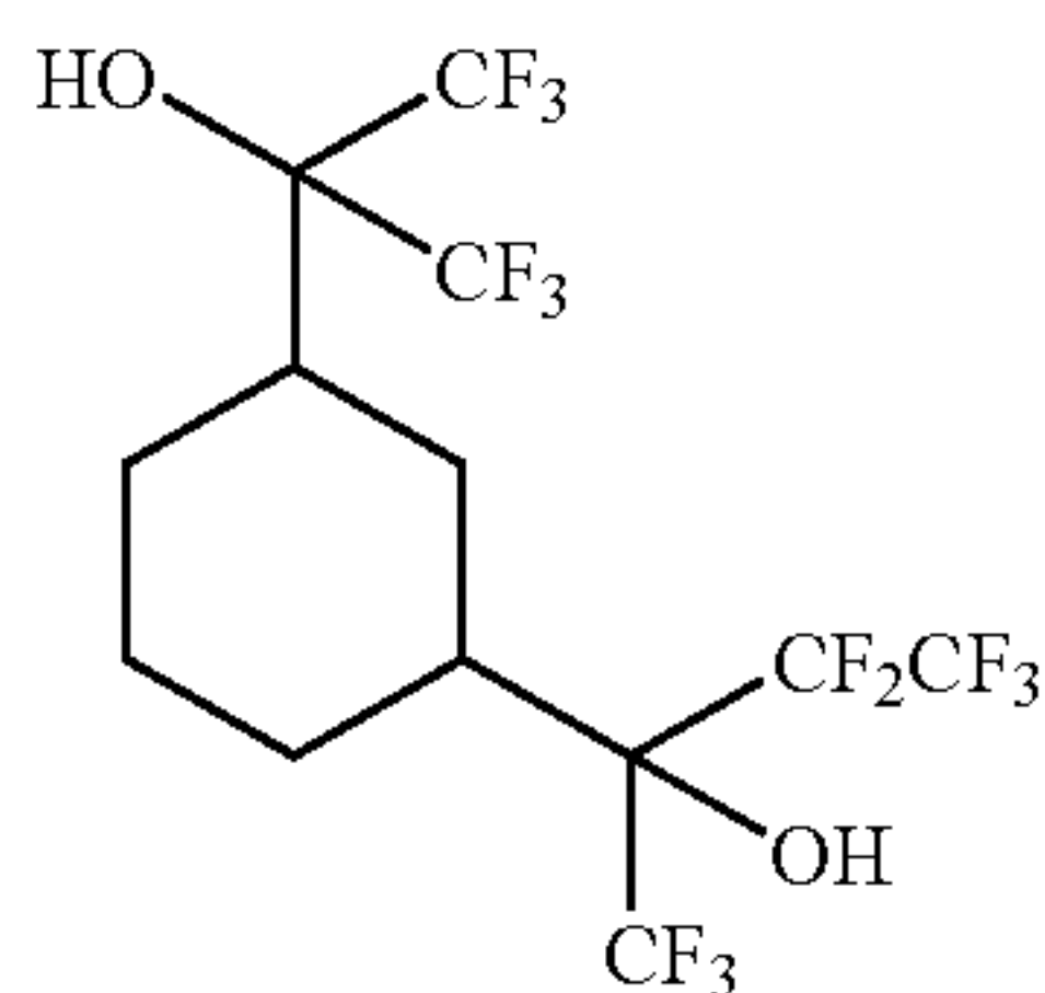
1,1,1,3,3,4,4,4-octafluoro-2-{3-[2,2,2-trifluoro-1-hydroxy-1-(trifluoromethyl)ethyl]cyclohexyl}butan-2-ol
