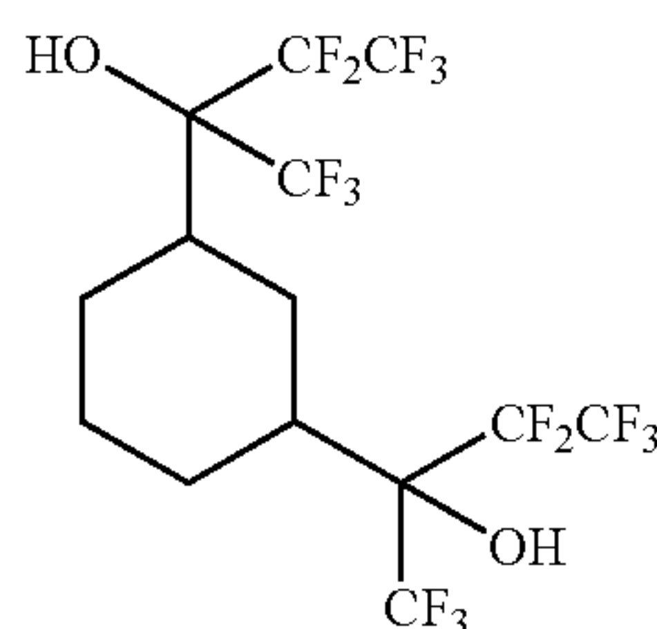
1,1,1,3,3,4,4,4-octafluoro-2-{3-[2,2,3,3,3-pentafluoro-1-hydroxy-1-(trifluoromethyl)propyl]cyclohexyl}butan-2-ol
