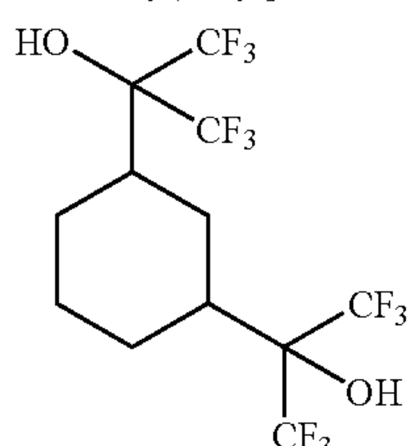
1,1,1,3,3,4,4,4-hexafluoro-2-{3-[2,2,2-trifluoro-1-hydroxy-1-(trifluoromethyl)ethyl]cyclohexyl}propan-2-ol
