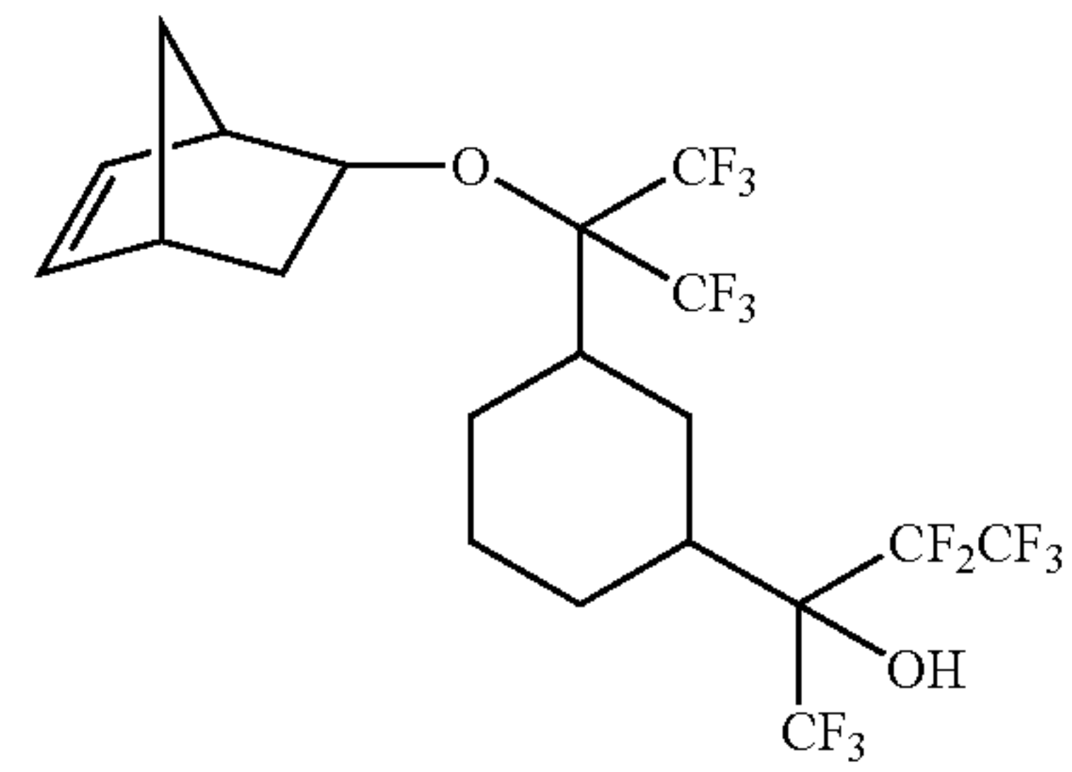
2-{3-[1-bicyclo[2.2.1]hept-5-en-2-yloxy-2,2,2-trifluoro-1-(trifluoromethyl)ethyl]cyclohexyl}-1,1,1,3,3,4,4,4-octafluorobutan-2-ol
