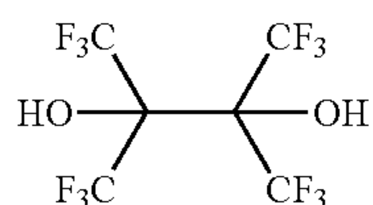
2,3-bis(trifluoromethyl)-1,1,1,4,4,4-hexafluorobutane-2,3-diol
