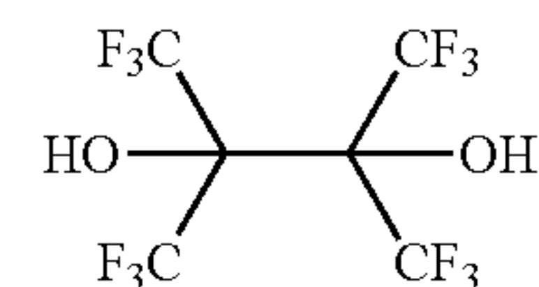
2,3-bis(trifluoromethyl)-1,1,1,4,4,4-hexafluorobutane-2,3-diol
