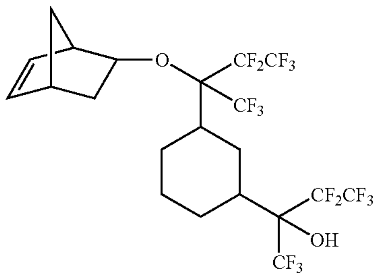
2-{3-[1-bicyclo[2.2.1]hept-5-en-2-yloxy-2,2,3,3,3-pentafluoro-1-(trifluoromethyl)propyl]cyclohexyl}-1,1,1,3,3,4,4,4-octafluorobutan-2-ol
