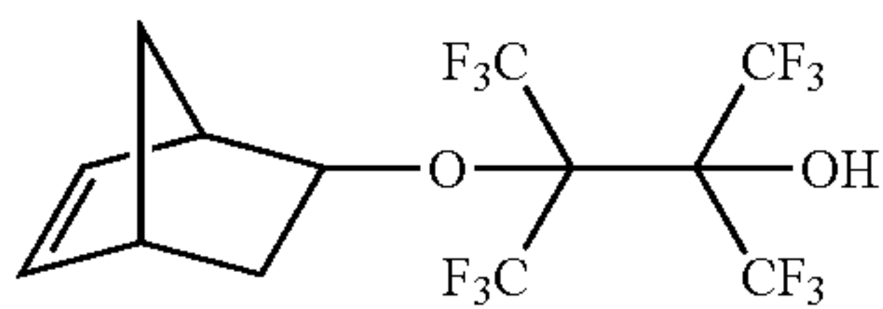
3-bicyclo[2.2.1]hept-5-en-2-yloxy-2,3-bis(trifluoromethyl)-1,1,1,4,4,4-hexafluorobutan-2-ol
