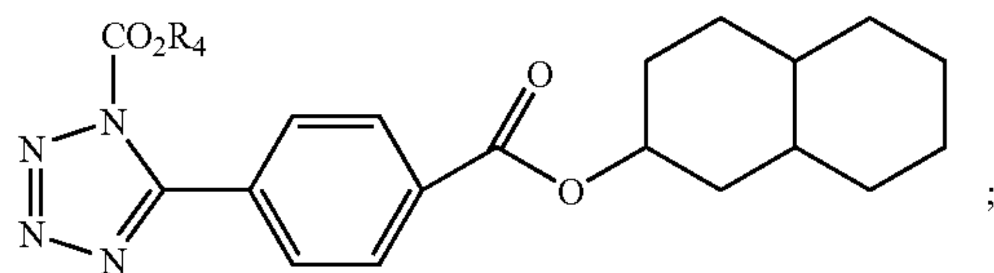
Formula BU
