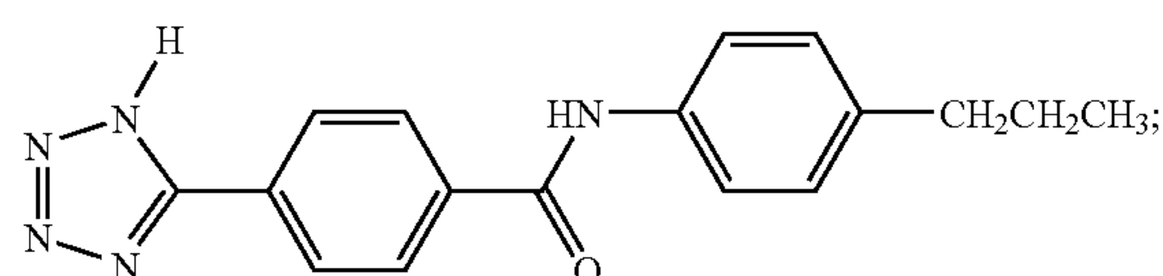
Compound EI
