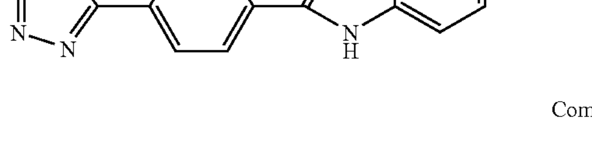
Compound IK
