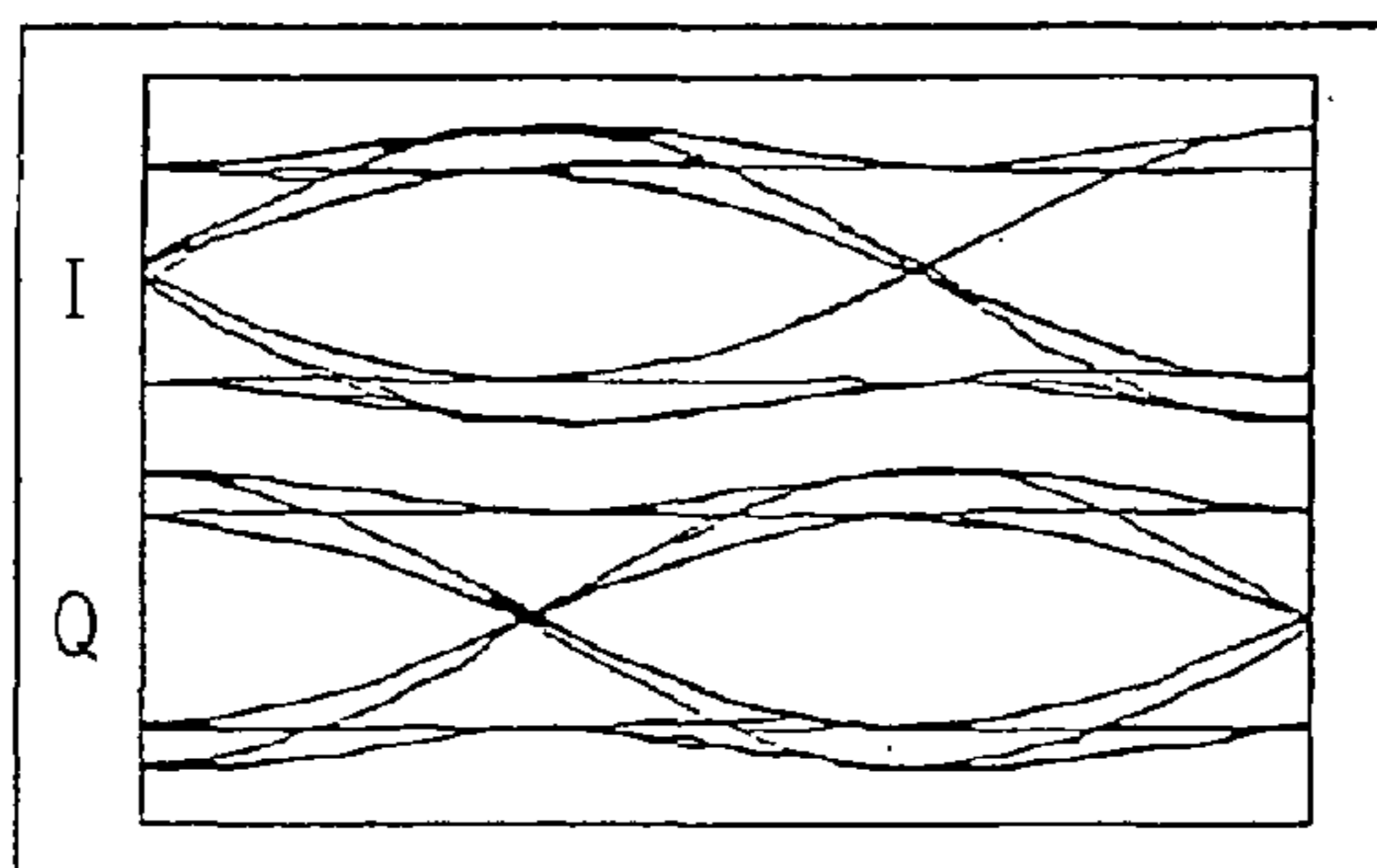
FQPSK-B MEAS.
