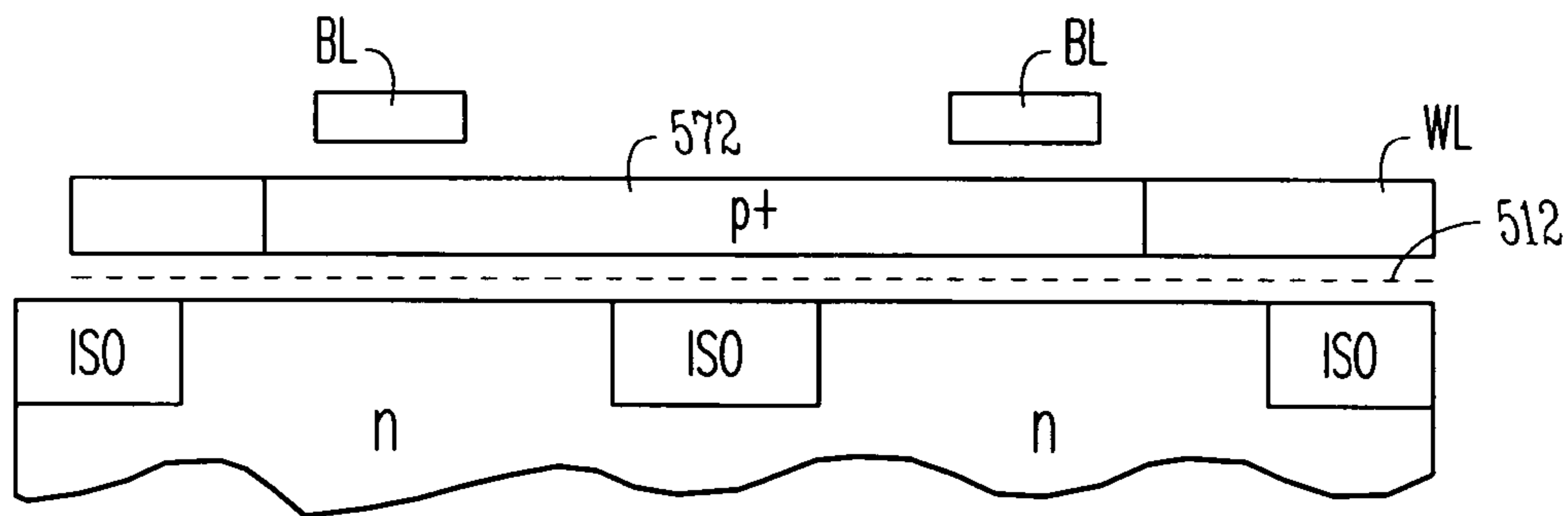
Fig. 5D
