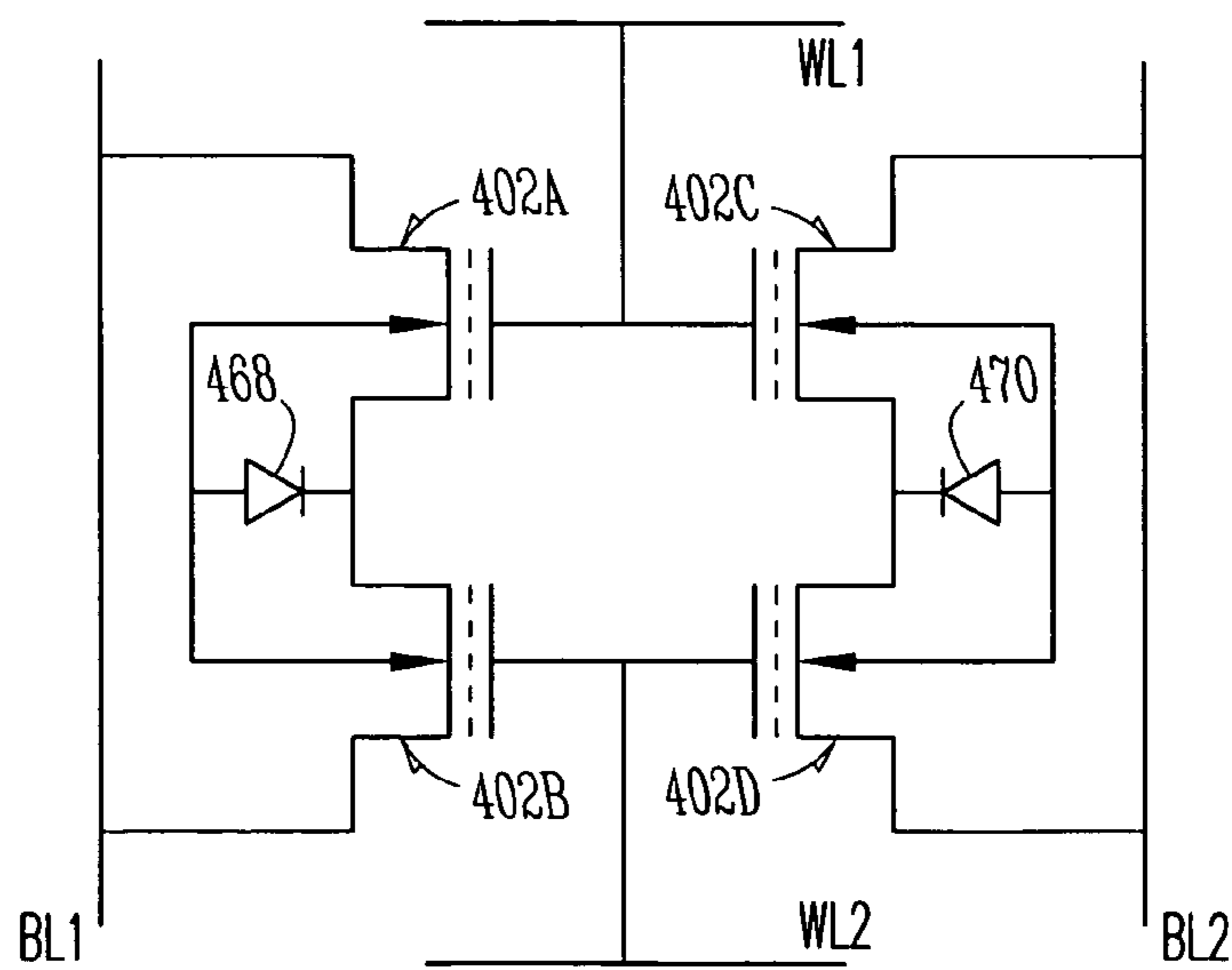
Fig. 4E
