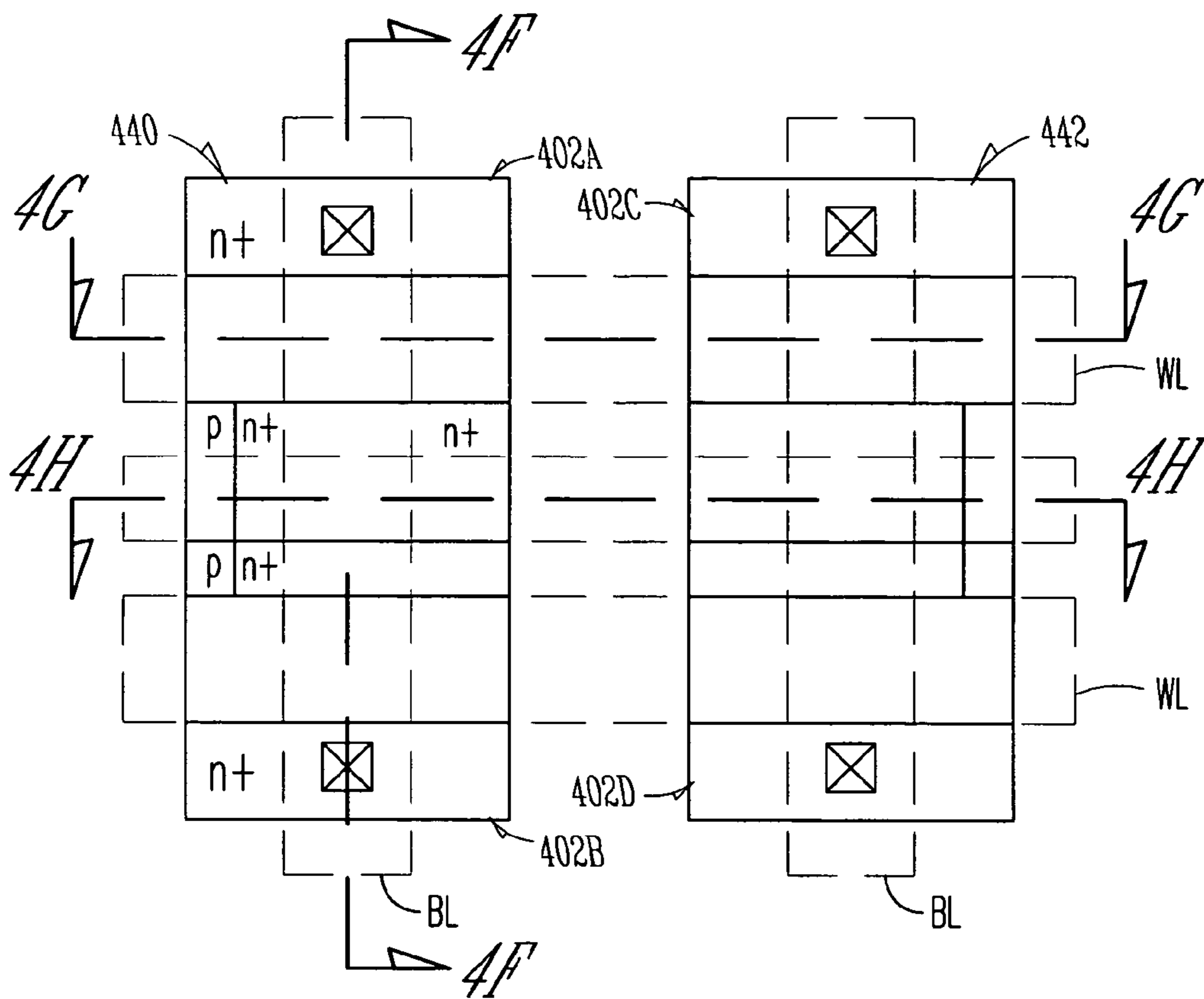
Fig. 4D
