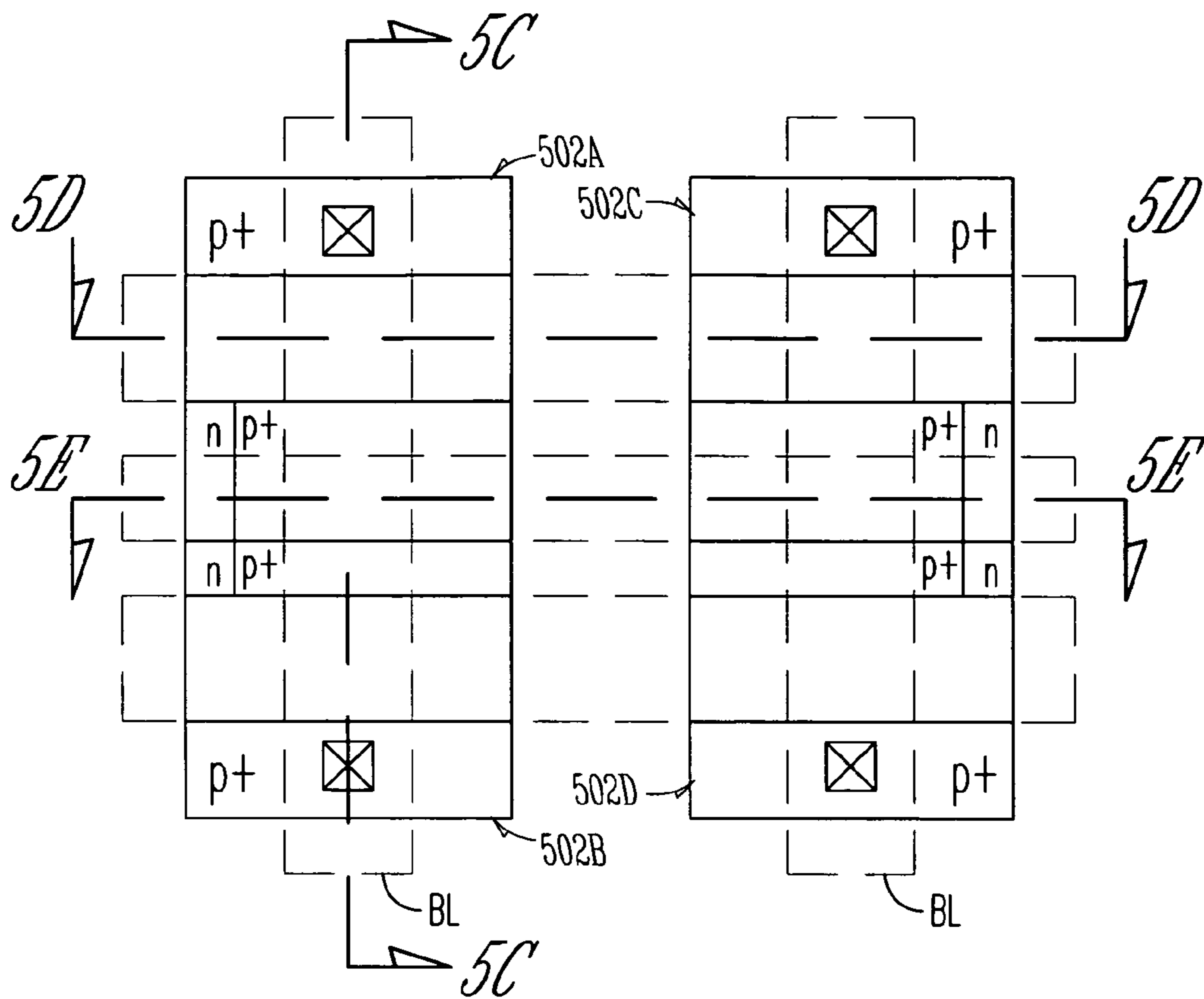
Fig. 5A
