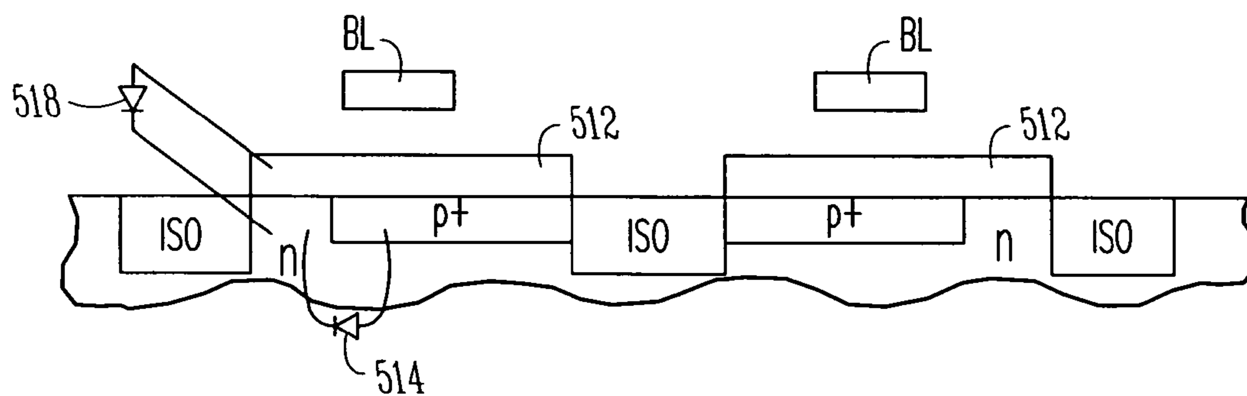
Fig. 5E
