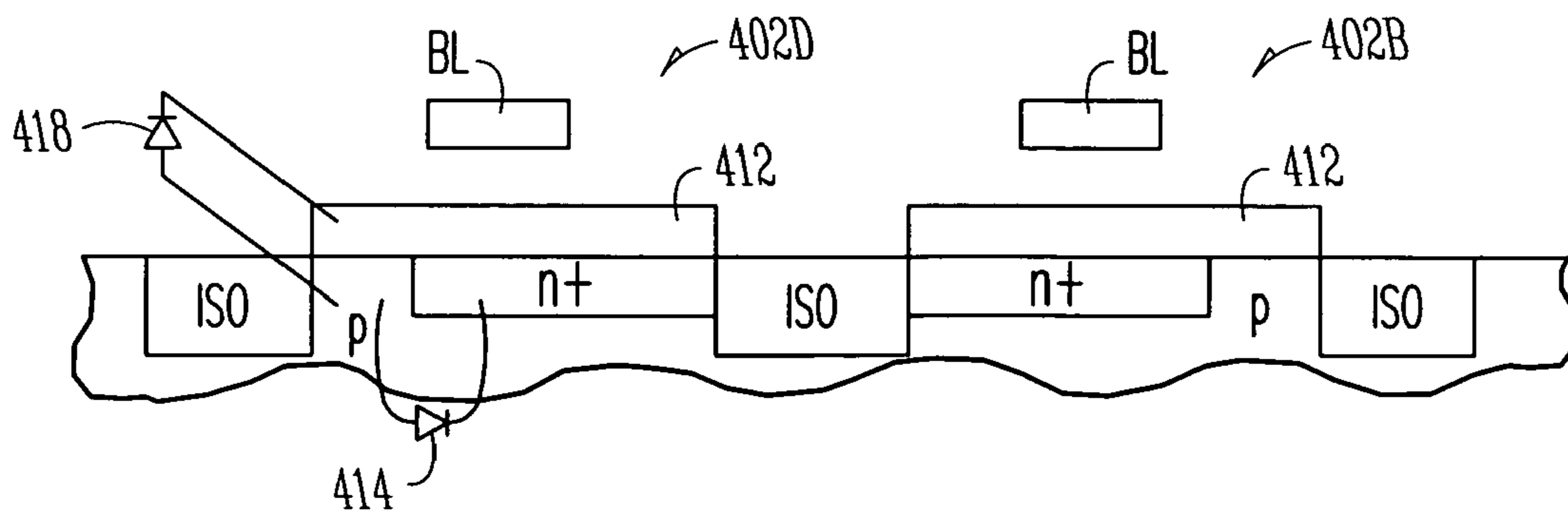
Fig. 4H
