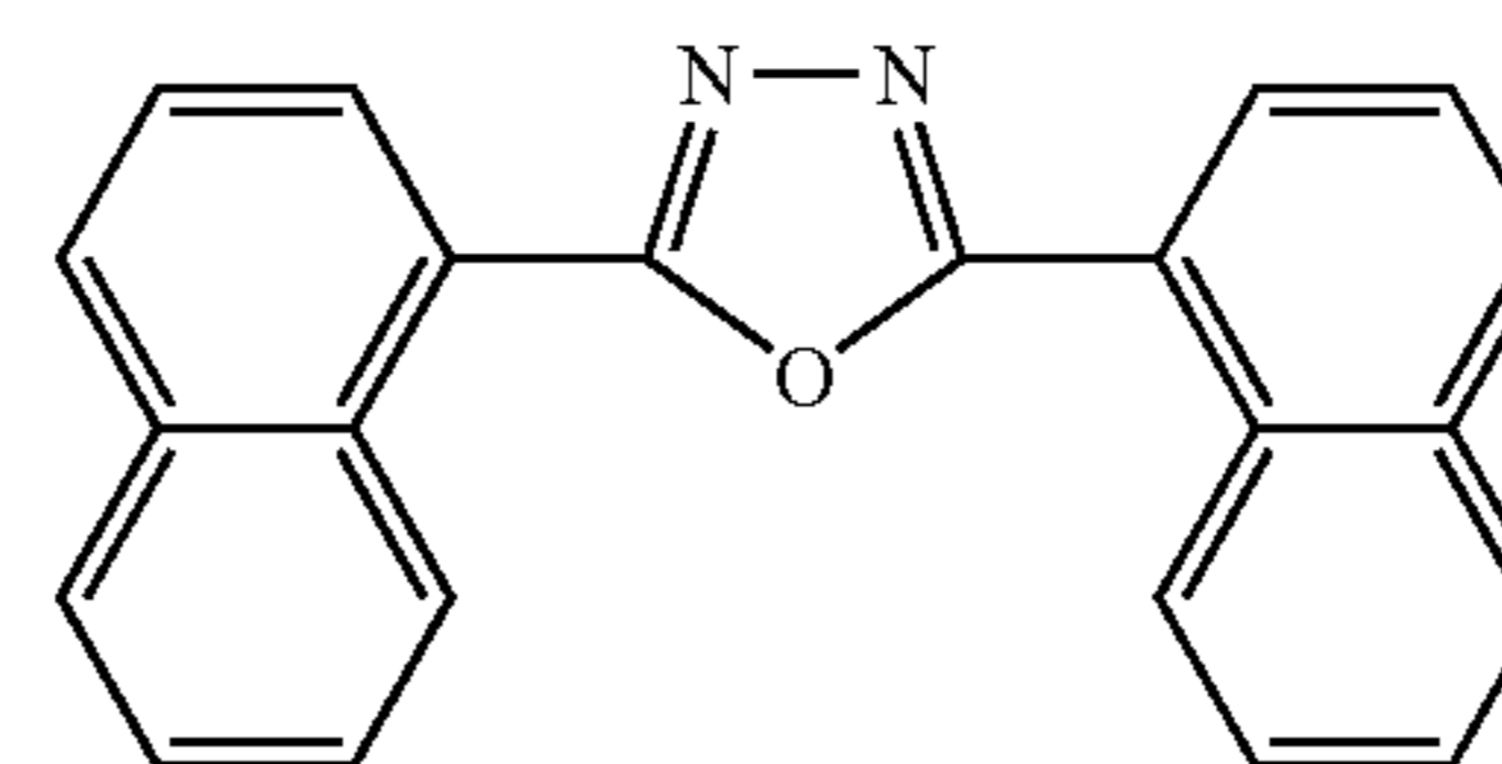
BND
