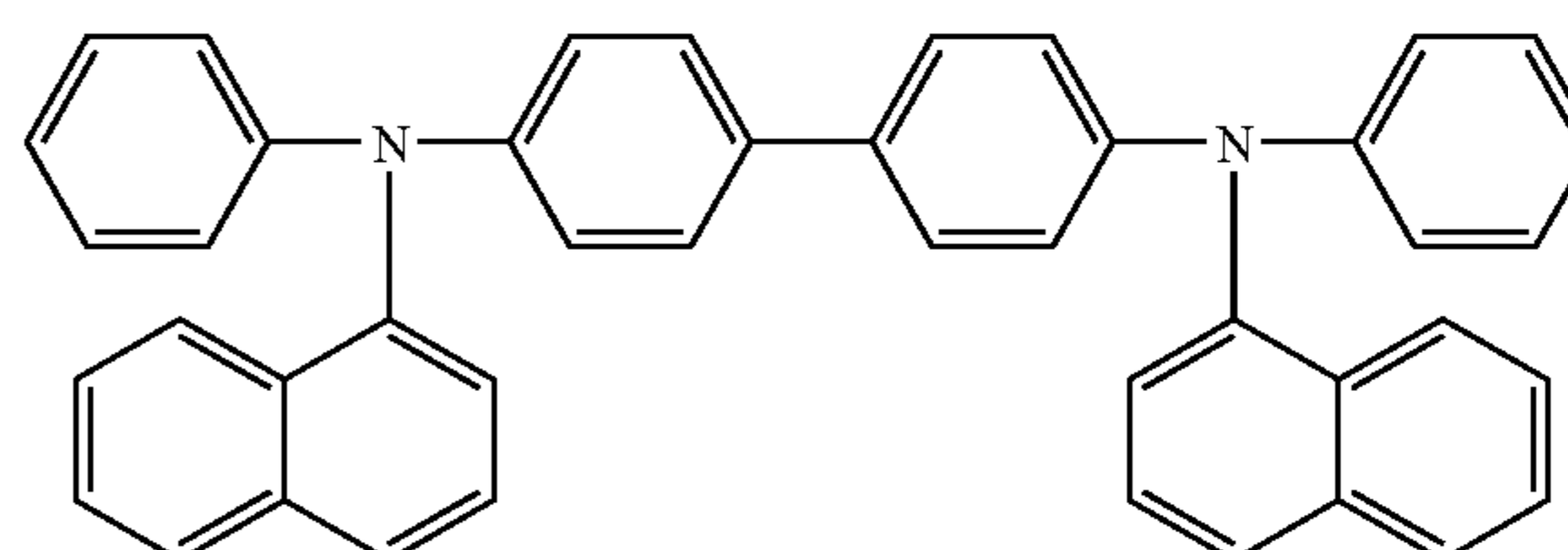
\alpha -NPD
