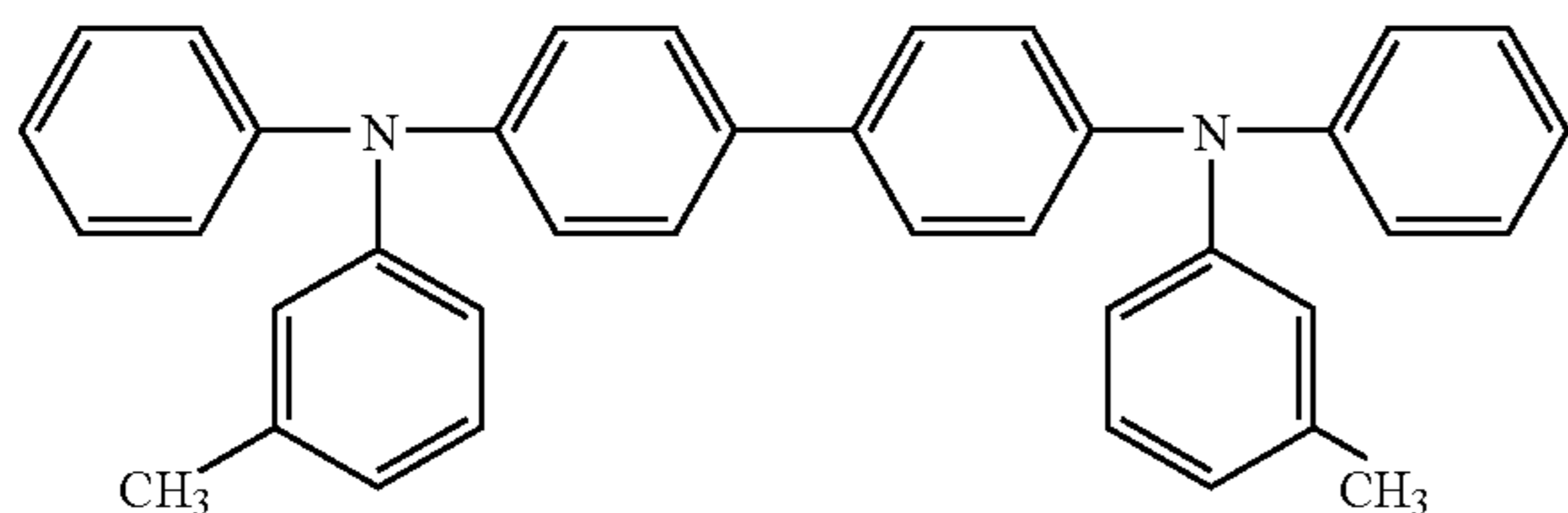
TPD
