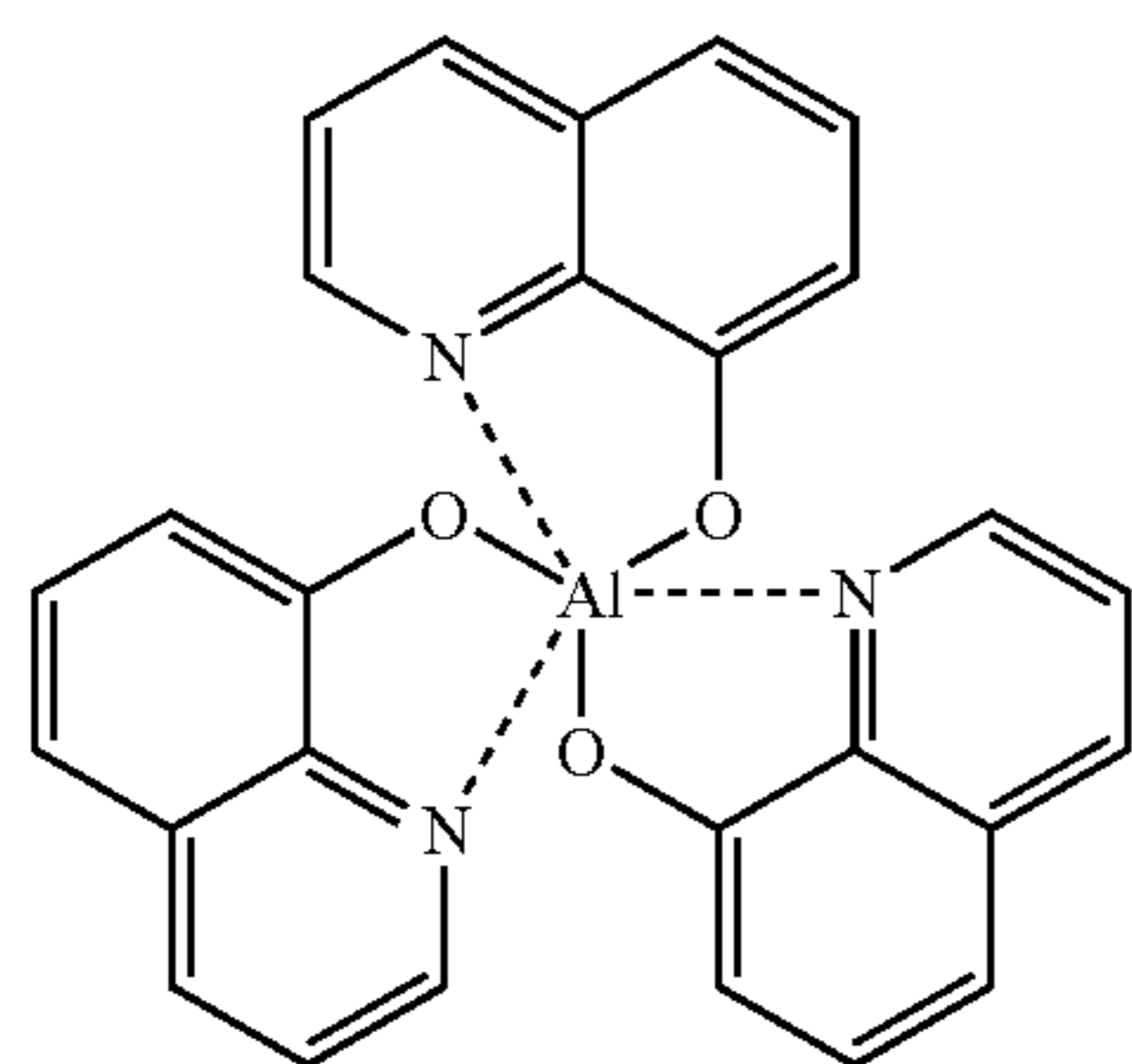
Alq3
